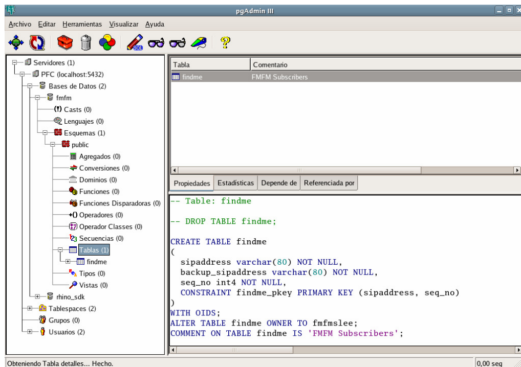
Figura 4.51: Base da datos fmfm vista desde el pgAdmin III.
