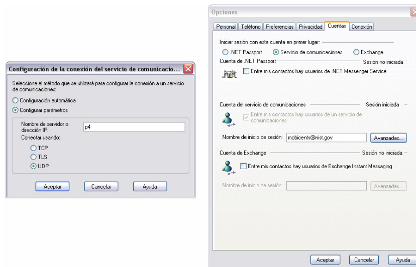
Figura 4.56: Configuración del cliente MSN.
