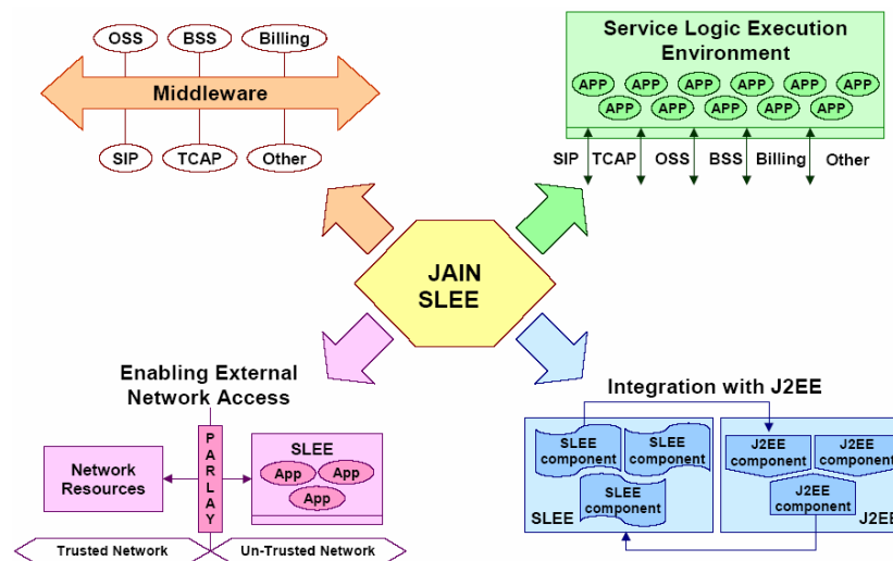
Figura 3.2: JAIN SLEE en un entorno de telecomunicaciones.
