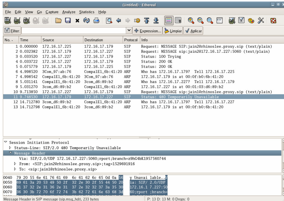
Figura 4.18: Ethereal durante el envío de mensajes instantáneos.
