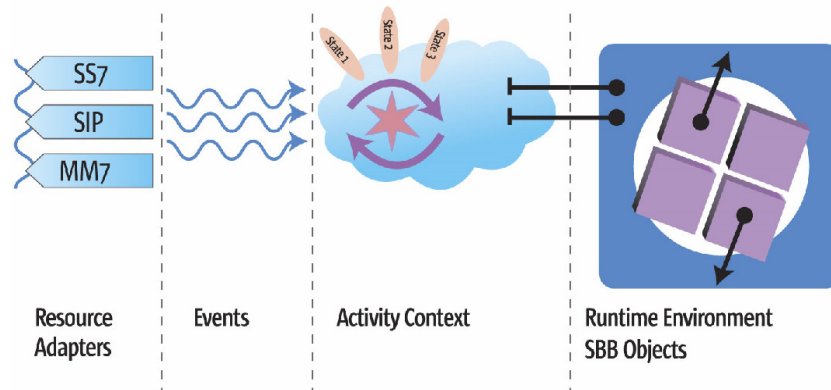
Figura 2.7: Los 4 elementos básicos del SLEE.
