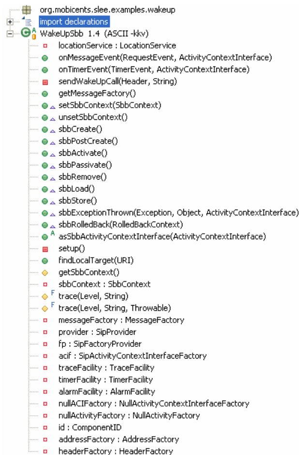
Figura 4.55: Listado del contenido del SBB.
