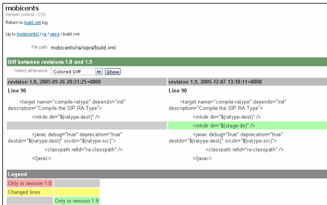
Figura 4.61: Diferencias con la versión anterior del fichero build.xml del SIP RA.
