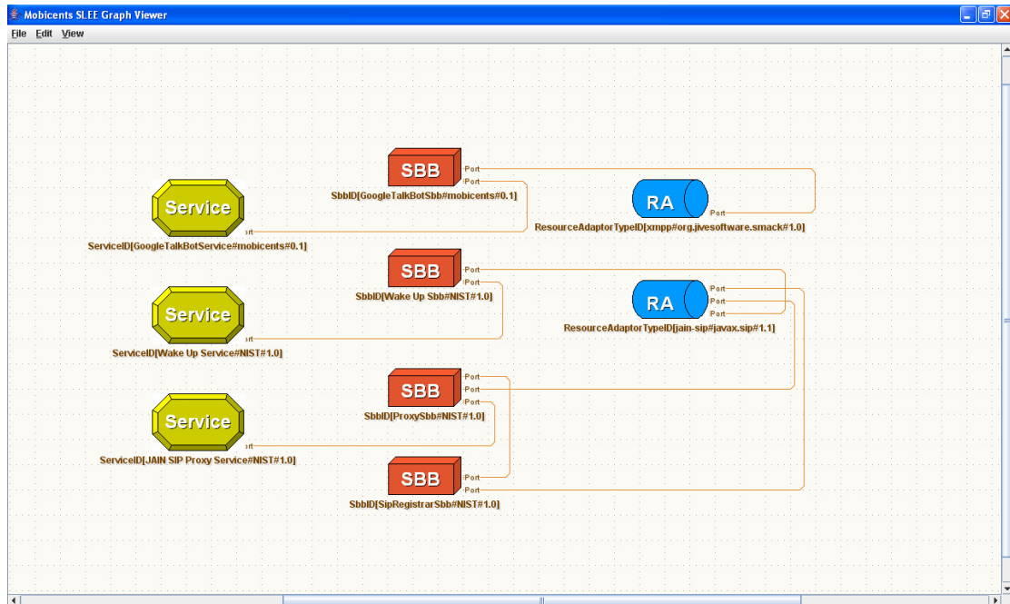
Figura 5.1: Aplicación Slee Graph Viewer .
