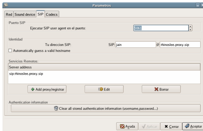
Figura 4.28: Cambio del puerto SIP en el cliente.
