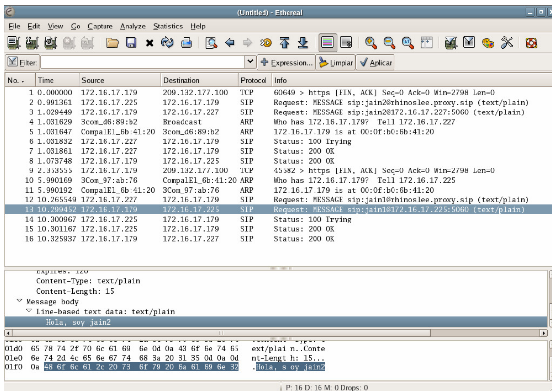
Figura 4.25: Ethereal durante el envío de mensajes instantáneos (solucionado el problema).
