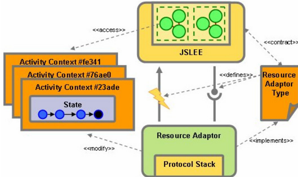
Figura 3.6: RA, RA Type, pila de protocolo, contexto de actividad y JSLEE.
