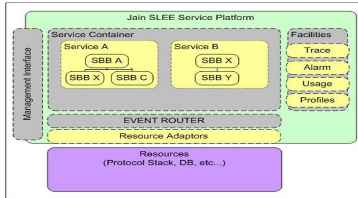
Figura 3.10: Arquitectura JSLEE simplificada 1.
