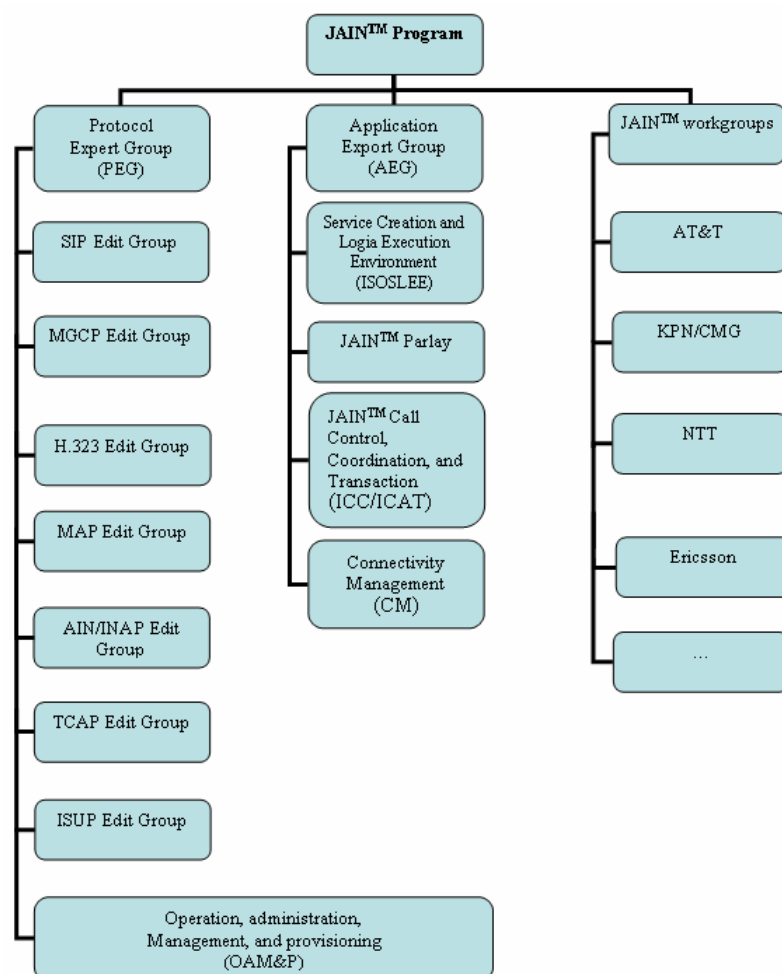
Figura 2.3: Organización de la comunidad JAIN.
