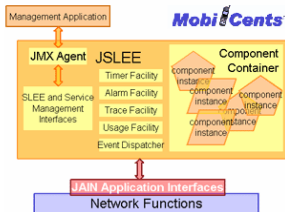
Figura 3.11: Arquitectura JSLEE simplificada 2.
