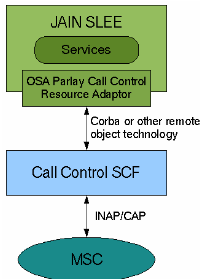
Figura 5.2: JAIN SLEE y OSA/Parlay.
