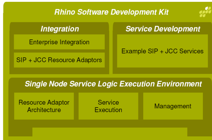
Figura 3.8: El Rhino SDK SLEE de Open Cloud.
