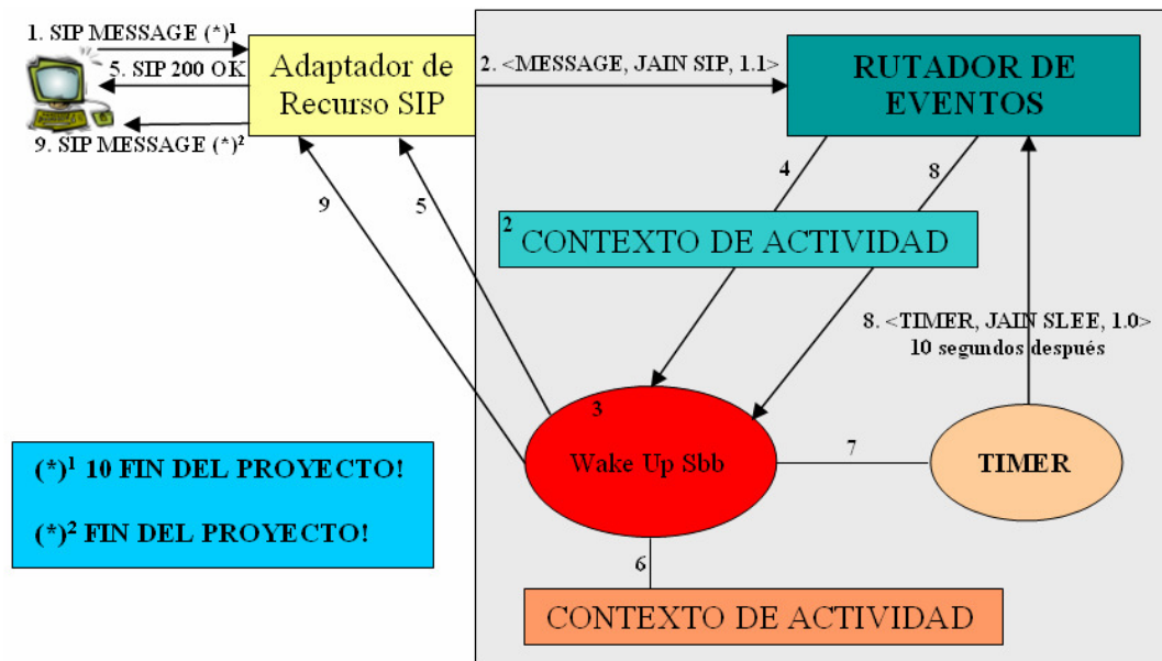
Figura 4.54: Pasos seguidos en el servicio Wake Up Call .
