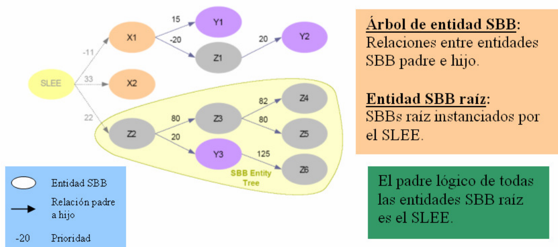
Figura 3.3: Árboles de entidad SBB.
