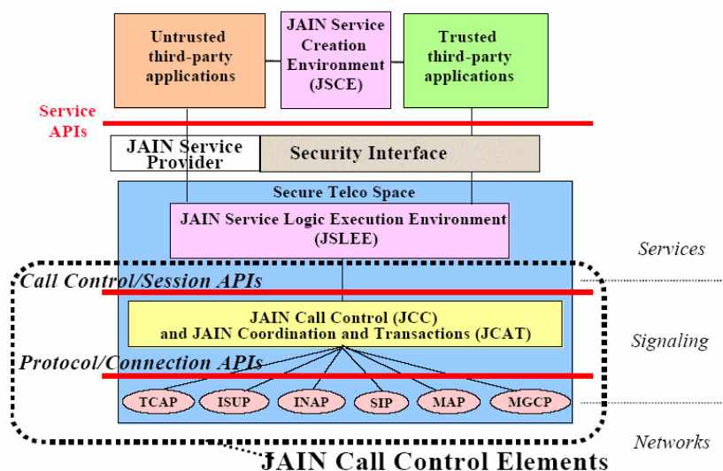
Figura 2.6: APIs de JAIN.
