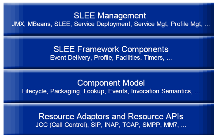
Figura 3.1: Capas de la arquitectura JSLEE.
