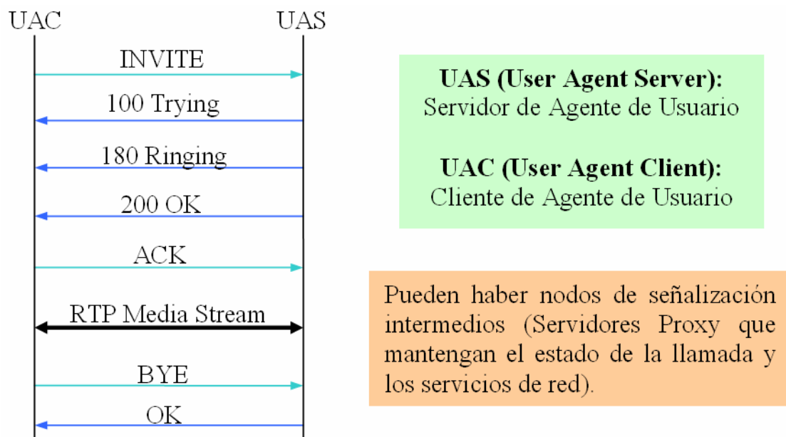
Figura 2.2: Ejemplo SIP de un flujo de llamada.
