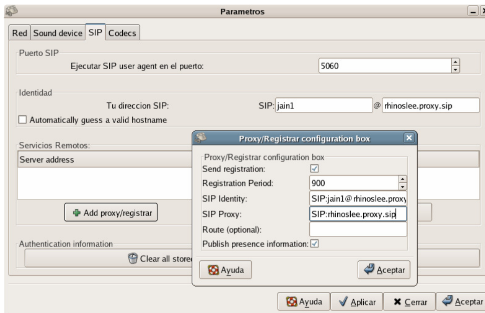
Figura 4.12: Configuración del Proxy/Registrar .
