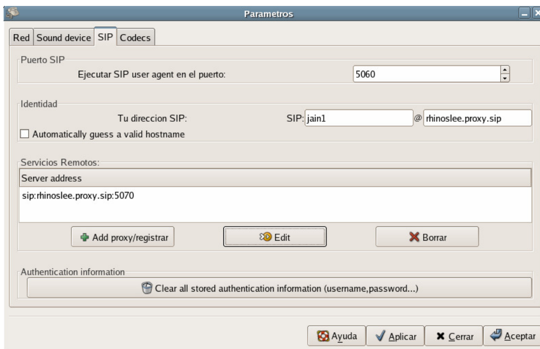
Figura 4.30: Nueva configuración del Linphone.
