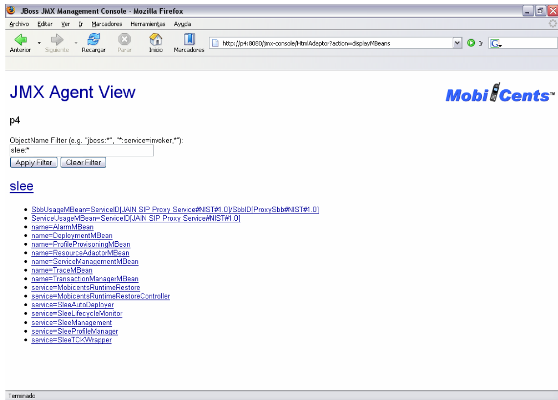
Ilustración 4: Consola JMX.
