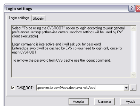
Ilustración 1: WinCvs - Login.
