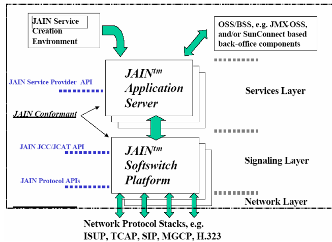
Figura 2.4: Arquitectura JAIN.
