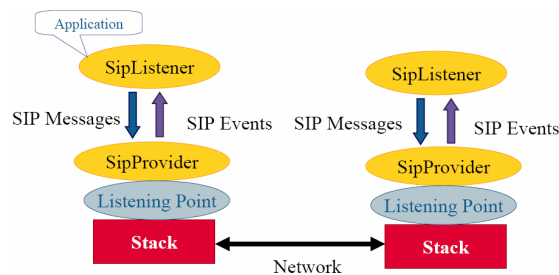
Figura 2.5: Arquitectura de la mensajería JAIN SIP.
