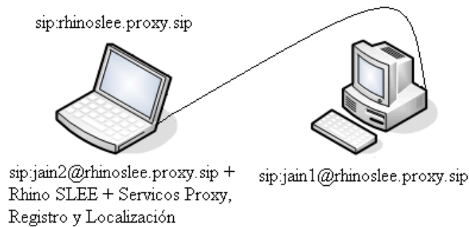
Figura 4.27: Red VoIP alternativa.
