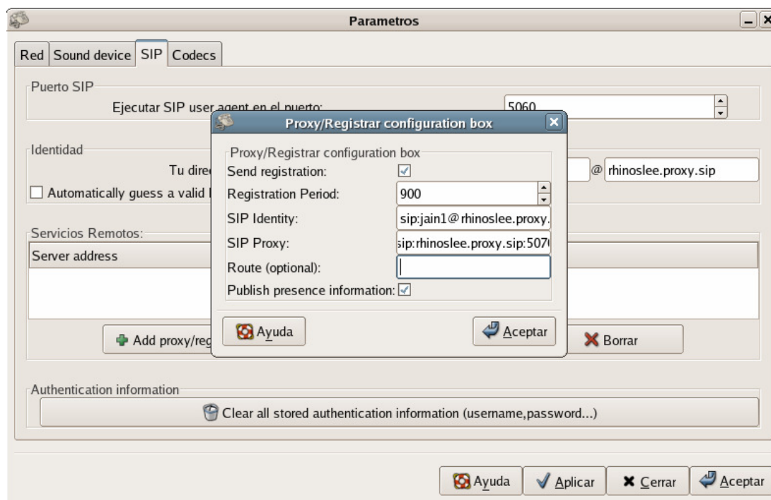
Figura 4.29: Cambio de la configuración del proxy.
