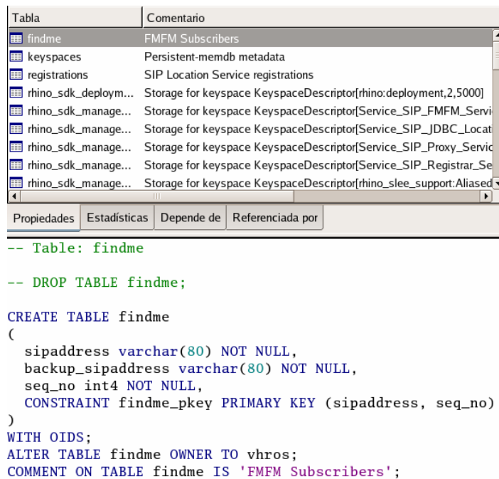
Figura 4.45: Tabla findme en la base de datos rhino_sdk .
