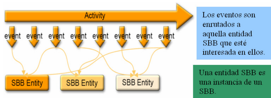
Figura 3.4: Actividad.
