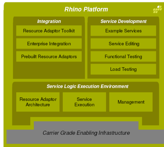
Figura 3.7: Plataforma Rhino.
