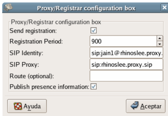
Figura 4.21: Configuración correcta.
