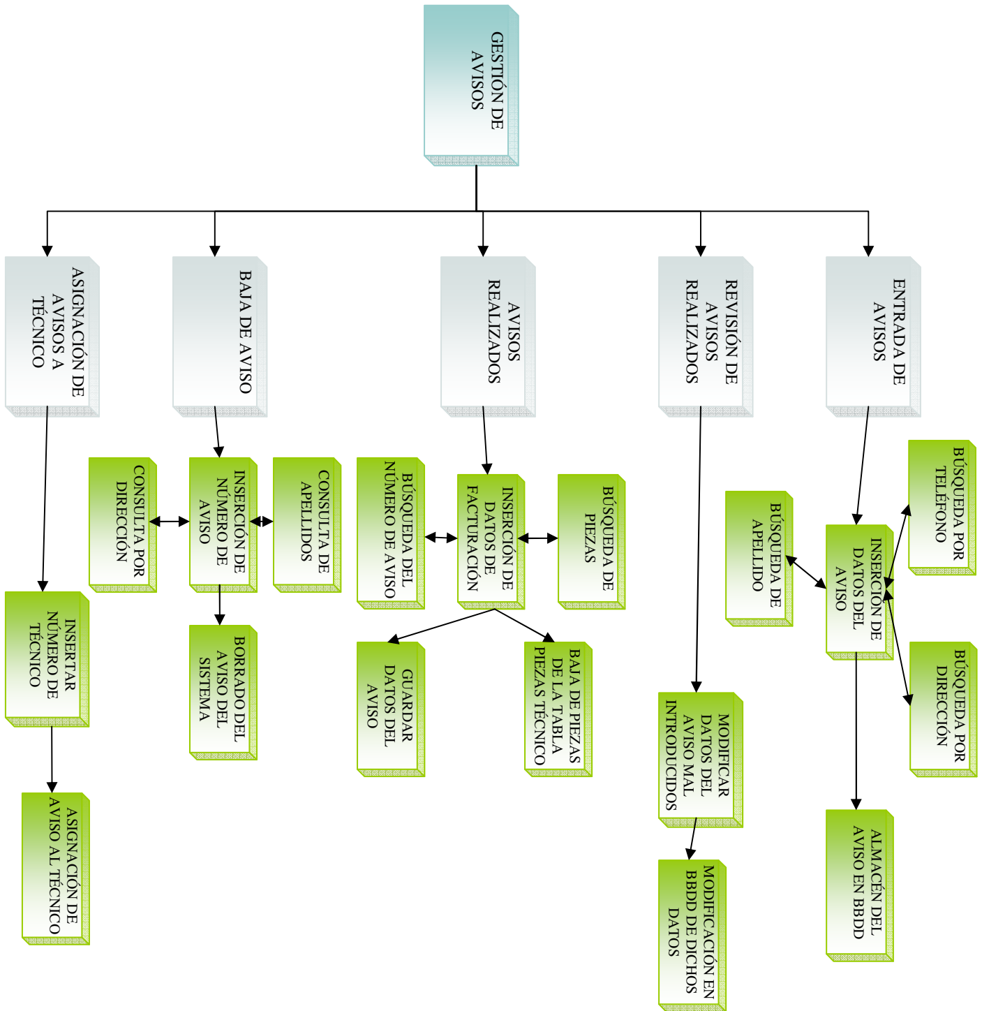
Figura 26. Diagrama de Detalle de la Gestión de Avisos
