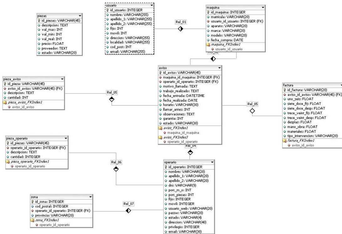
Figura 33. Base de Datos del Sistema
