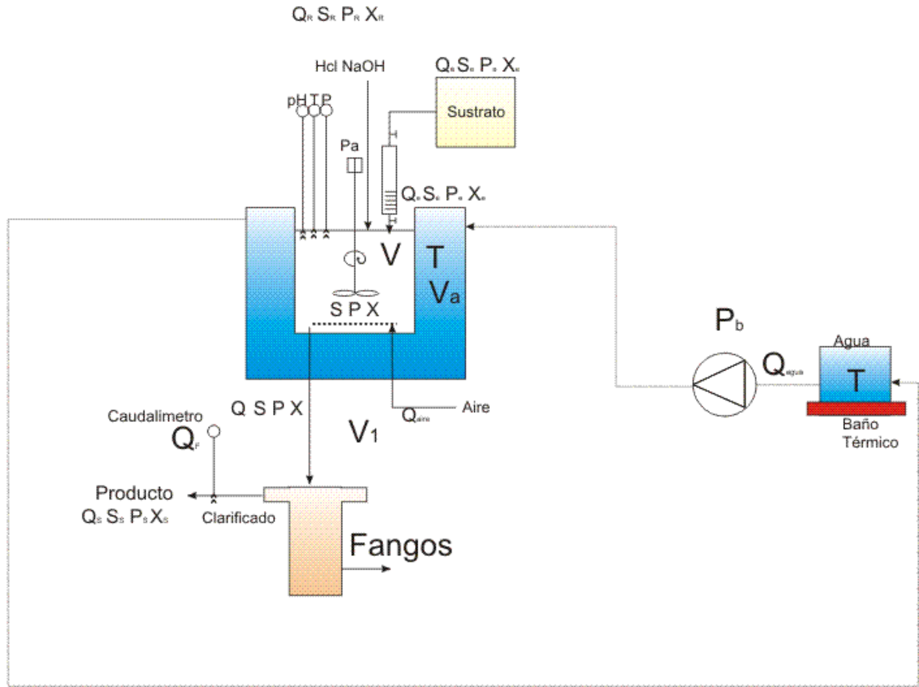
Esquema 1. Reactor tanque mezcla perfecta en discontinuo
