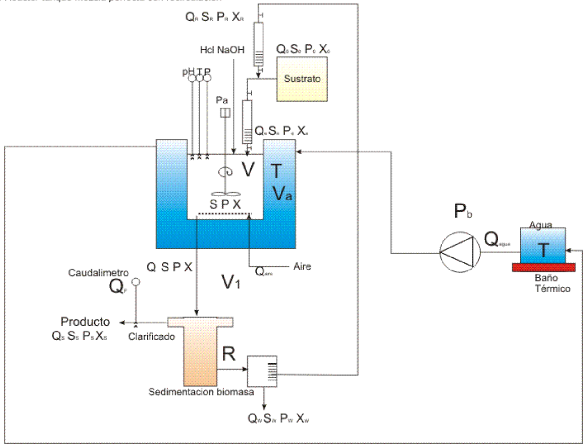
Esquema 5. Reactor tanque mezcla perfecta con recirculación
