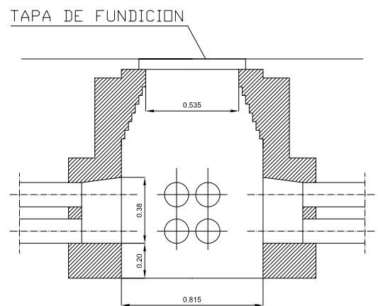
SECCION B - B'
