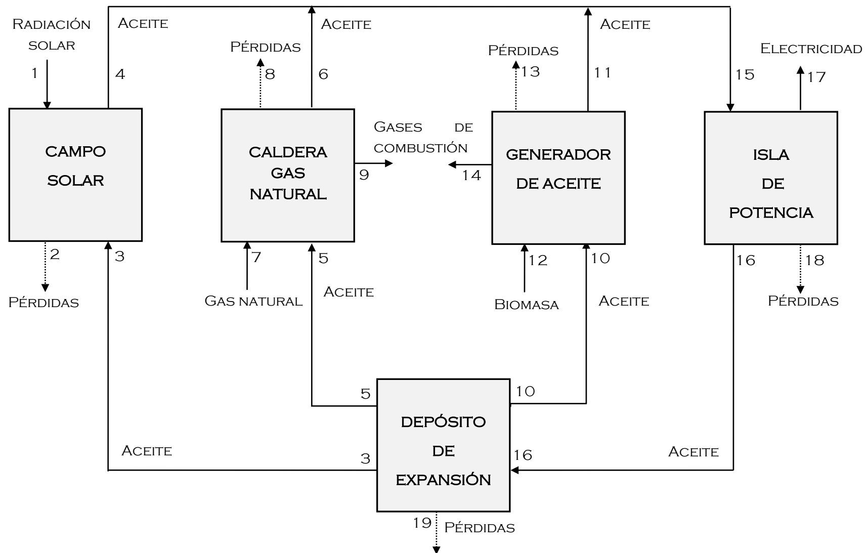
DIAGRAMA DESCRIPTIVO DE TODAS LA CORRIENTES PRESENTES EN LA CENTRAL TERMOSOLAR DE CCP
