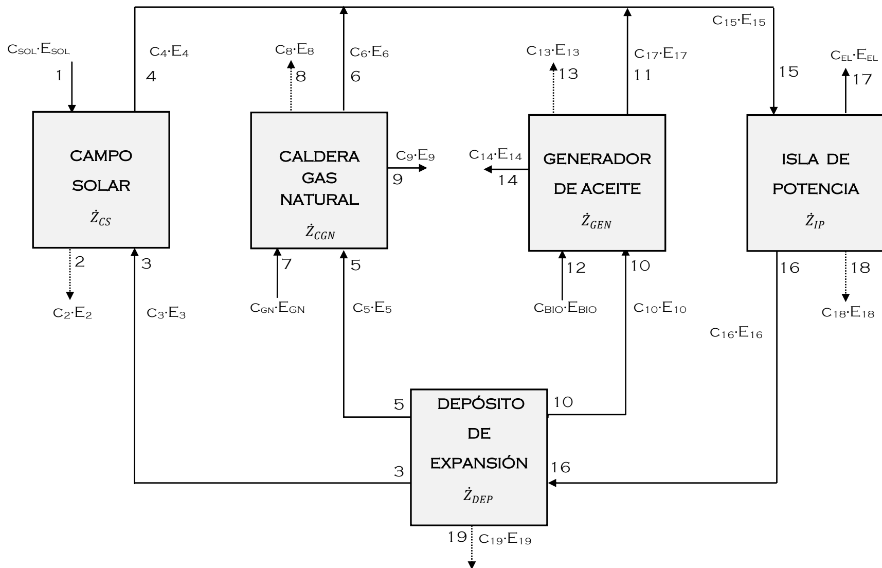
DIAGRAMA DE FLUJOS EXERGEOECONÓMICOS DE LA CENTRAL DE CCP
