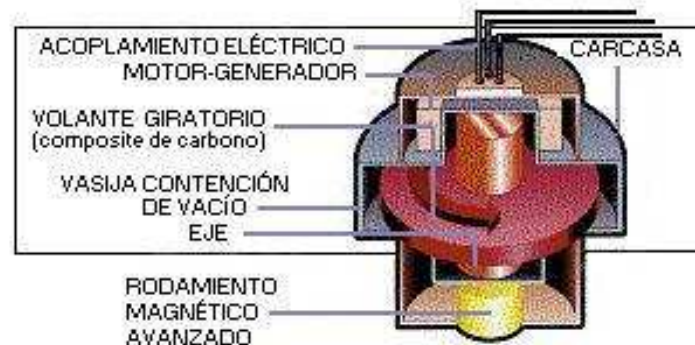
Figura 2.5 Componentes de un volante de inercia.
