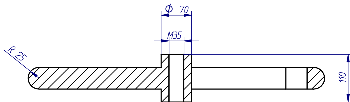
CORTE A-A
