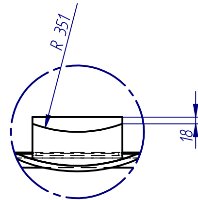
DETALLE A
