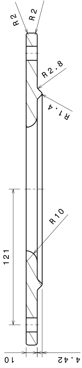
Sección A-A
