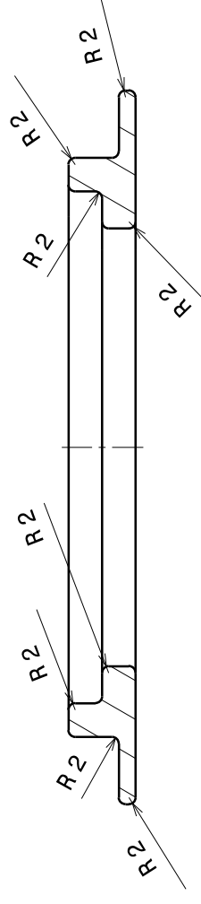
Sección A-A
