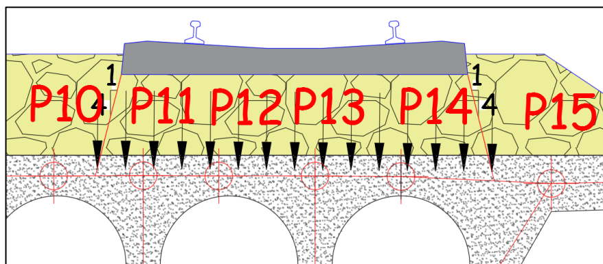
Figura 17. Reparto de cargas en los nodos bajo el carril.
