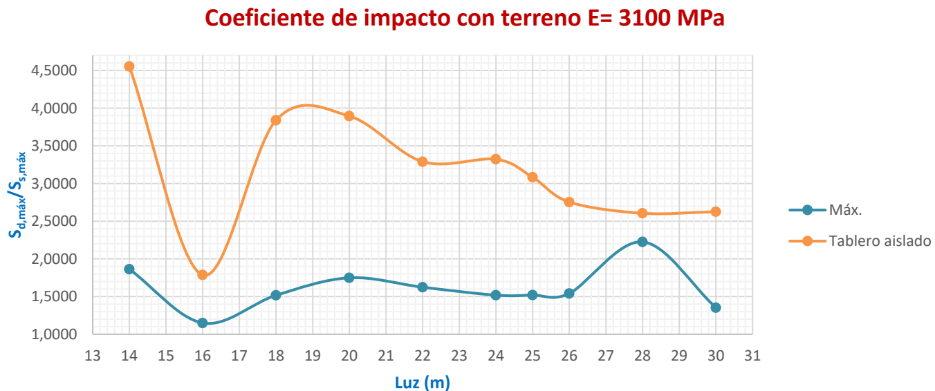
Figura 47. Comparativo coeficiente de impacto con terreno, E= 3100 MPa & tablero aislado.
