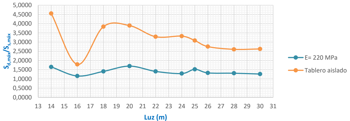
Figura 43. Comparativo coeficiente de impacto con terreno, E=220\text{ MPa} & tablero aislado
