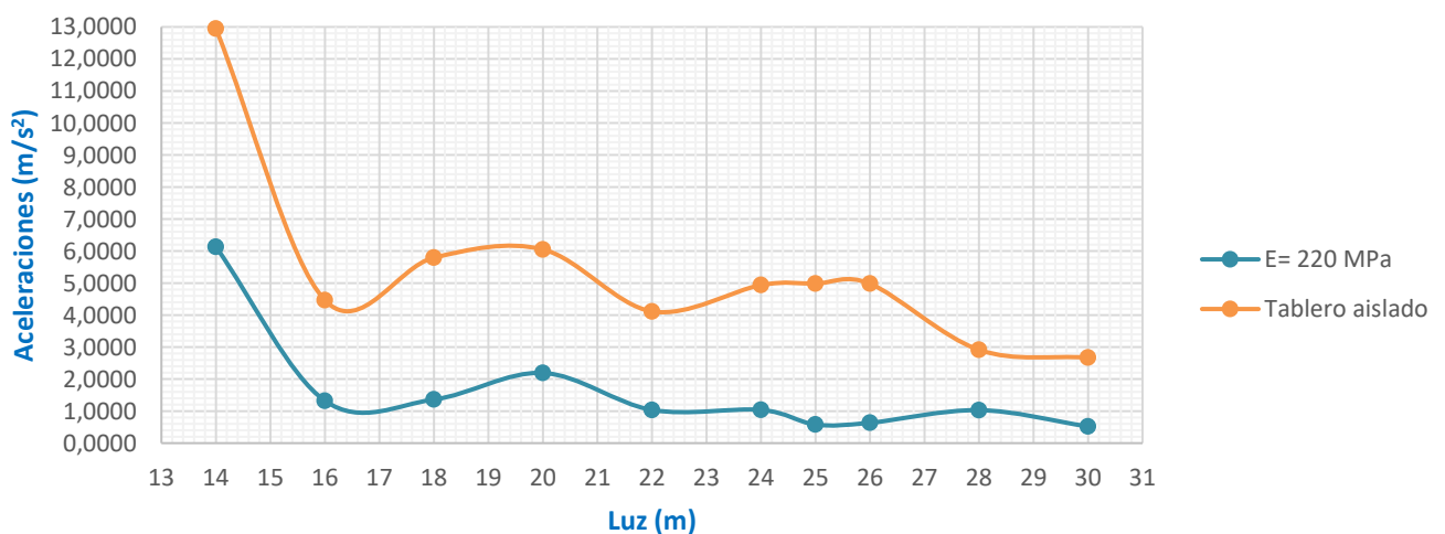
Figura 44. Aceleraciones producidas con terreno E=220\text{ MPa} & Tablero aislado.
