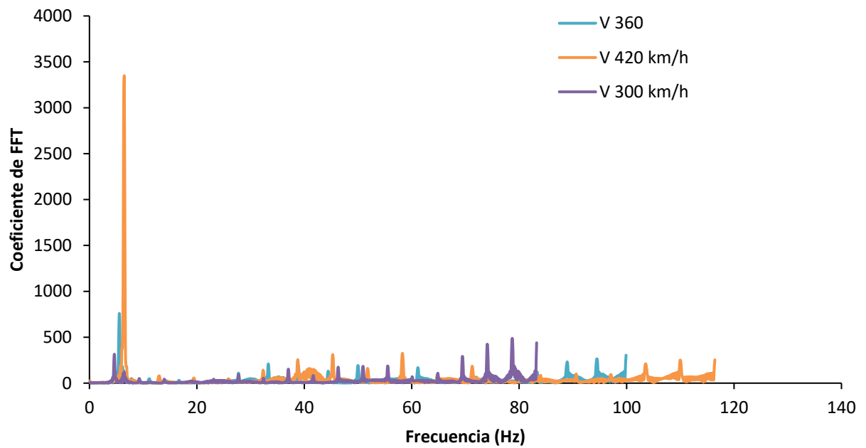
Figura 25. Comparación frecuencias excitadas según velocidad. Tablero 14 metros.
