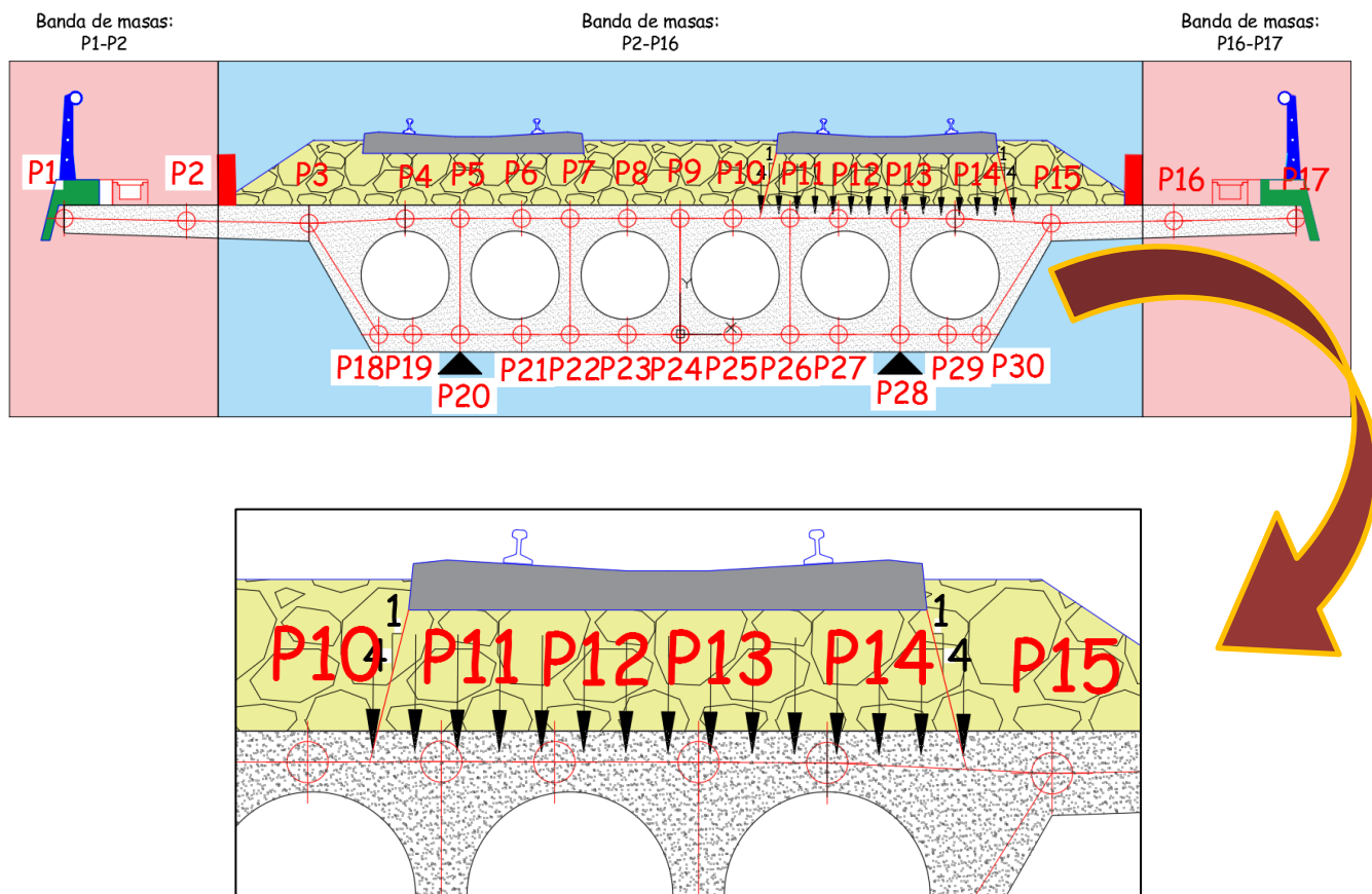
Figura 12. Divisiones en bandas de masas en tablero y puntos de aplicación. Ejemplo tablero 20 metros.
