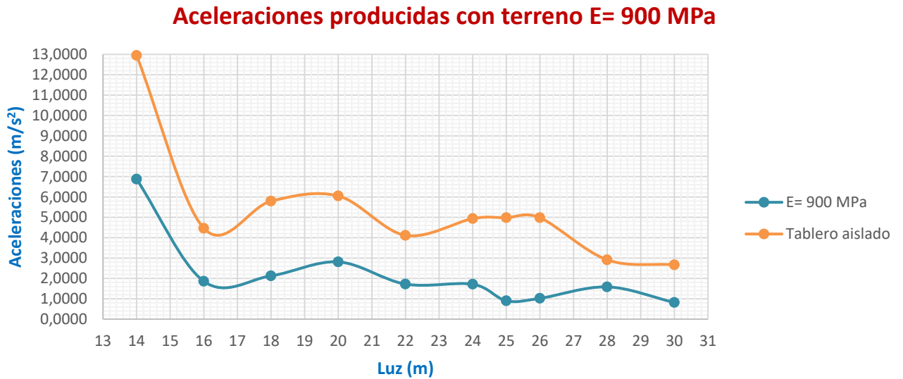
Figura 46. Aceleraciones producidas con terreno E= 900 MPa & Tablero aislado.
