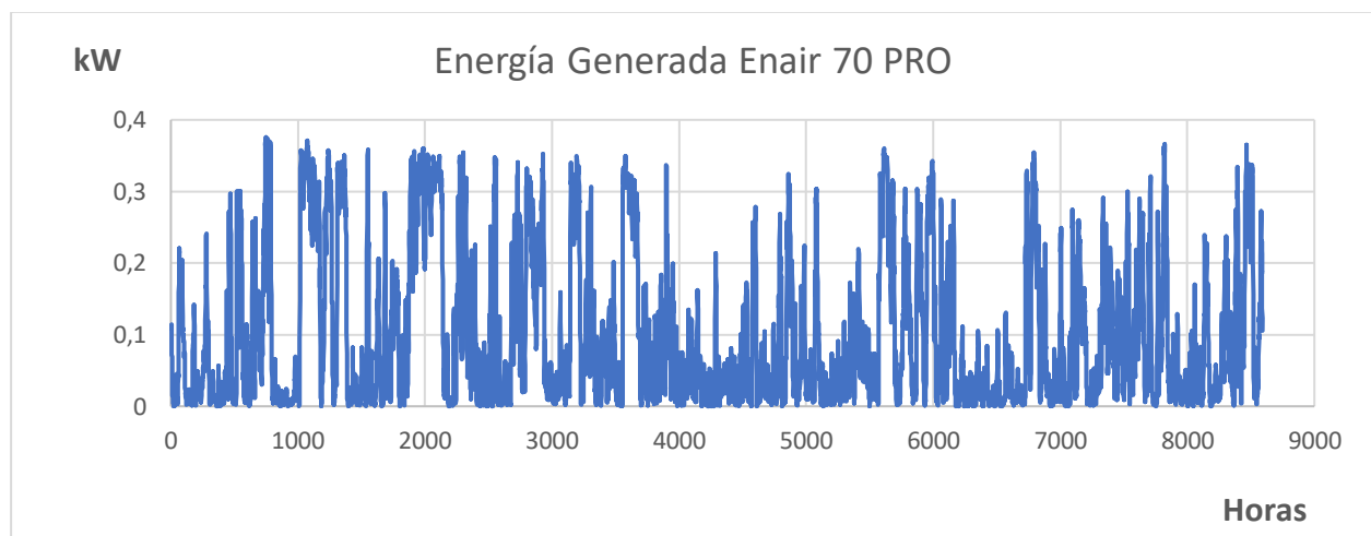
Figura 41. Generación minieólica Enair 70PRO
