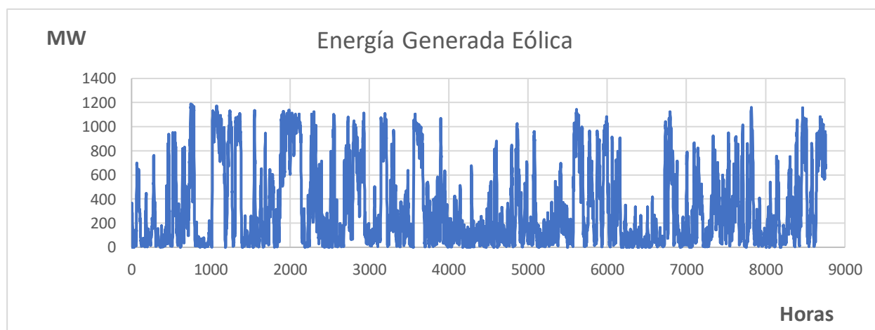
Figura 39. Generación minieólica Cádiz 2019
