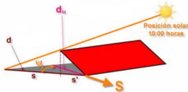
Figura 10. Distancia de sombreado [13]
