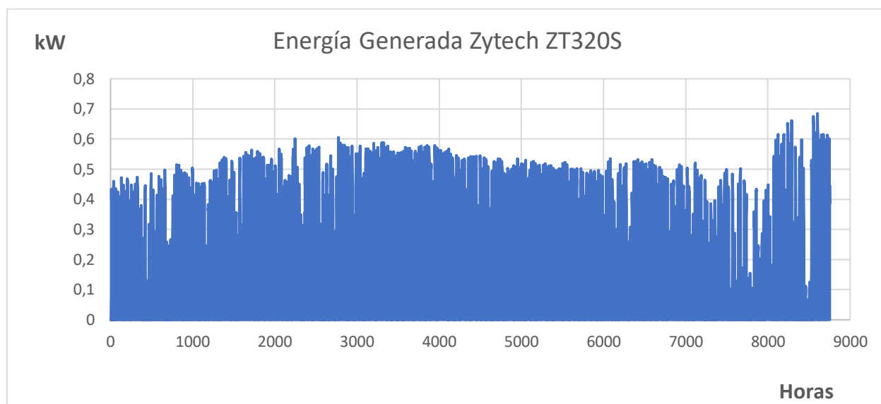
Figura 45. Generación fotovoltaica Zytech ZT320S
