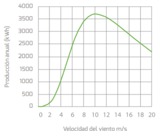
Figura 30. Energía anual Bornay 13+ [24]
