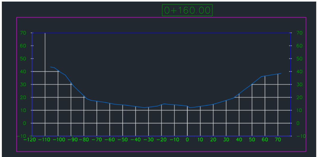
Figura 15: Sección transversal a una longitud de 160 metros.
