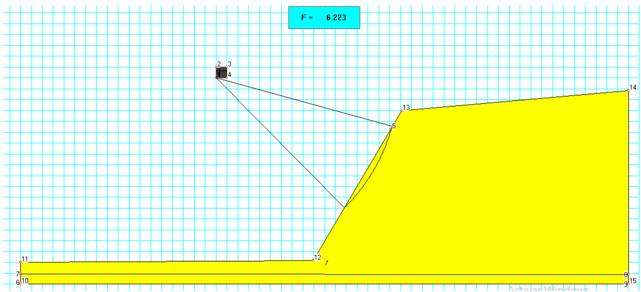
Figura 17: Esquema de simulación del talud para una inclinación de 55°.
