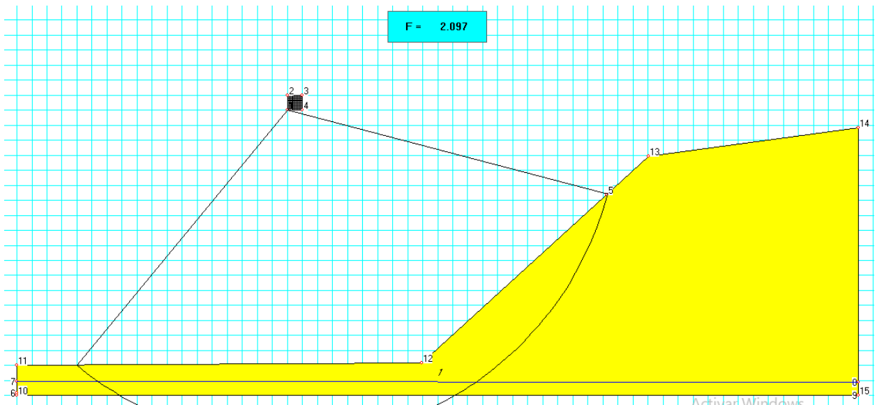
Figura 16: Esquema de simulación del talud para una inclinación de 33°.
