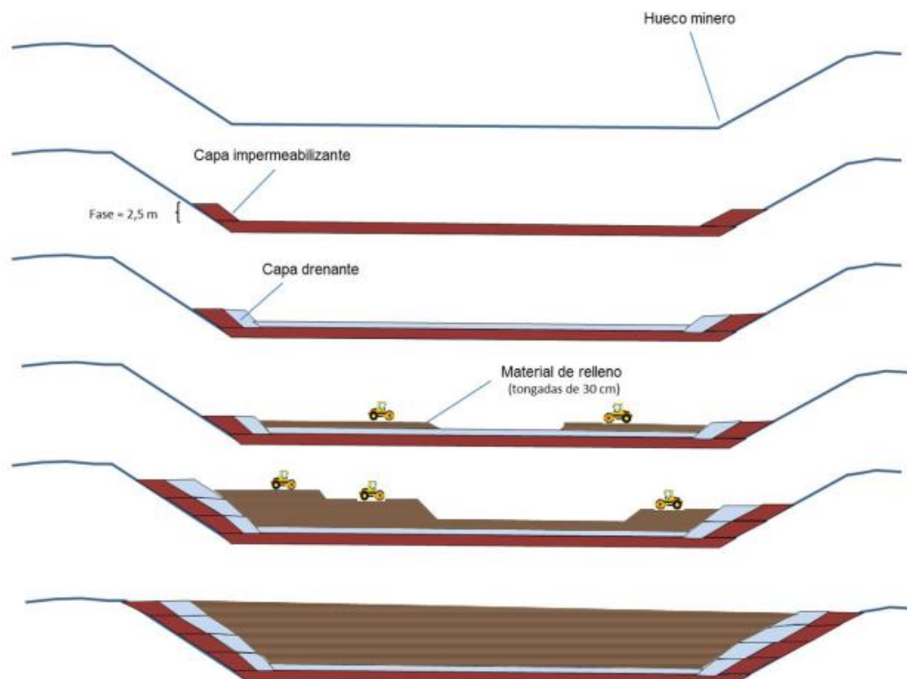
Figura 21: Esquema de procedimiento de relleno de hueco minero
