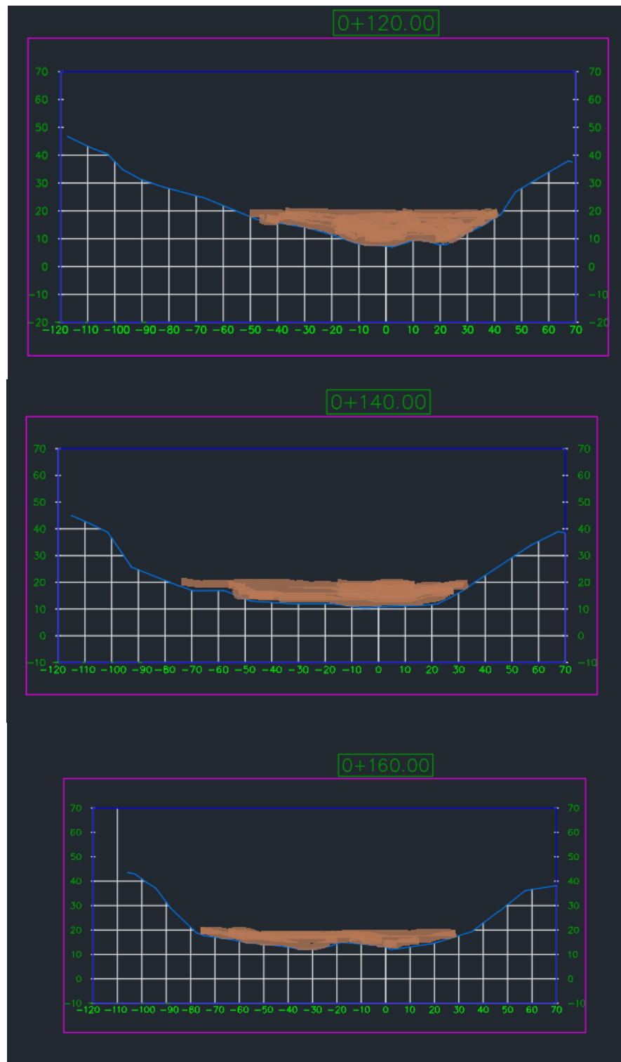
Figura 23: Fase del relleno, nivelación a 20 metros (2).
