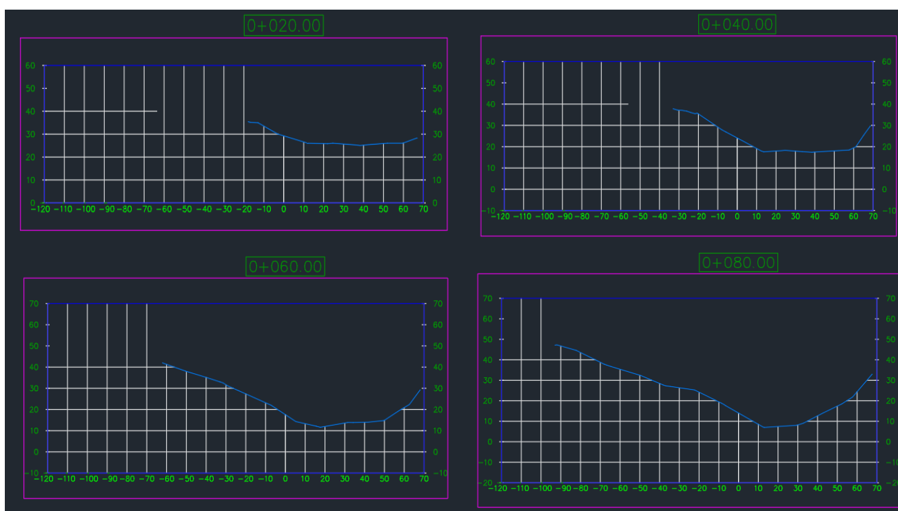
Figura 5: Representación de las secciones transversales de 0 a 80 m.
