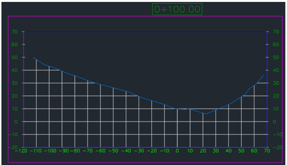
Figura 13: Sección transversal a una longitud de 100 metros.
