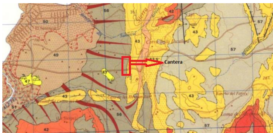
Figura 9: Situación de la cantera en plano geológico
