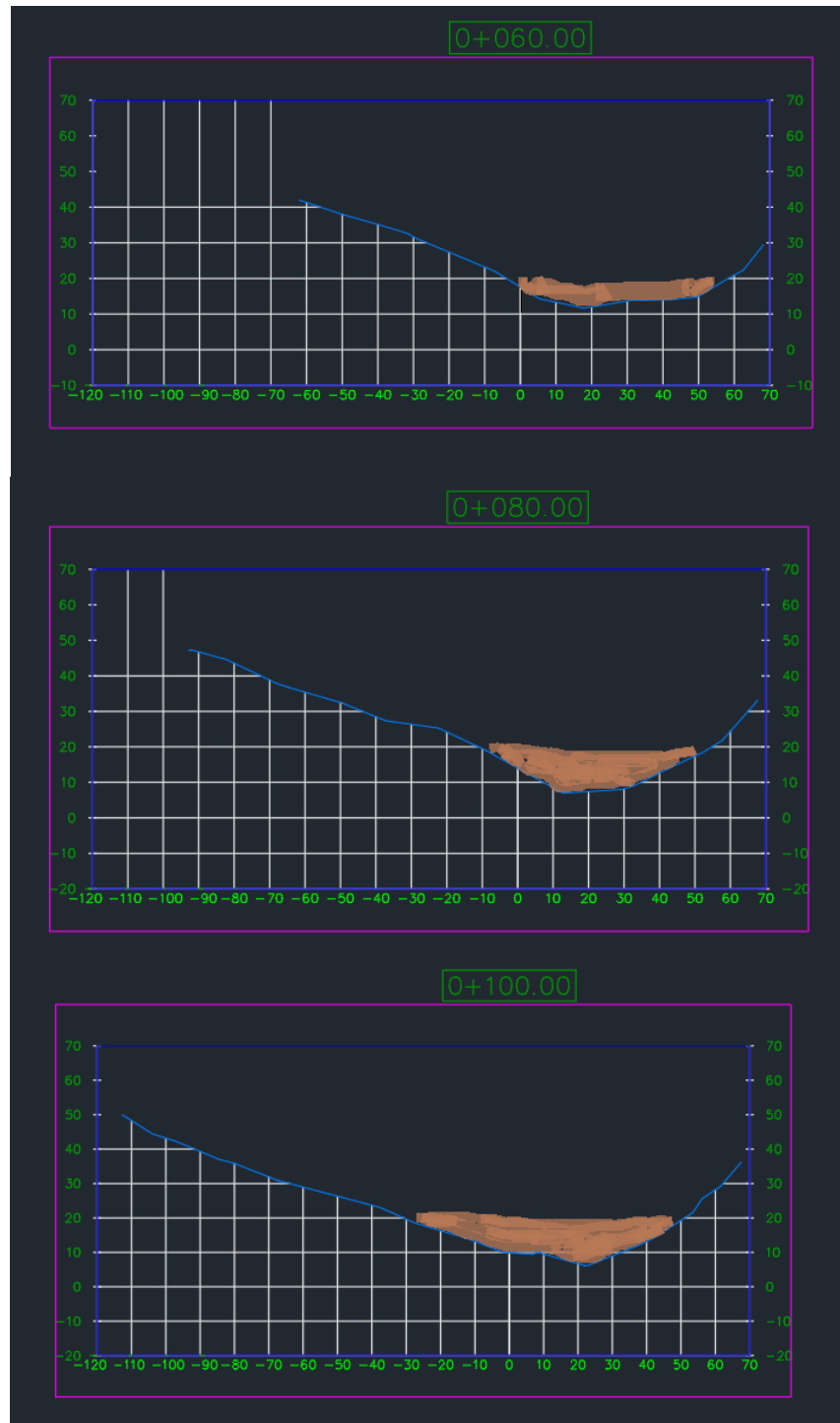
Figura 22: Fase del relleno, nivelación a 20 metros (1).
