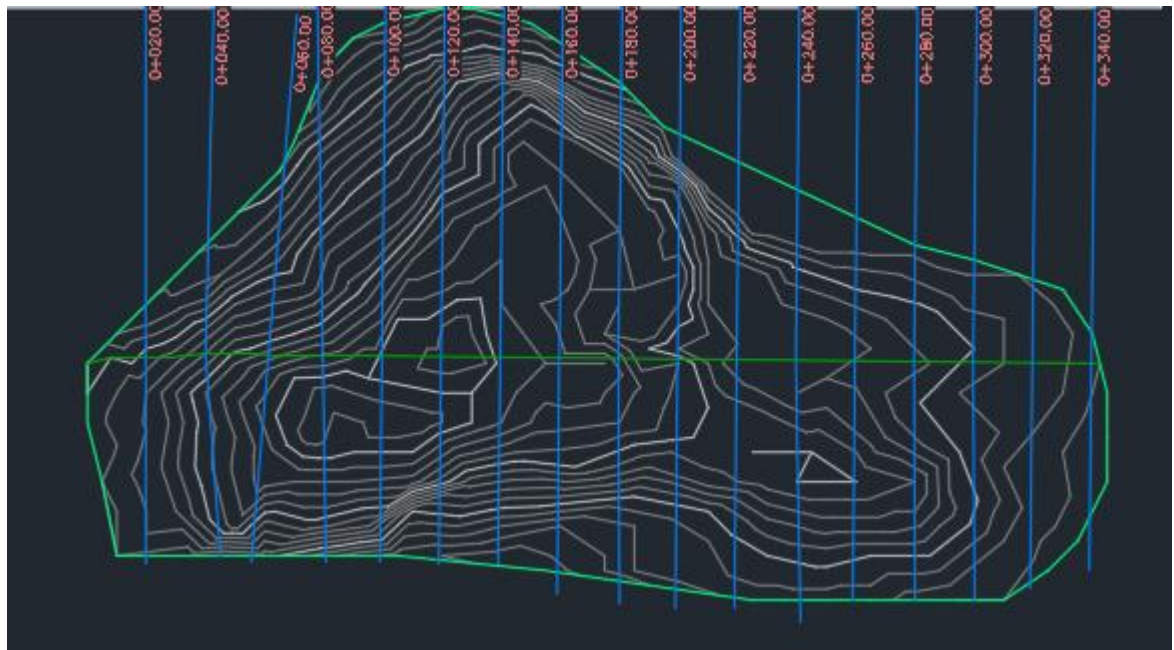
Figura 12: Planta de las secciones transversales del plano de la cantera.
