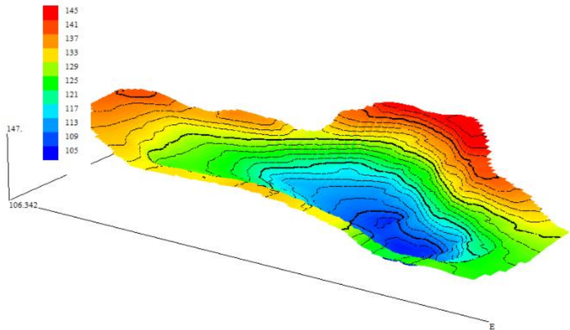
Figura 11: Representación 3D del hueco minero.
