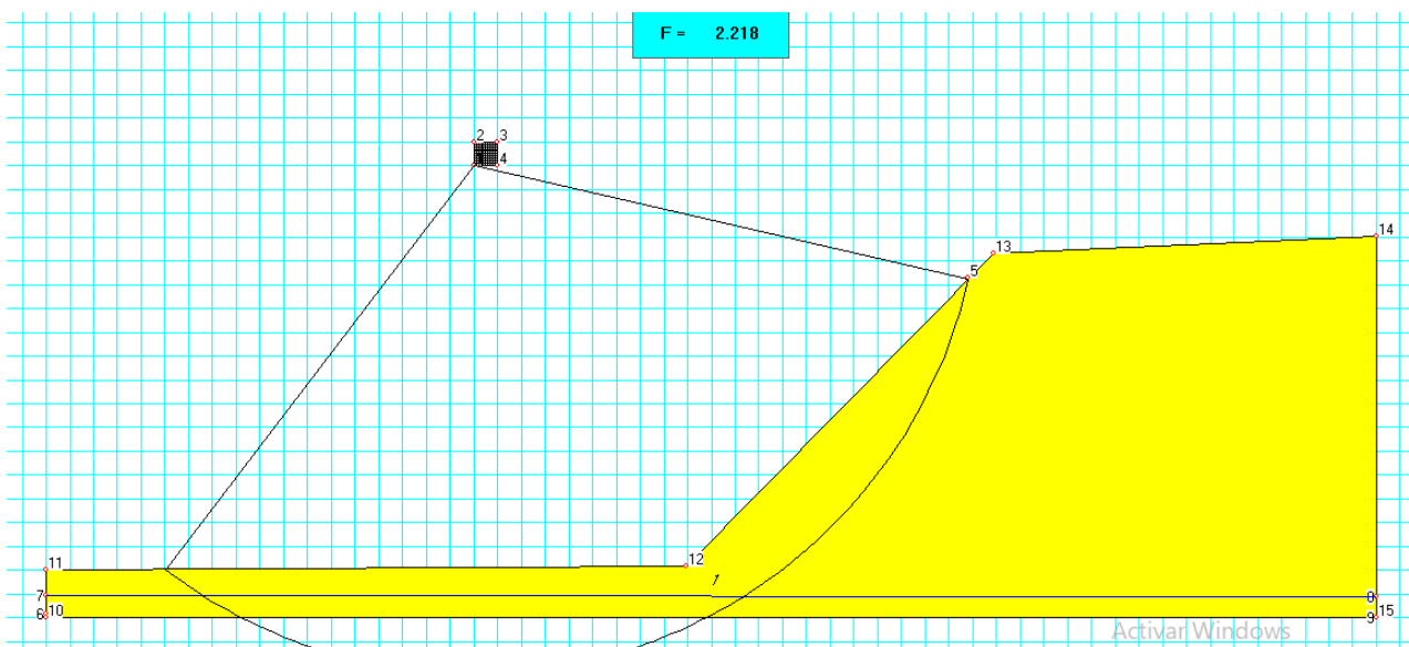
Figura 18: Esquema de simulación del talud para una inclinación de 45°.
