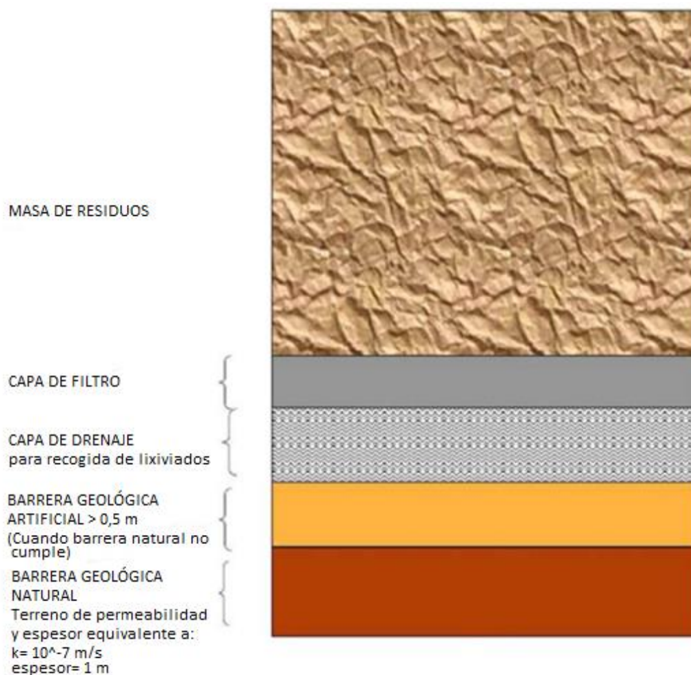
Figura 20: Capas a añadir para la preparación del terreno para la instauración del vertedero de RCD
