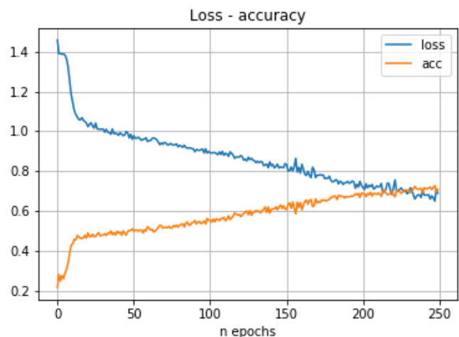
Figura 58. Red neuronal recurrente. Ensayo 6
