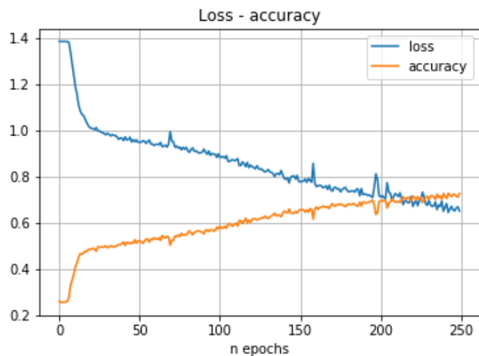
Figura 53. Red neuronal recurrente. Ensayo 1
