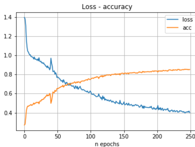
Figura 63. Red neuronal recurrente. Ensayo 11
