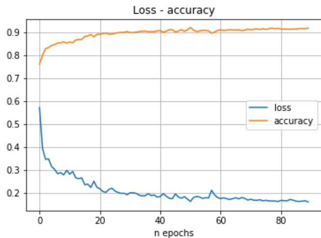
Figura 52. Red neuronal Convolutacional. Ensayo 15
