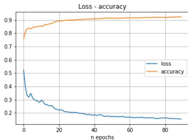
Figura 50. Red neuronal Convolutacional. Ensayo 13
