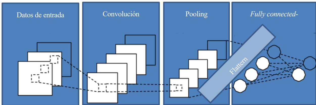
Figura 8. Estructura de la red Convolucional
