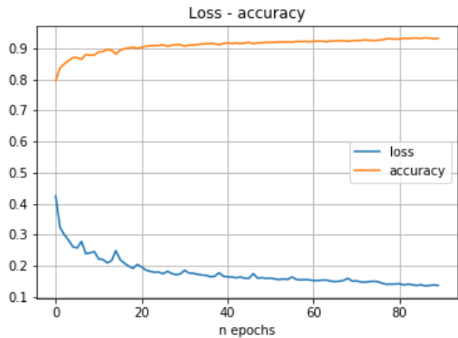
Figura 51. Red neuronal Convolutacional. Ensayo 14
