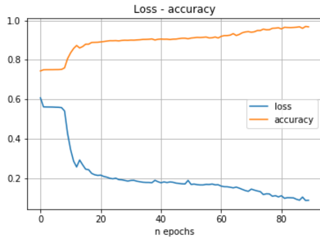
Figura 49. Red neuronal Convolutacional. Ensayo 12
