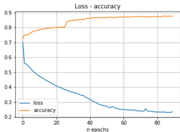
Figura 46. Red neuronal Convolucional. Ensayo 9
