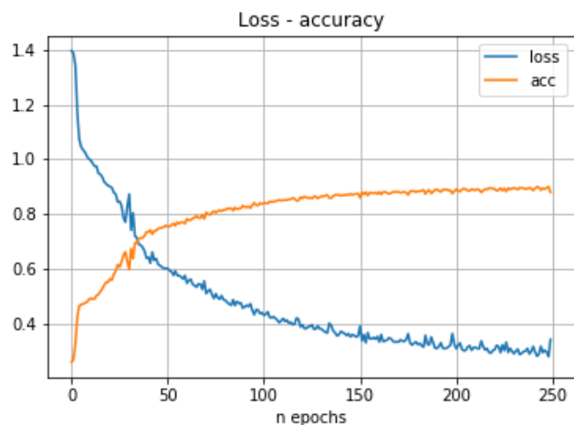
Figura 65. Red neuronal recurrente. Ensayo 13
