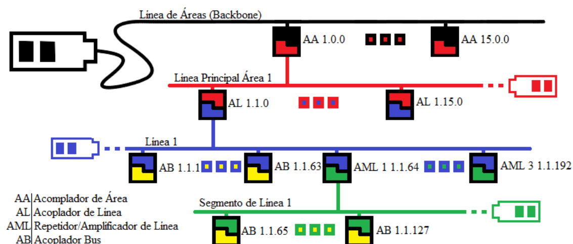
Figura 8 Ejemplo conexión sistema KNX
