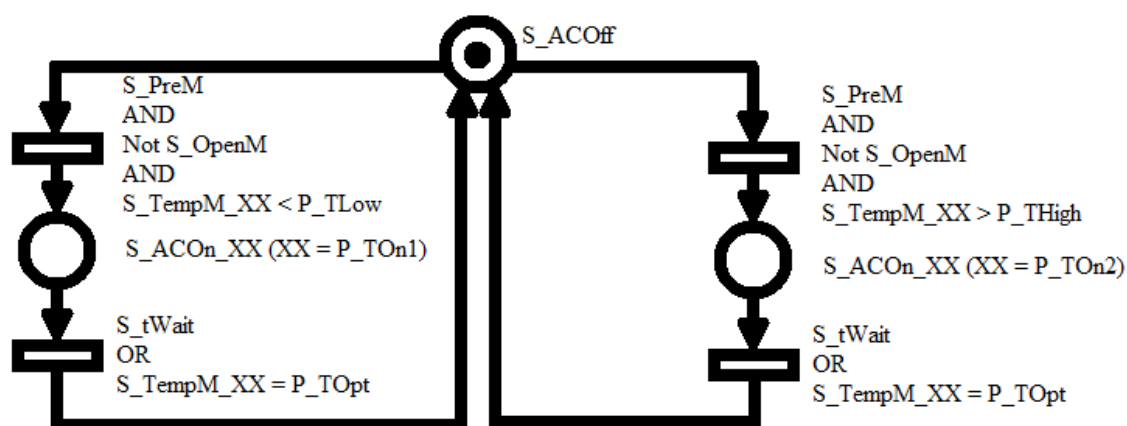
Figura 46 Termostato Inteligente
