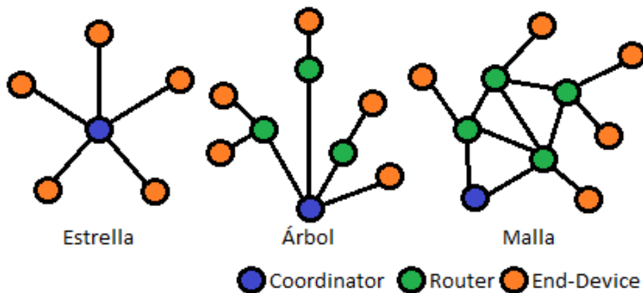
Figura 11 Topologías Zigbee
