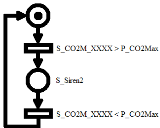
Figura 51 Sirena CO2 máximo permitido
