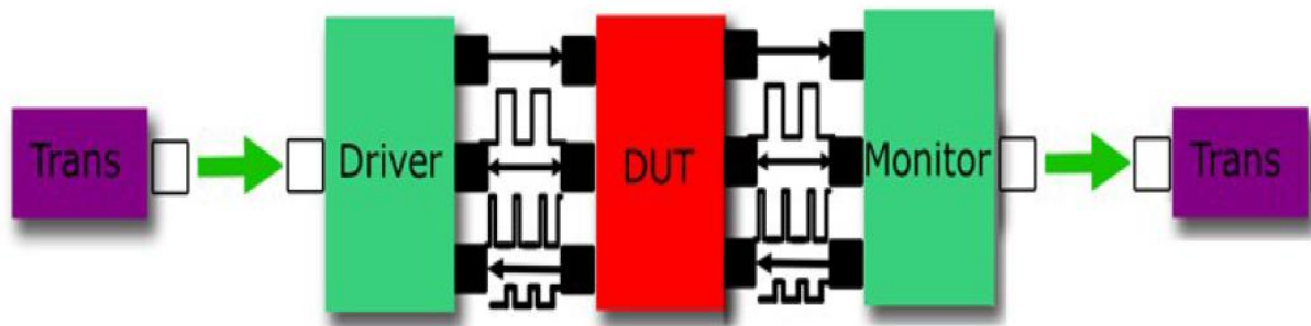
Figura 6-5. Testbench modelado a nivel de transacciones [15]
