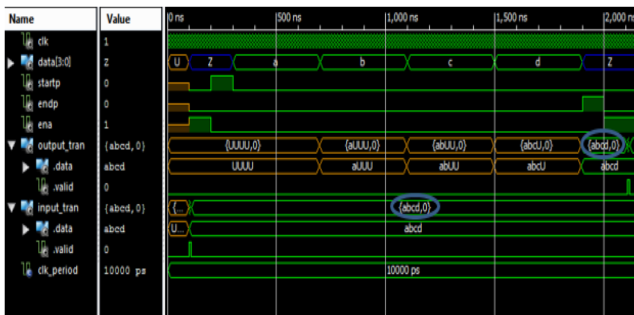
Figura 6-18. Simulación Monitor Protocolo ficticio – formato hexadecimal
