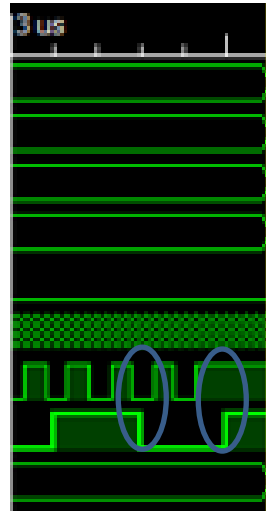
Figura 6-10. Secuencia de parada del protocolo I2C
