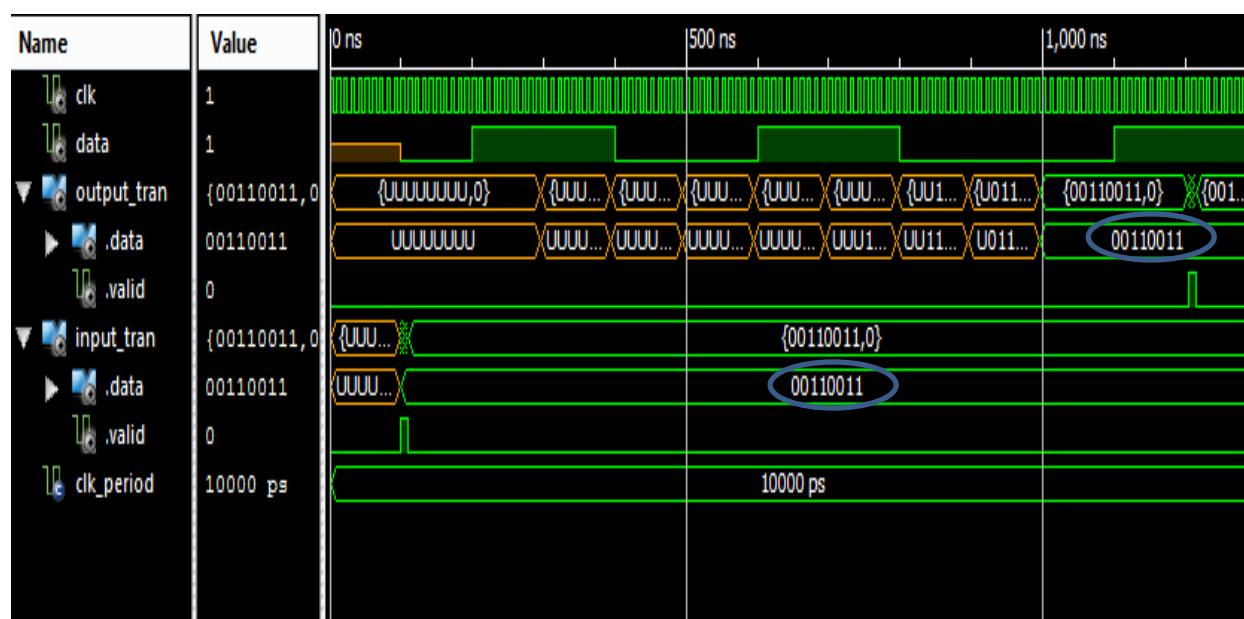
Figura 6-7. Simulación Monitor del protocolo UART
