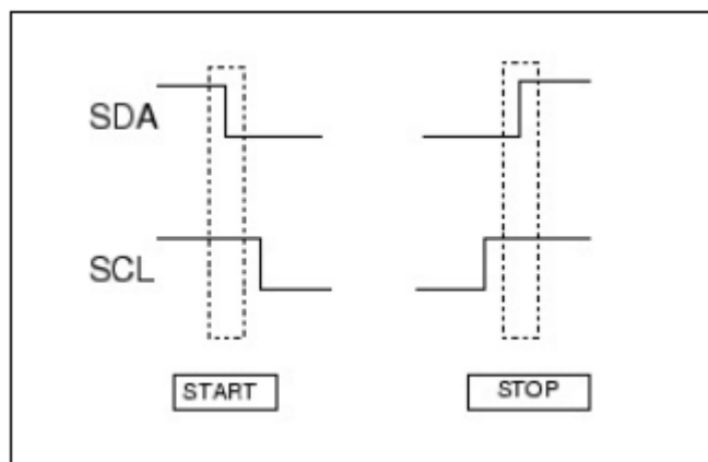
Figura 3-8. Condiciones de Inicio y parada del protocolo I2C [17]
