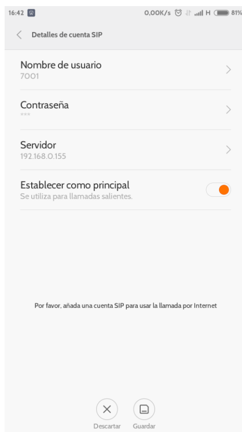
Figura 0-13: Configuración de cuenta SIP
