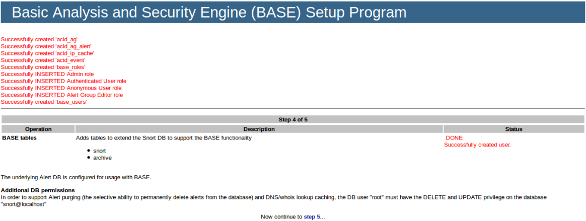
Figura 0-7: Paso 5 en la configuración de BASE
