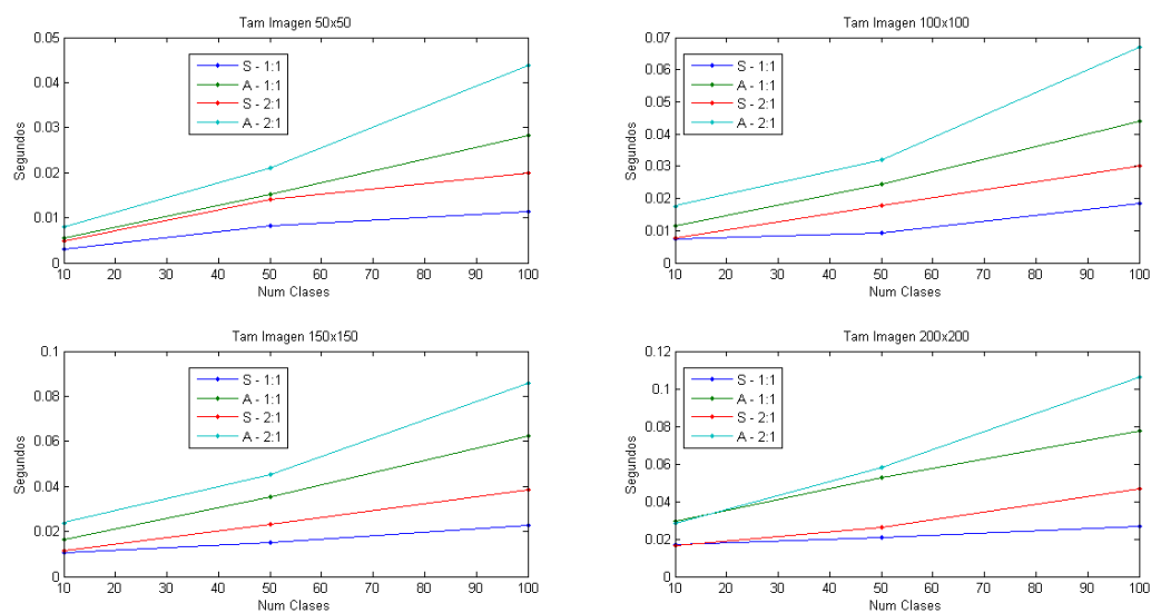
Figura 21. Tiempos medios de identificación del modelo LBPFace.
