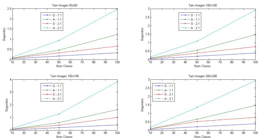
Figura 18. Tiempos de carga del modelo LBPHFace.
