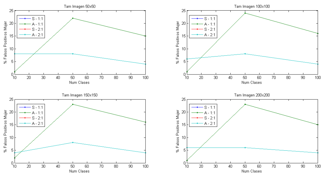
Figura 25. Porcentajes de falsos positivos en mujeres del modelo EigenFace.
