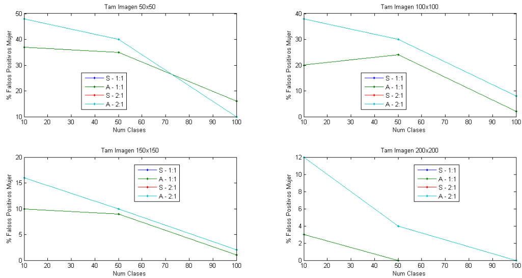
Figura 27. Porcentajes de falsos positivos en mujeres del modelo LBPHFace.
