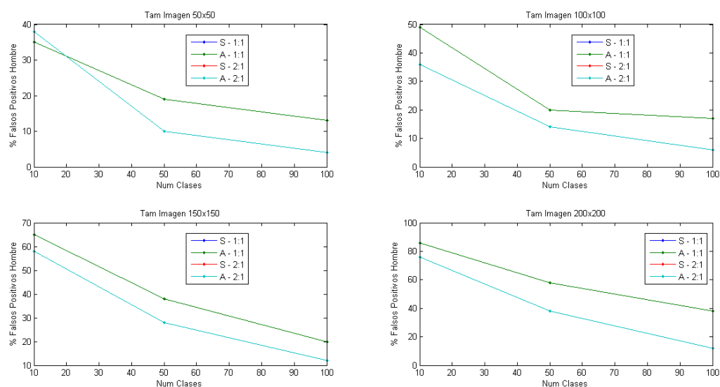
Figura 30. Porcentajes de falsos positivos en hombres del modelo LBPHFace
