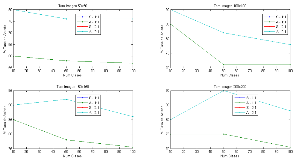
Figura 33. Porcentajes de tasas de acierto del modelo LBPHFace.
