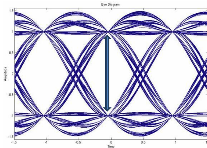
Figura 5-3. Diagrama de ojo
