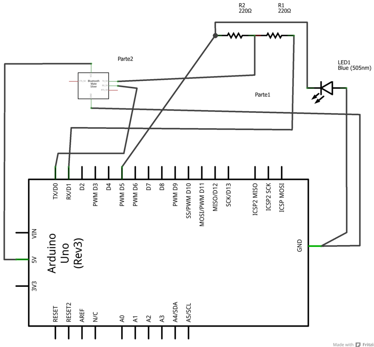
Figura 7-21. Esquemático del sistema receptor
