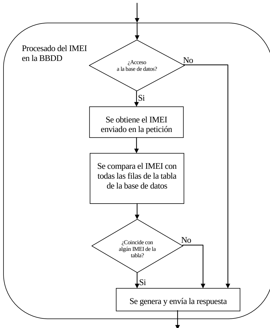
Figura 5-10. Diagrama de flujo de los procesos en la base de datos
