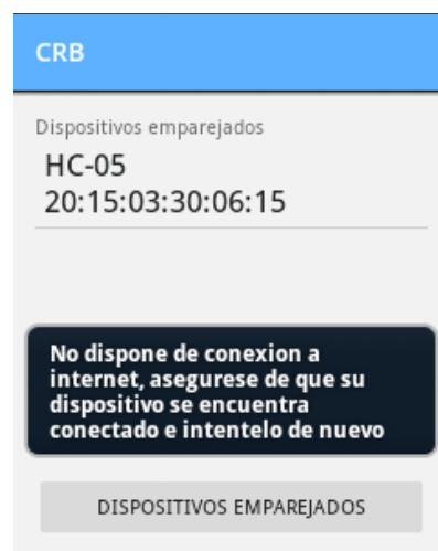
Figura 7-14. Mensaje mostrado por la aplicación en caso de no tener conexión a internet.
