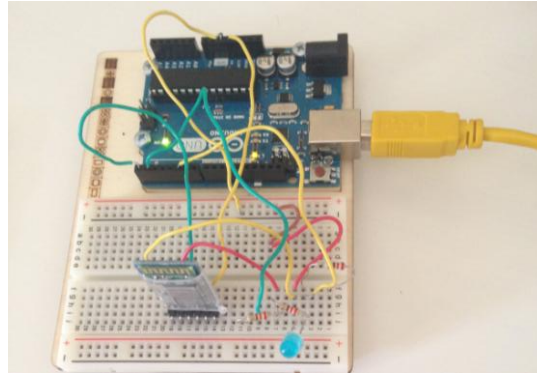
Figura 7-19. Sistema Arduino y Bluetooth para la recepción del IMEI del dispositivo móvil.
