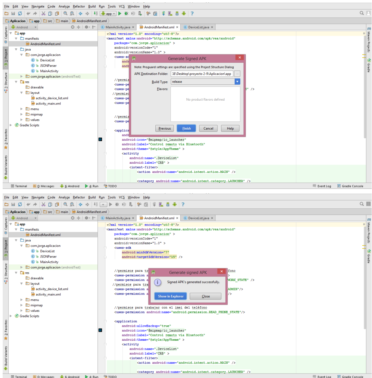
Figura 7-2. Proceso de generación del archivo de instalación de la aplicación en el dispositivo móvil.
