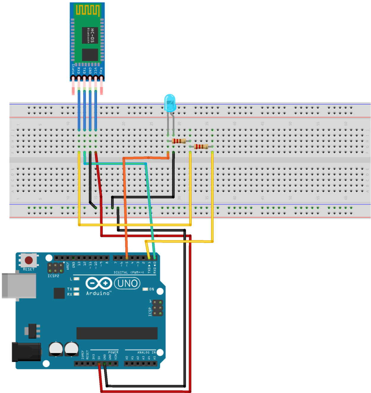
Figura 7-20. Protoboard del sistema receptor
