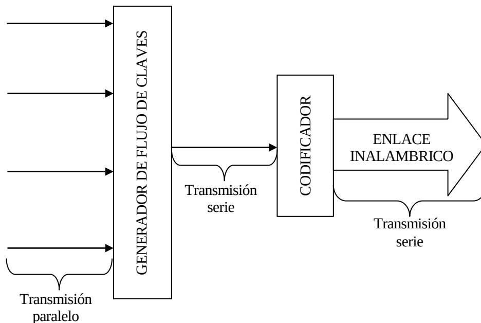
Figura 3-2. Comparación de la transmisión serie y paralelo
