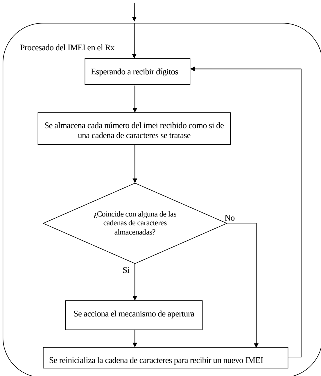
Figura 5-9. Diagrama de flujo los procesos en el sistema receptor
