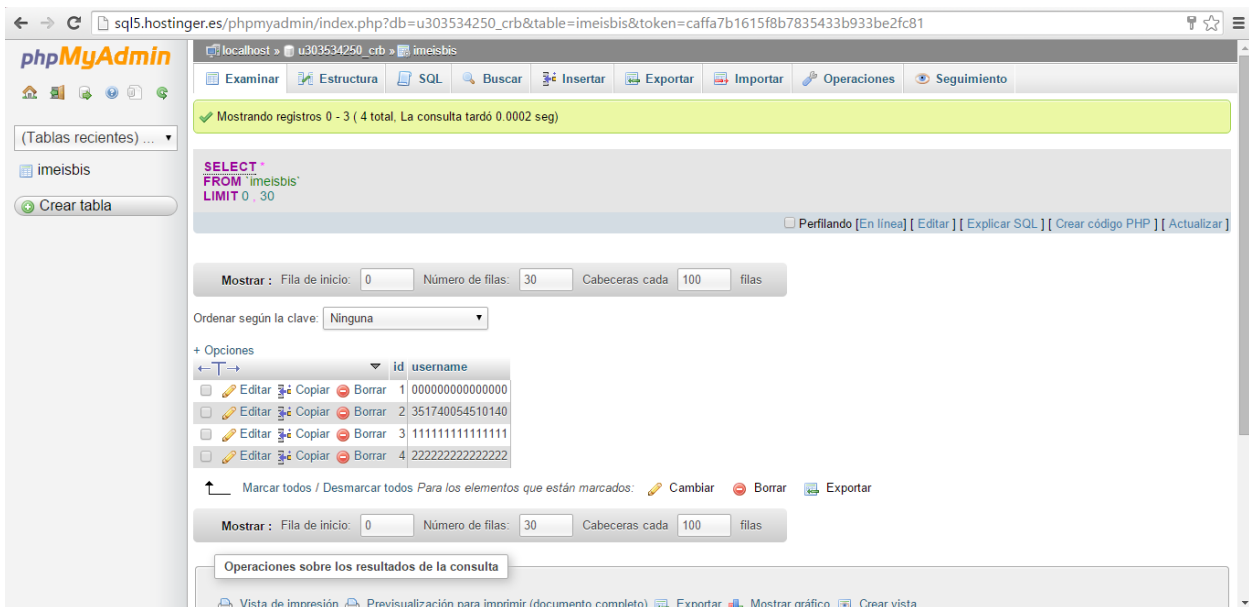
Figura 7-23. Vista previa de la creación de la tabla donde están almacenados los IMEI's (columna username).
