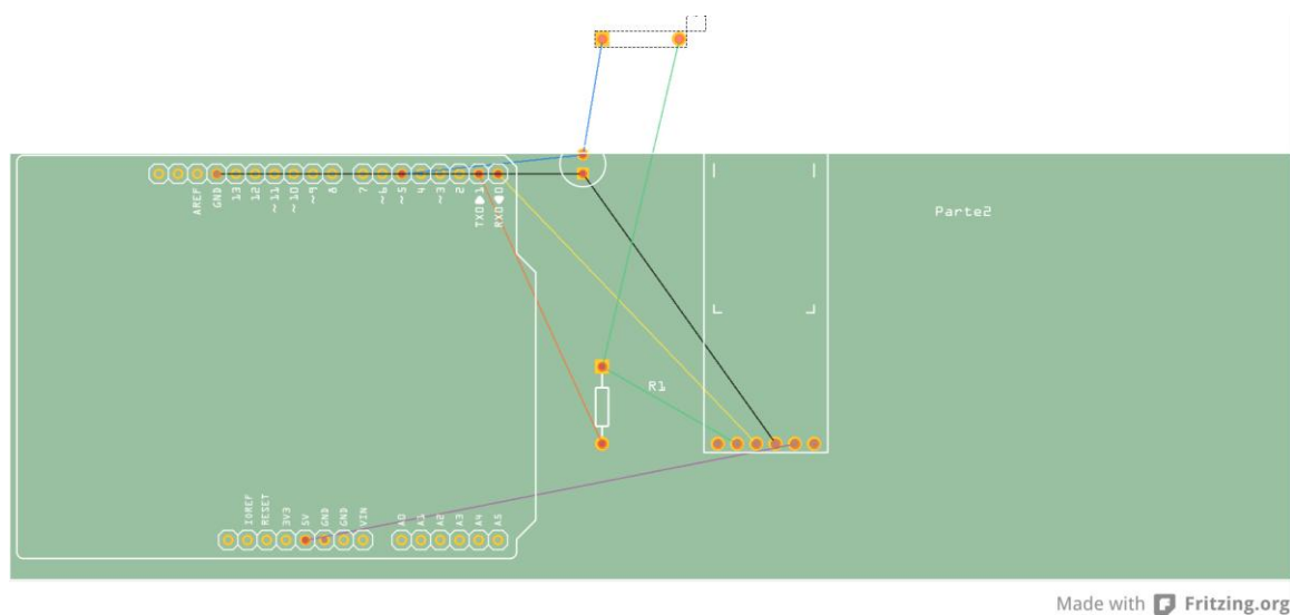
Figura 7-22. PCB del sistema receptor
