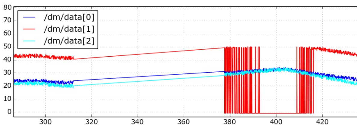
Figura 4-106. ROS, Medidas recibidas por el PF
