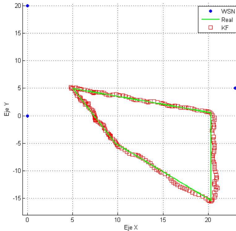
Figura 4-50. Cuadrilátero, sensores w_r = 0,5 \text{ m} , modelo v = 0,1 \text{ m}
