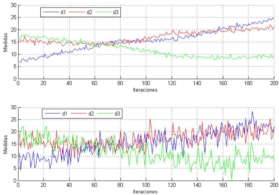
Figura 4-42. Zigzag, distancias medidas con sensores de: a) w_r = 0,5 \text{ m} , b) w_r = 2,5 \text{ m}
