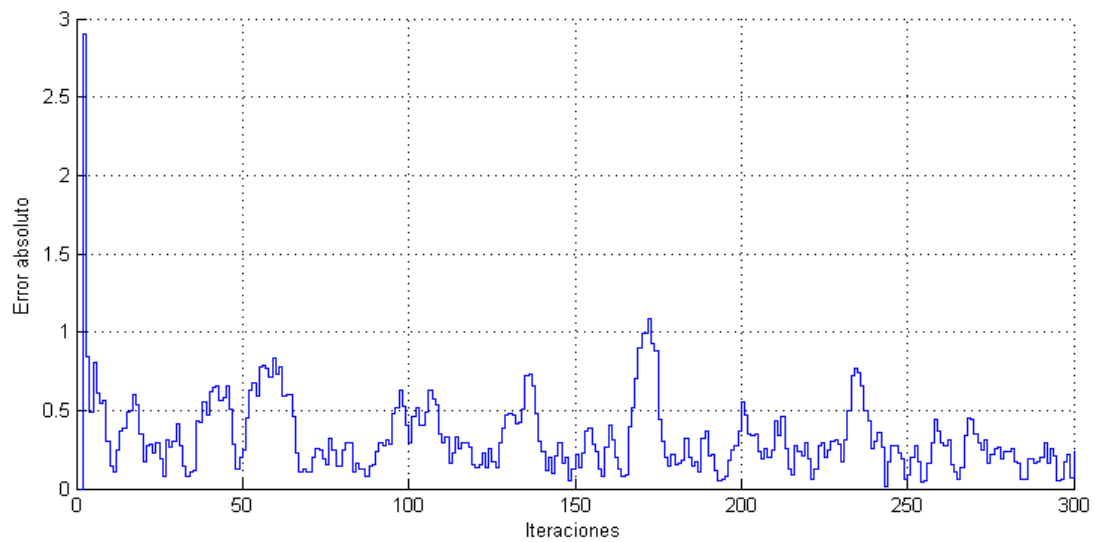
Figura 4-90. PF-2, Error, Uso de 200 partículas
