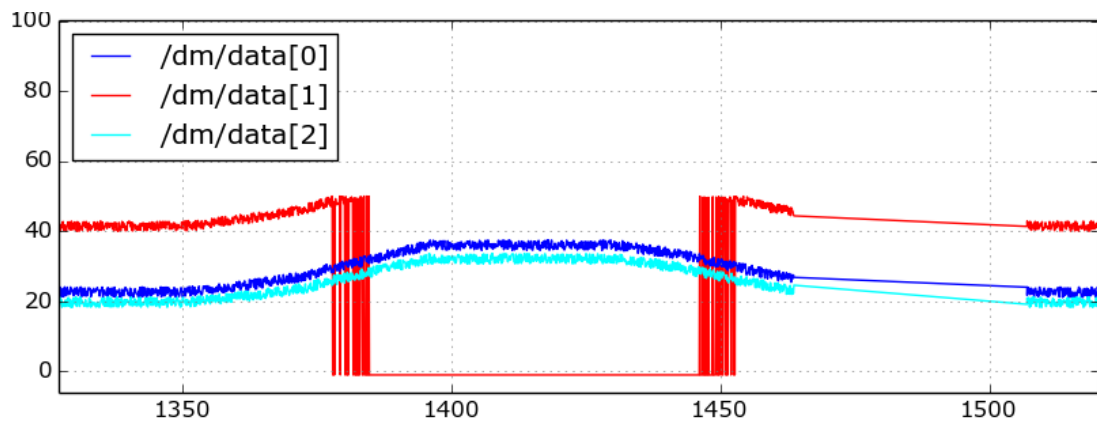
Figura 4-68. ROS, Medidas recibidas por el EIF
