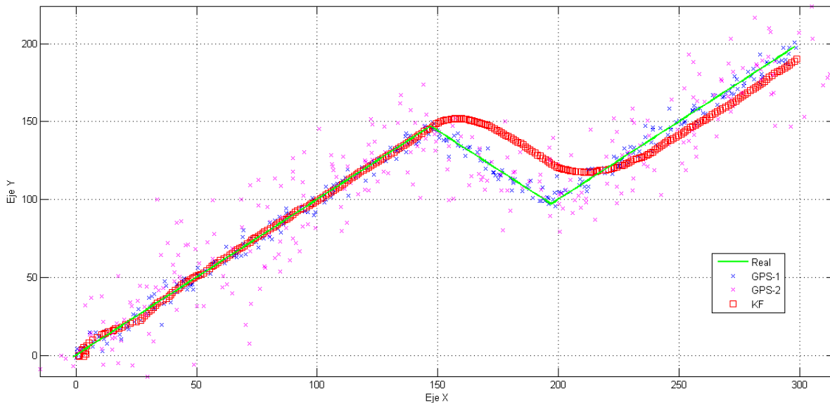
Figura 4-8. Uso de 2 GPS, dispersiones: w_{g1} = 3\text{ m} , w_{g2} = 15\text{ m}
