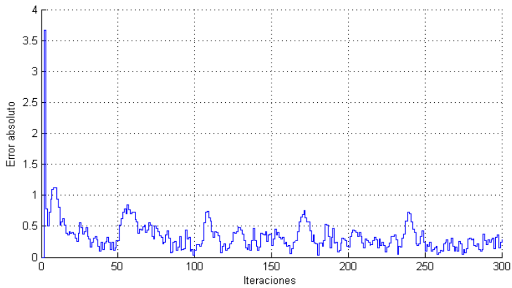
Figura 4-93. PF-2, Error, Uso de 500 partículas
