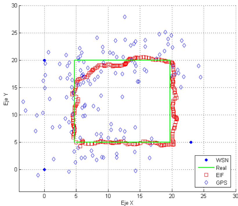
Figura 4-64. Cuadrado, sensores w_r = 0,5 \text{ m} , w_g = 3 \text{ m} , modelo v = 0,1 \text{ m}
