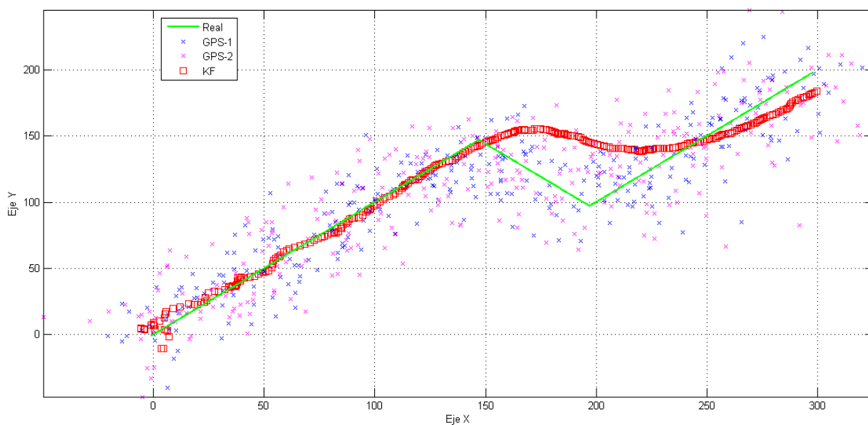
Figura 4-6. Uso de dos GPS, misma dispersión, w_g = 15\text{ m}
