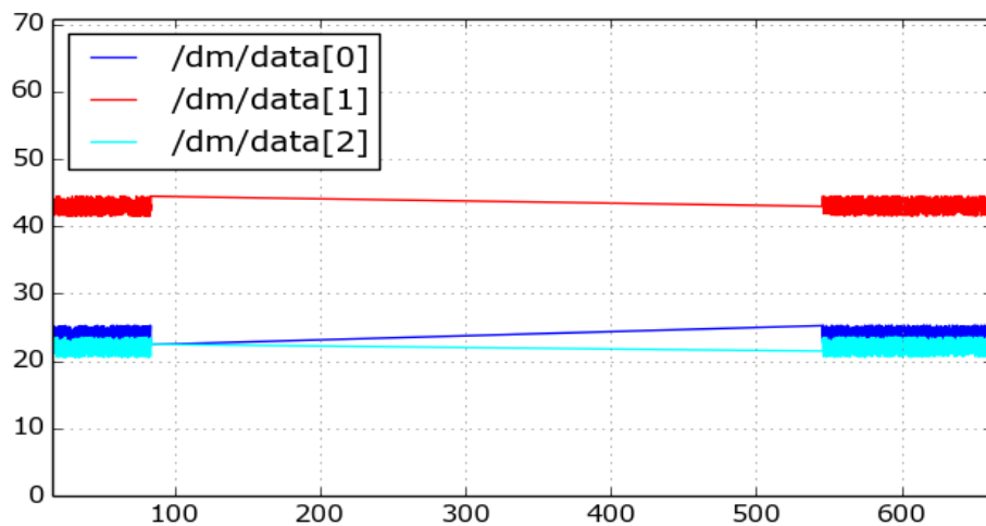
Figura 4-55. ROS, Medidas de rango con tramo sin cobertura
