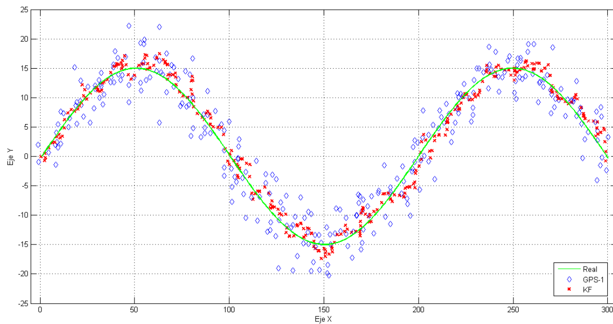
Figura 4-25. Senoide, GPS con w_g = 3\text{ m} , error del modelo: v = 1\text{ m} , a) Modelo rectilíneo, b) Modelo estático
