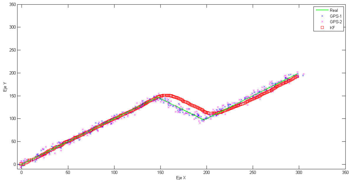
Figura 4-4. Uso de dos GPS, misma dispersión, w_g = 3 \text{ m}
