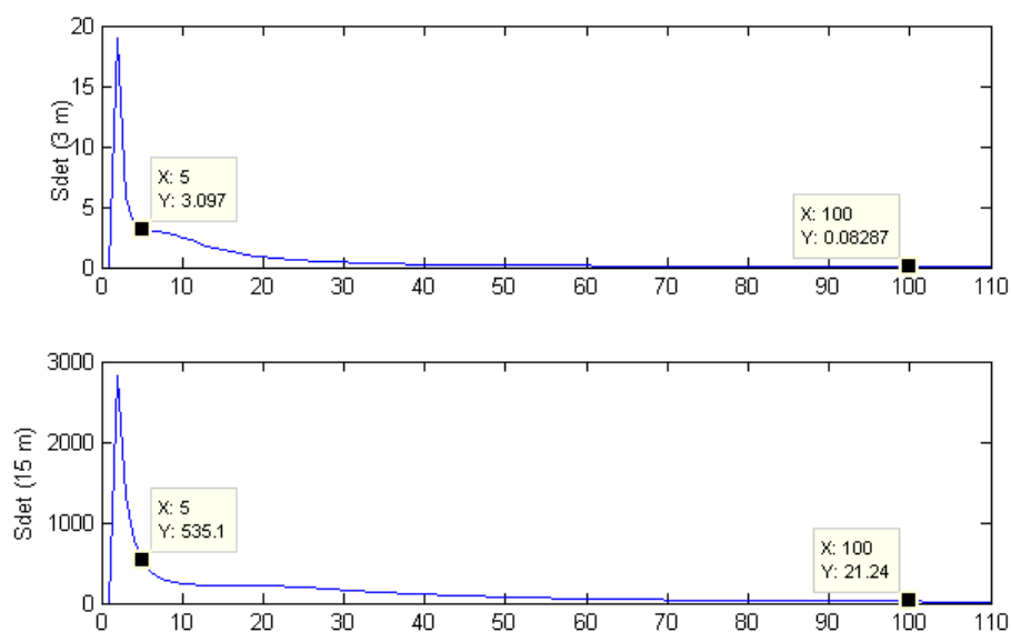
Figura 4-3. Medida de la incertidumbre durante las pruebas anteriores
