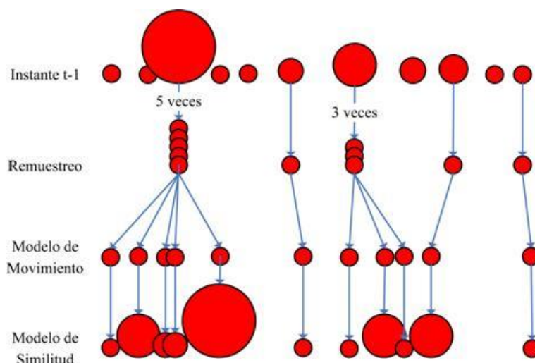
Figura 2-7. Pseudoprocedimiento del filtro de Partículas
