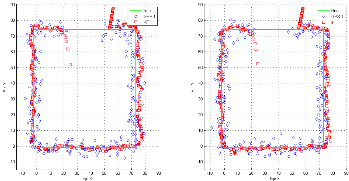
Figura 4-34. Cuadrado 2, GPS con w_g = 3\text{ m} , error del modelo: v = 0,5\text{ m} ,
