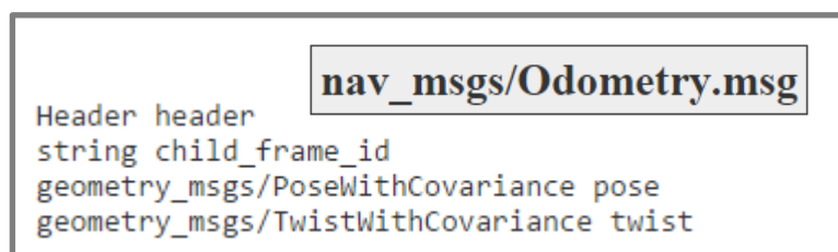
Figura 3-6. Mensaje Odometry en ROS del paquete nav_msgs
