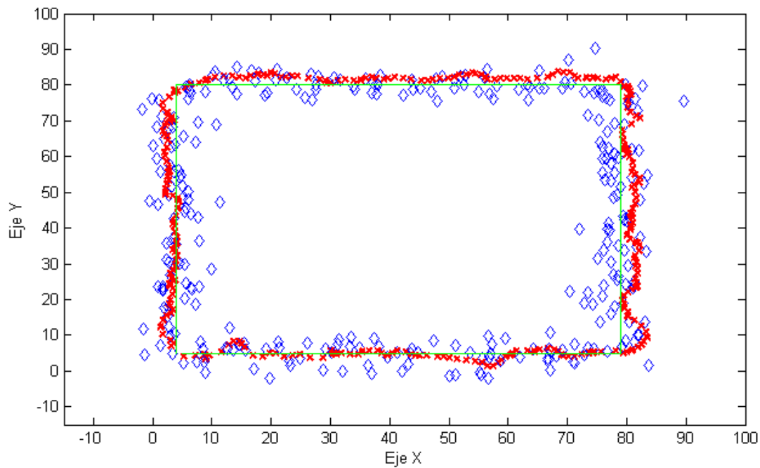
Figura 4-15. GPS con w_g = 3 \text{ m} , error del modelo: v = 0,5 \text{ m}
