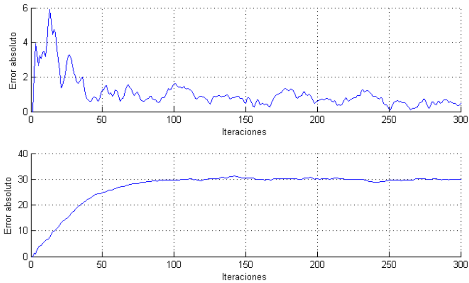
Figura 4-21. Lineal, Error en posición, a) Modelo rectilíneo, b) Modelo estático
