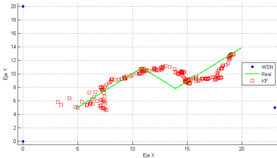
Figura 4-41. Zigzag, sensores con desviación w_r = 2,5 \text{ m} , modelo v = 0,1 \text{ m}
