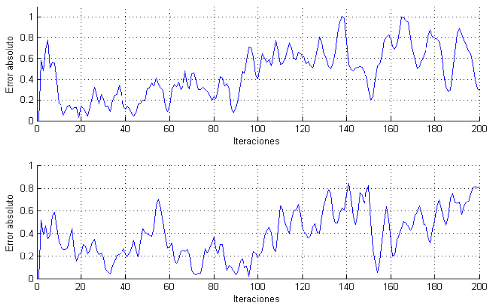
Figura 4-63. Zigzag con parada, errores: a) Modelo rectilíneo, b) Modelo estático
