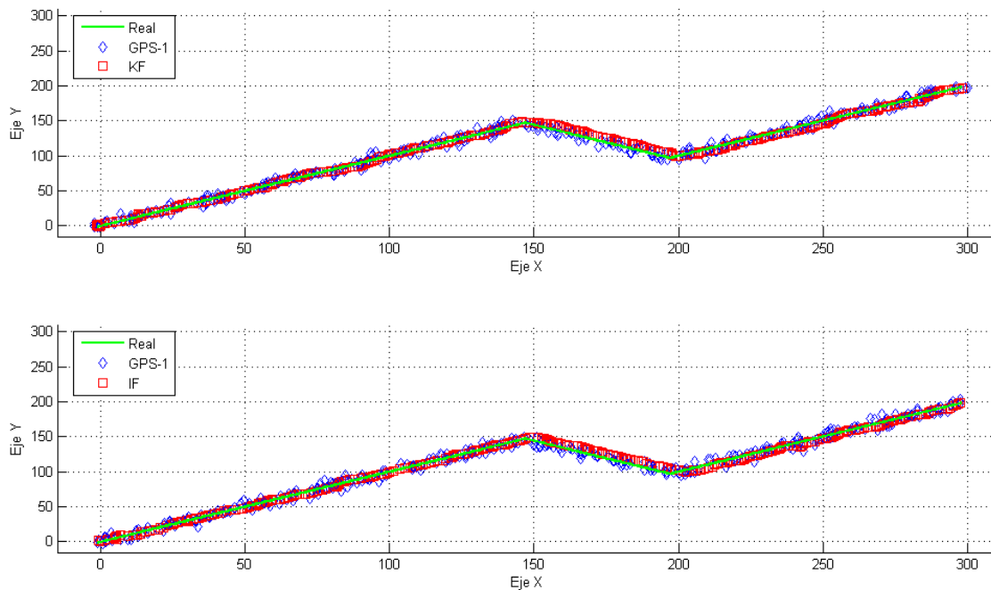
Figura 4-30. Zigzag, GPS con w_g = 3\text{ m} , error del modelo: v = 0,5\text{ m} , a) Filtro de Kalman, b) Filtro de Información
