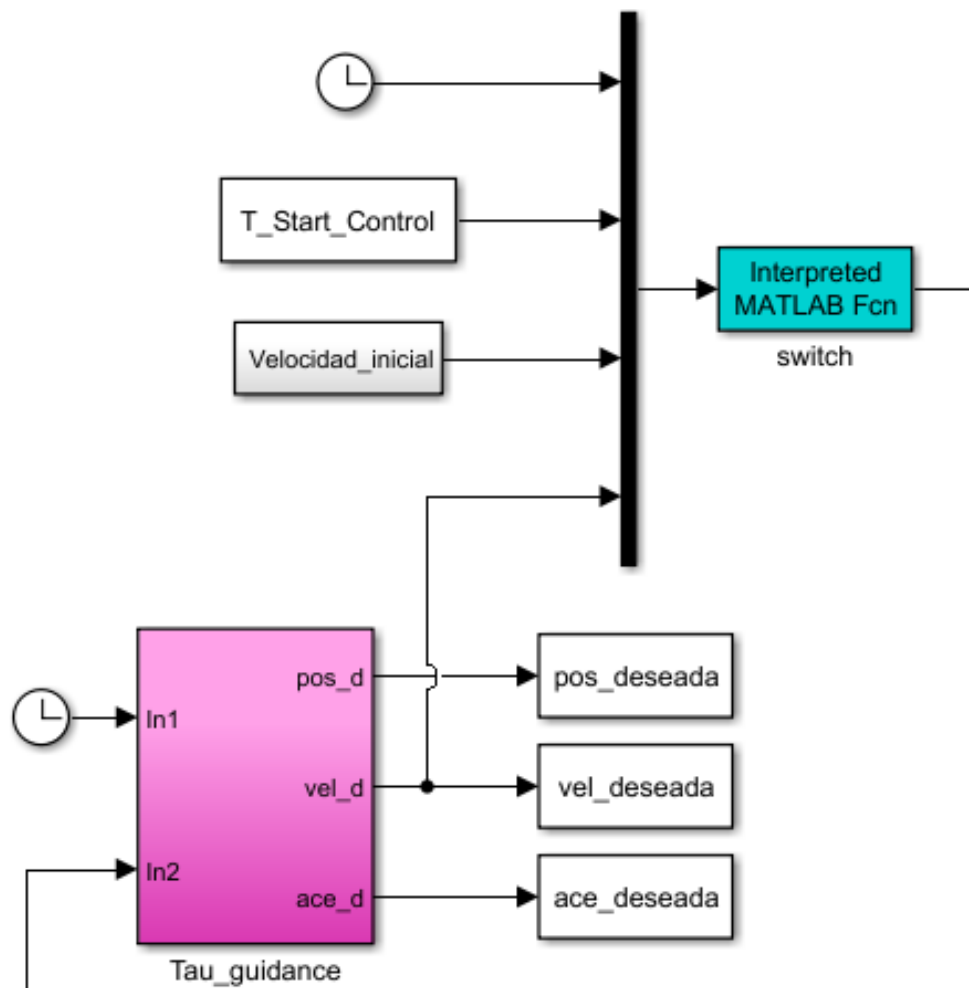
Figura 3:4 Bloque Switch y su entrada
