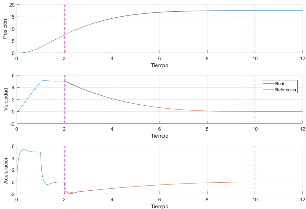
Figura 3:10 Simulación k=0.5
