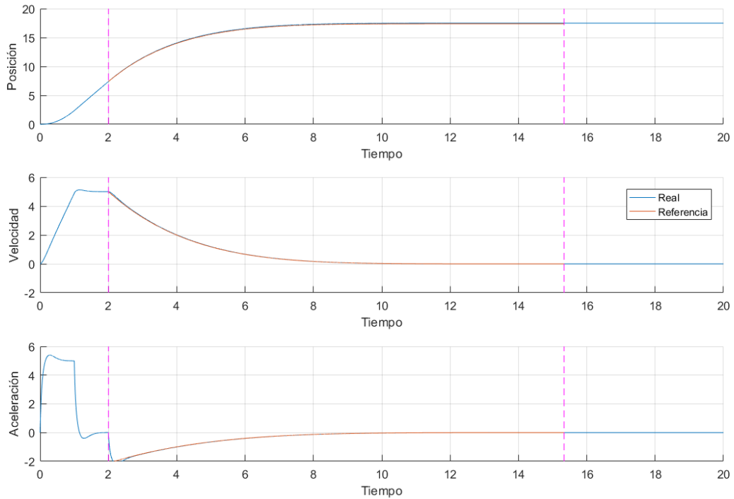
Figura 3:16 Simulación K=0.3
