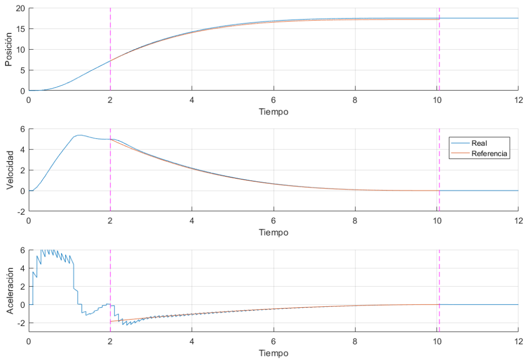
Figura 3:18 Simulación con tiempo de muestreo de 0.1 segundo
