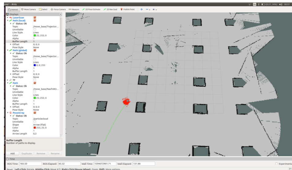
Figura 3.5. Desplazamiento del robot visualizado en Rviz (3).
