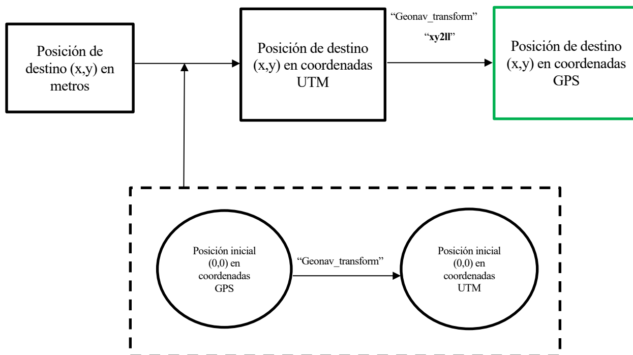
Figura 3.24. Obtención de las coordenadas del punto de destino (esquema).
