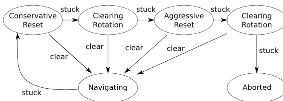
Figura 3.1. Esquema del paquete move_base. Obtenida de [16].
