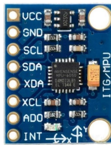
Figura 2.15 Controlador MPU.
