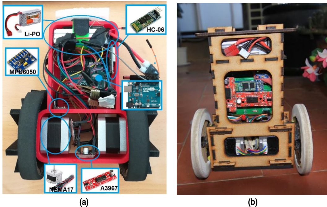
Figura 1.2 (a) Vehículo Jose A. Borja. (b) Vehículo Nicolás Cortés .
