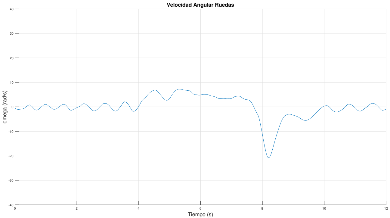
Figura 6.27 LQRI: Velocidad angular de las ruedas ante ensayo de fuerza creciente en parte superior del vehículo.
