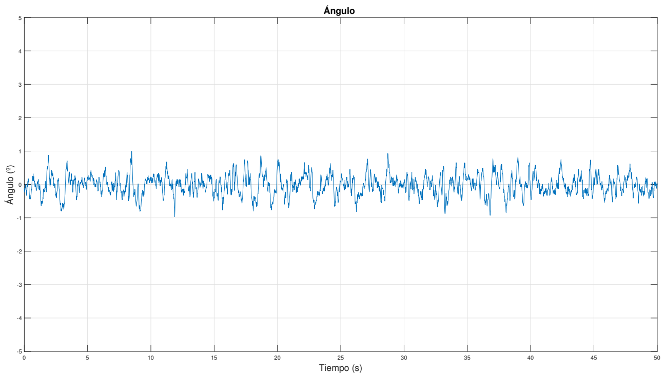
Figura 6.32 MPC: Ángulo ante ensayo de seguimiento de referencia nula en velocidad.
