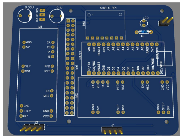
Figura 2.23 Vista 3D de la PCB.
