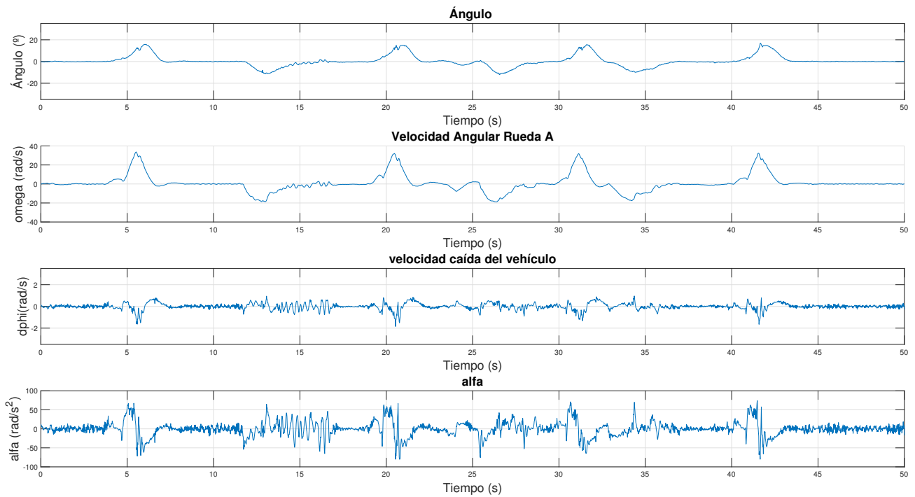
Figura 6.40 MPC: Variables ante ensayo en plano inclinado.
