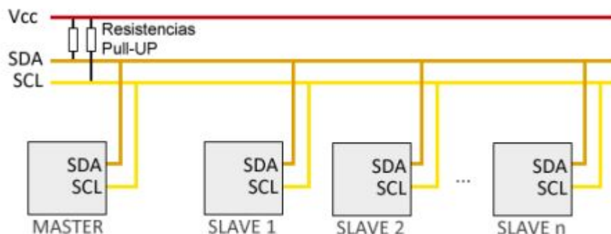
Figura 2.11 Esquema comunicación I2C.
