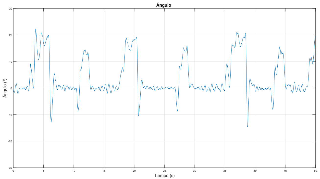
Figura 6.14 LQR: Ángulo ante ensayo en plano inclinado. Control remoto.
