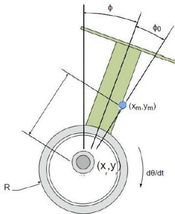
Figura 3.1 Esquema del modelo.
