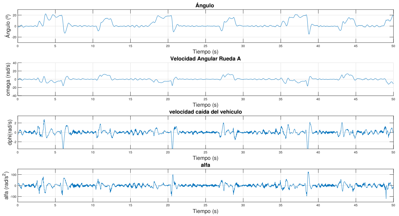
Figura 6.13 LQR: Variables ante ensayo en plano inclinado. Control remoto.
