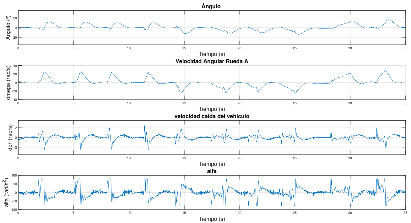
Figura 6.34 MPC: Variables ante ensayo de perturbaciones tipo pulso.
