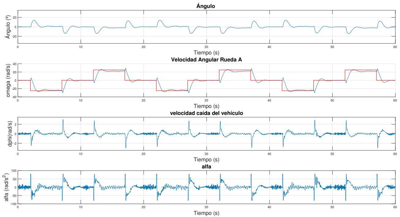
Figura 6.37 MPC: Variables ante ensayo de seguimiento de referencia cambiante en velocidad.
