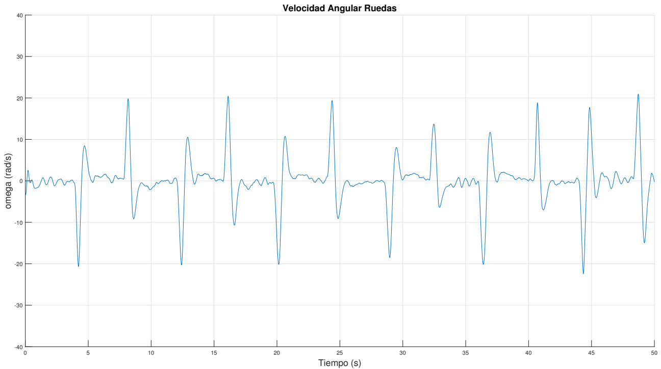
Figura 6.21 LQRI: Velocidad angular de las ruedas ante ensayo de perturbaciones tipo pulso.
