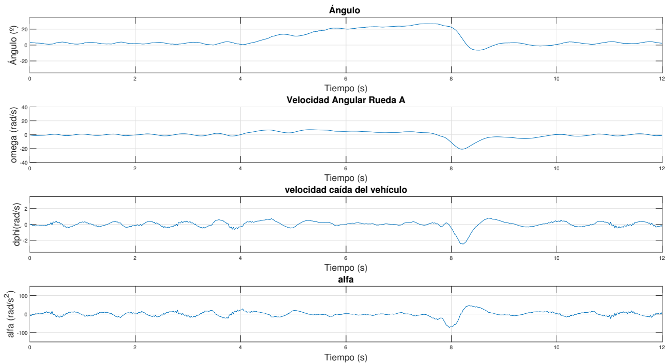
Figura 6.25 LQRI: Variables ante ensayo de fuerza creciente en parte superior del vehículo.
