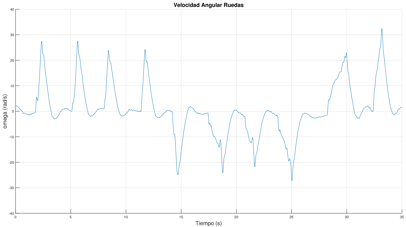
Figura 6.36 MPC: Velocidad angular de las ruedas ante ensayo de perturbaciones tipo pulso.
