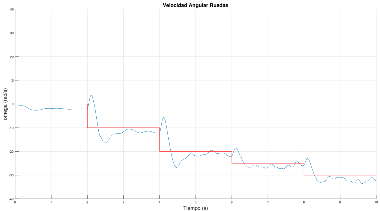
Figura 6.9 LQR: Velocidad angular de las ruedas ante ensayo de seguimiento de referencia cambiante en velocidad.
