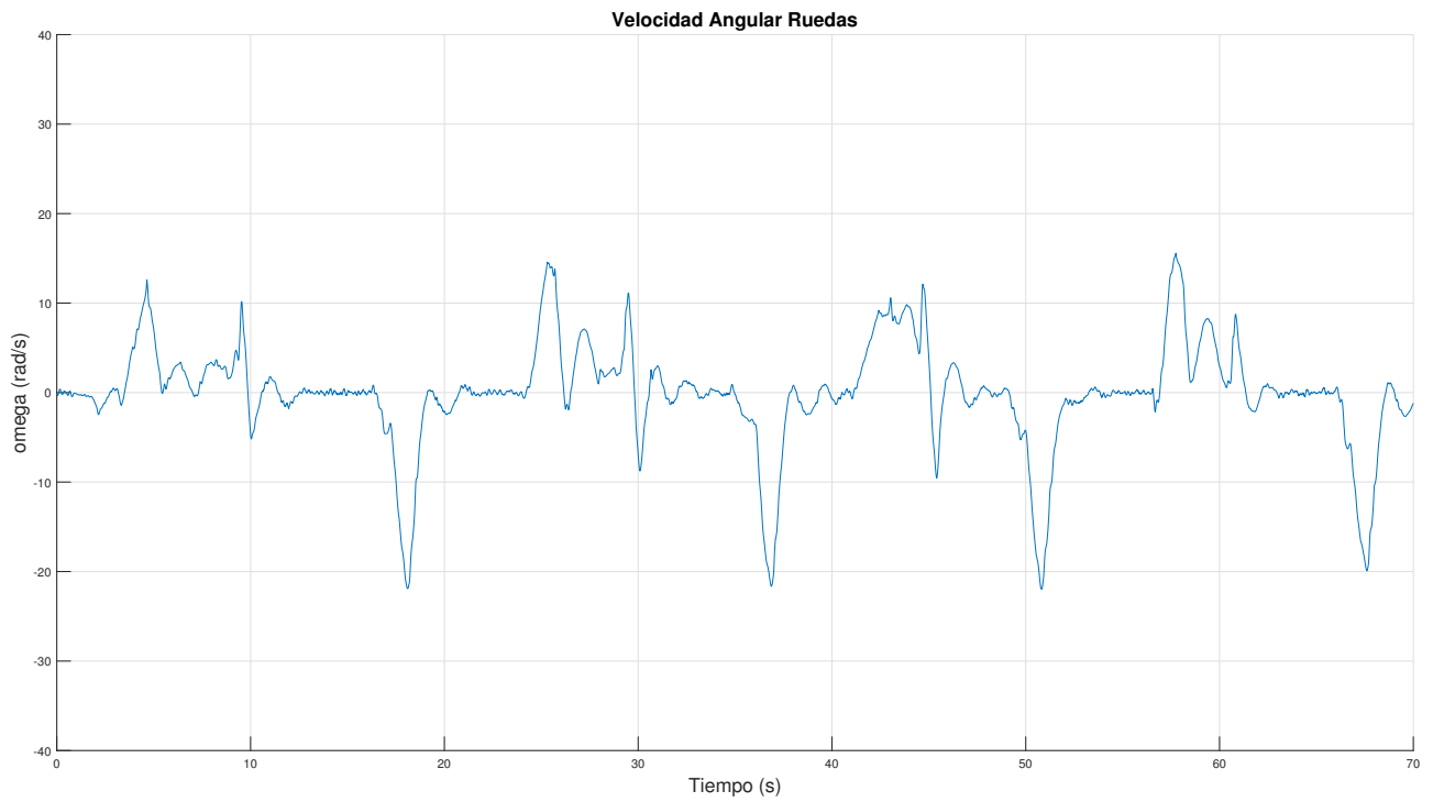
Figura 6.45 MPC: Velocidad angular de las ruedas ante ensayo en plano inclinado. Control remoto.
