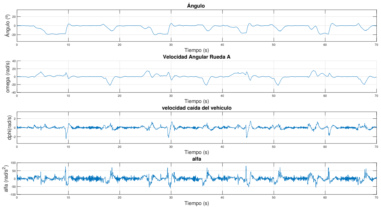
Figura 6.43 MPC: Variables ante ensayo en plano inclinado. Control remoto.
