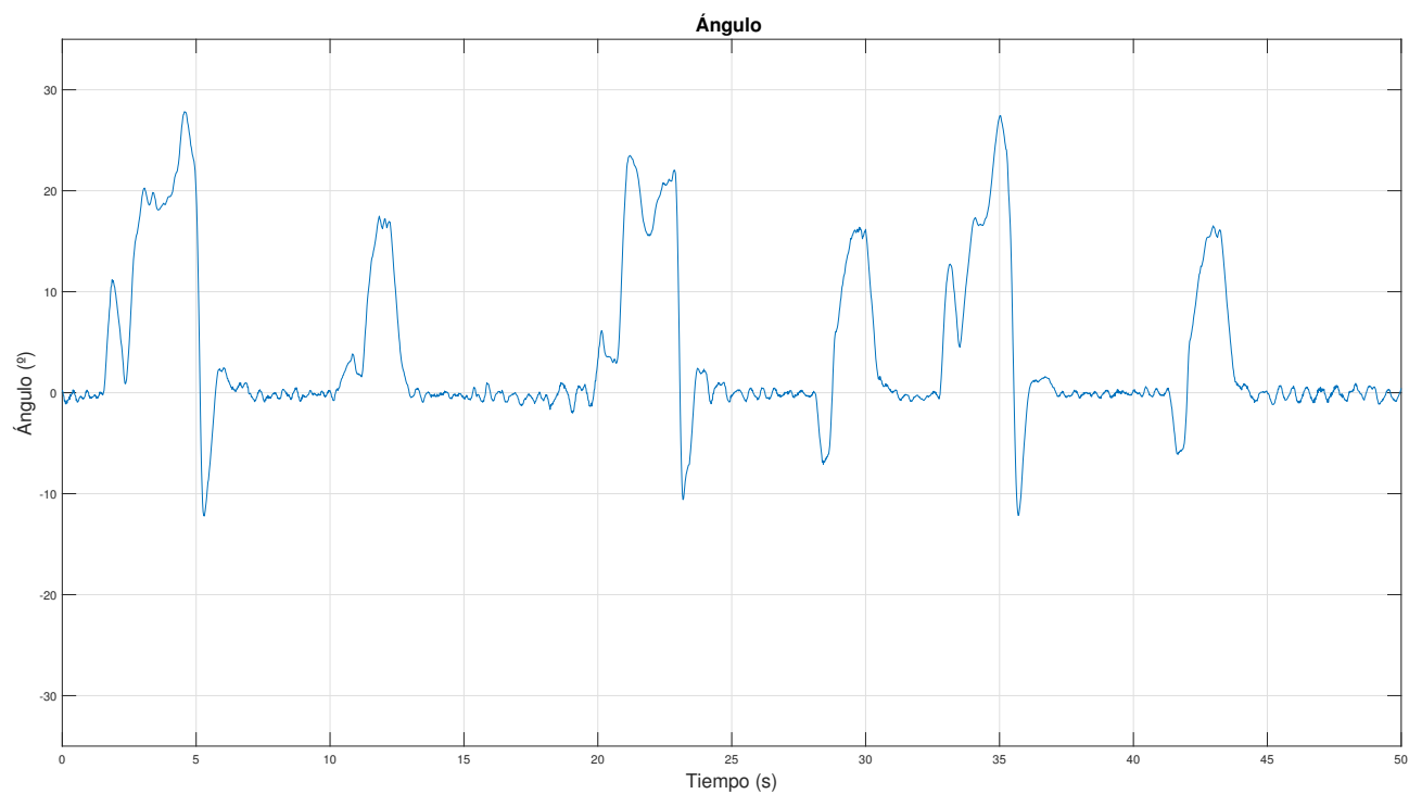
Figura 6.29 LQRI: Ángulo ante ensayo en plano inclinado. Control remoto.
