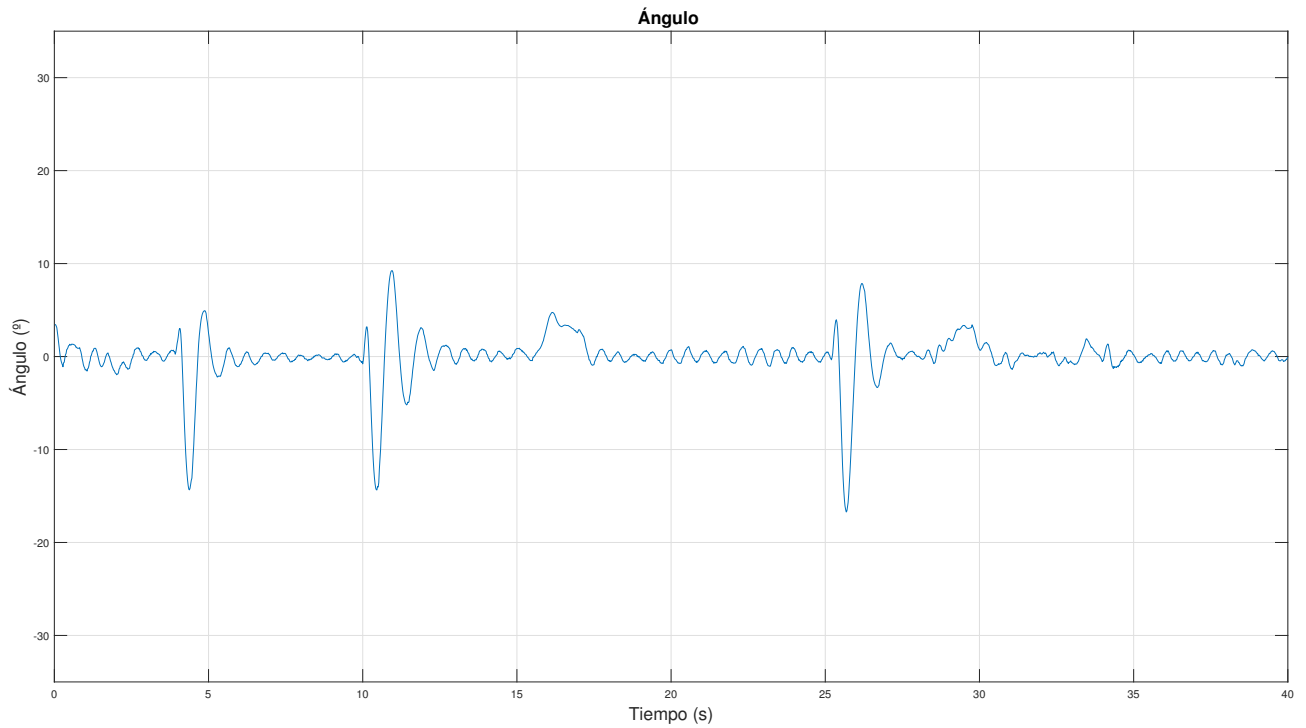
Figura 6.5 LQR: Ángulo ante ensayo de perturbaciones tipo pulso.
