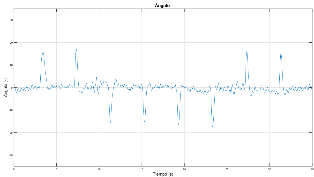
Figura 6.23 LQRI: Ángulo ante ensayo de seguimiento de referencia cambiante en velocidad.
