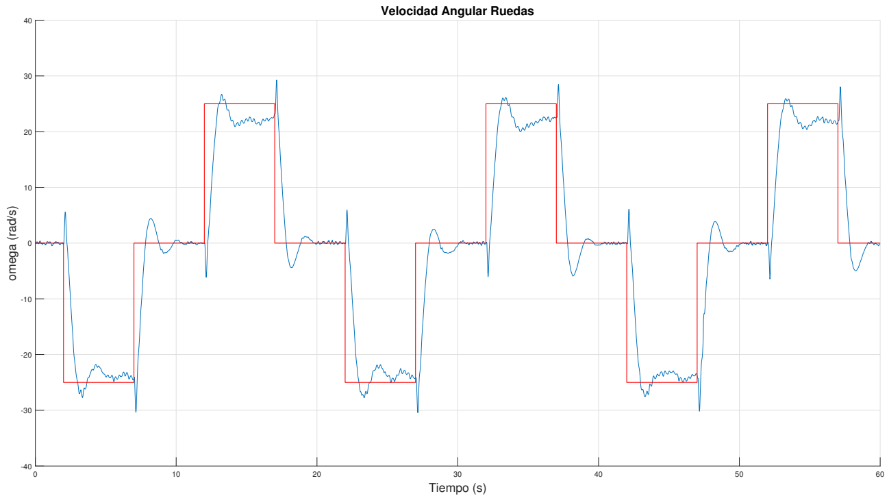
Figura 6.39 MPC: Velocidad angular de las ruedas ante ensayo de seguimiento de referencia cambiante en velocidad.
