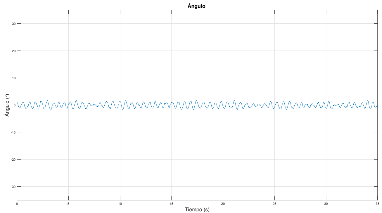
Figura 6.17 LQRI: Ángulo ante ensayo de seguimiento de referencia nula en velocidad.
