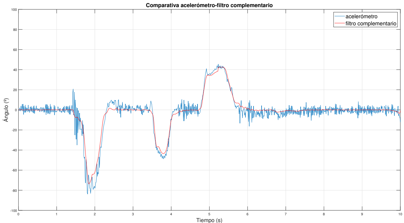
Figura 5.3 Comparativa del ángulo calculado mediante el acelerómetro y el filtro complementario.
