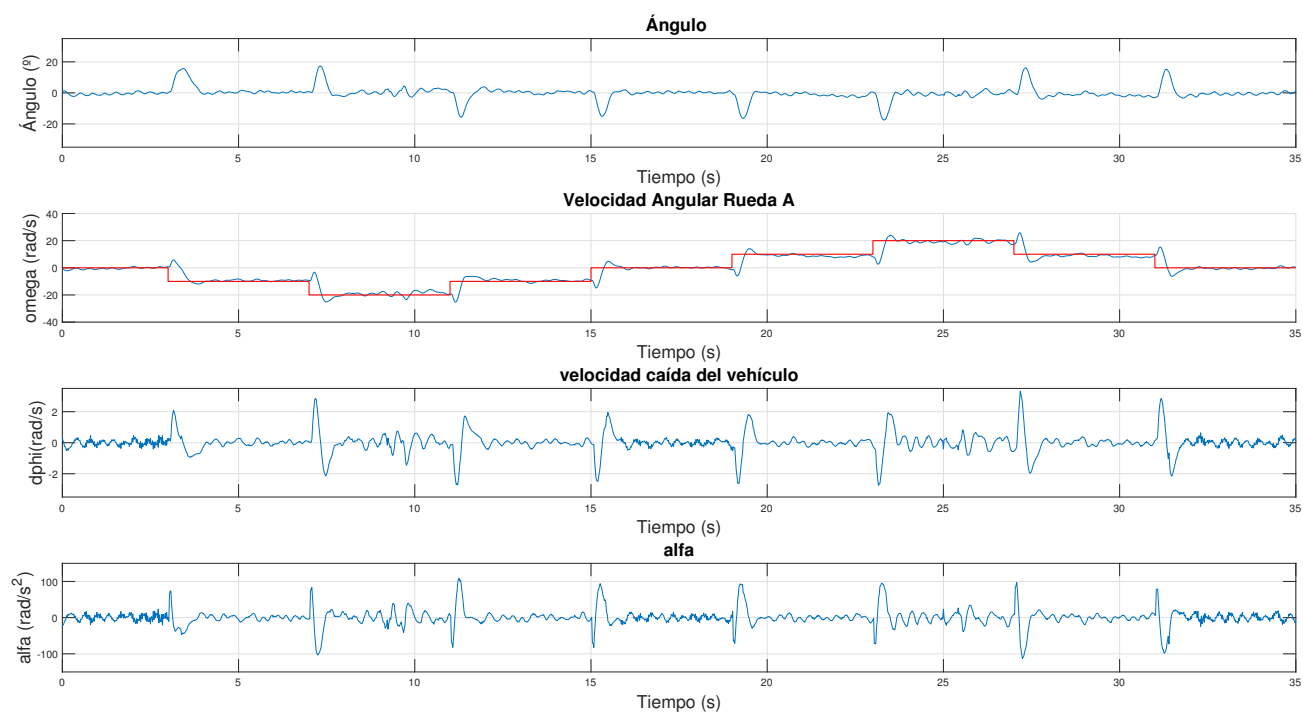
Figura 6.22 LQRI: Variables ante ensayo de seguimiento de referencia cambiante en velocidad.
