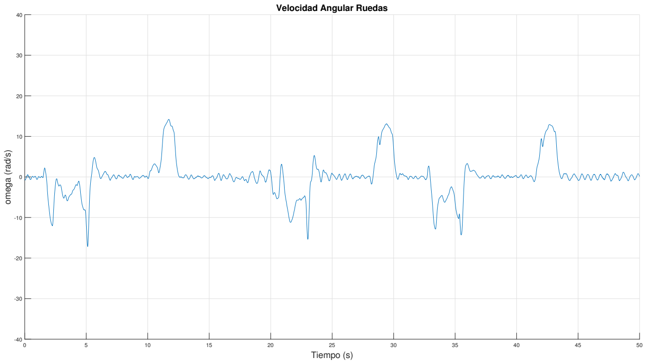
Figura 6.30 LQRI: Velocidad angular de las ruedas ante ensayo en plano inclinado. Control remoto.
