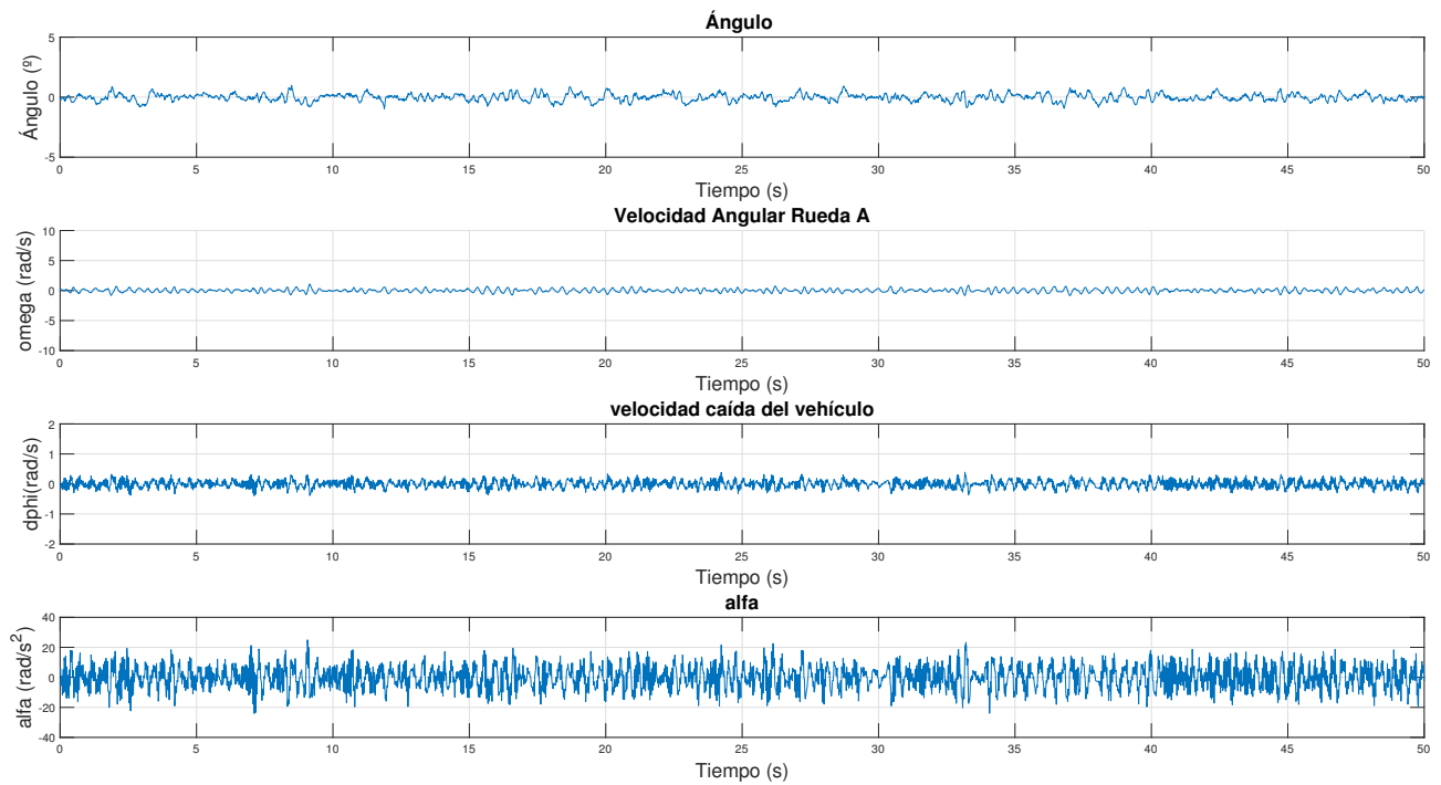
Figura 6.31 MPC: Variables ante ensayo de seguimiento de referencia nula en velocidad.
