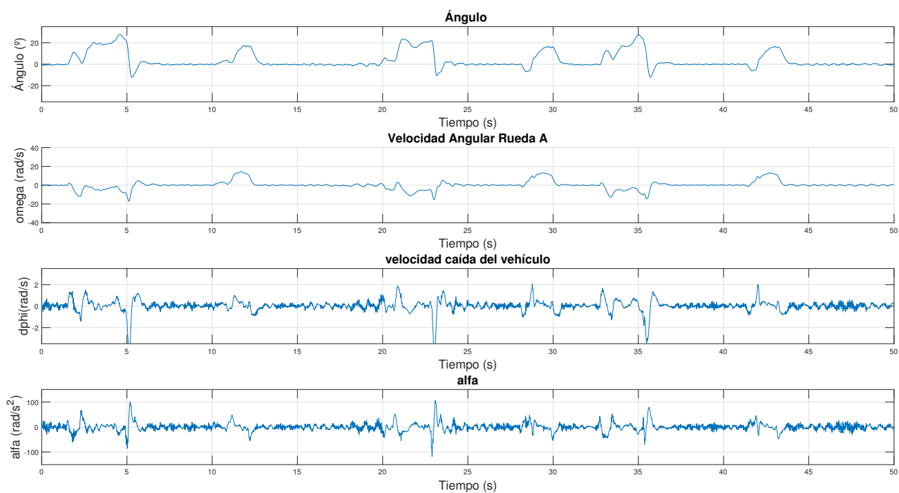
Figura 6.28 LQRI: Variables ante ensayo en plano inclinado. Control remoto.
