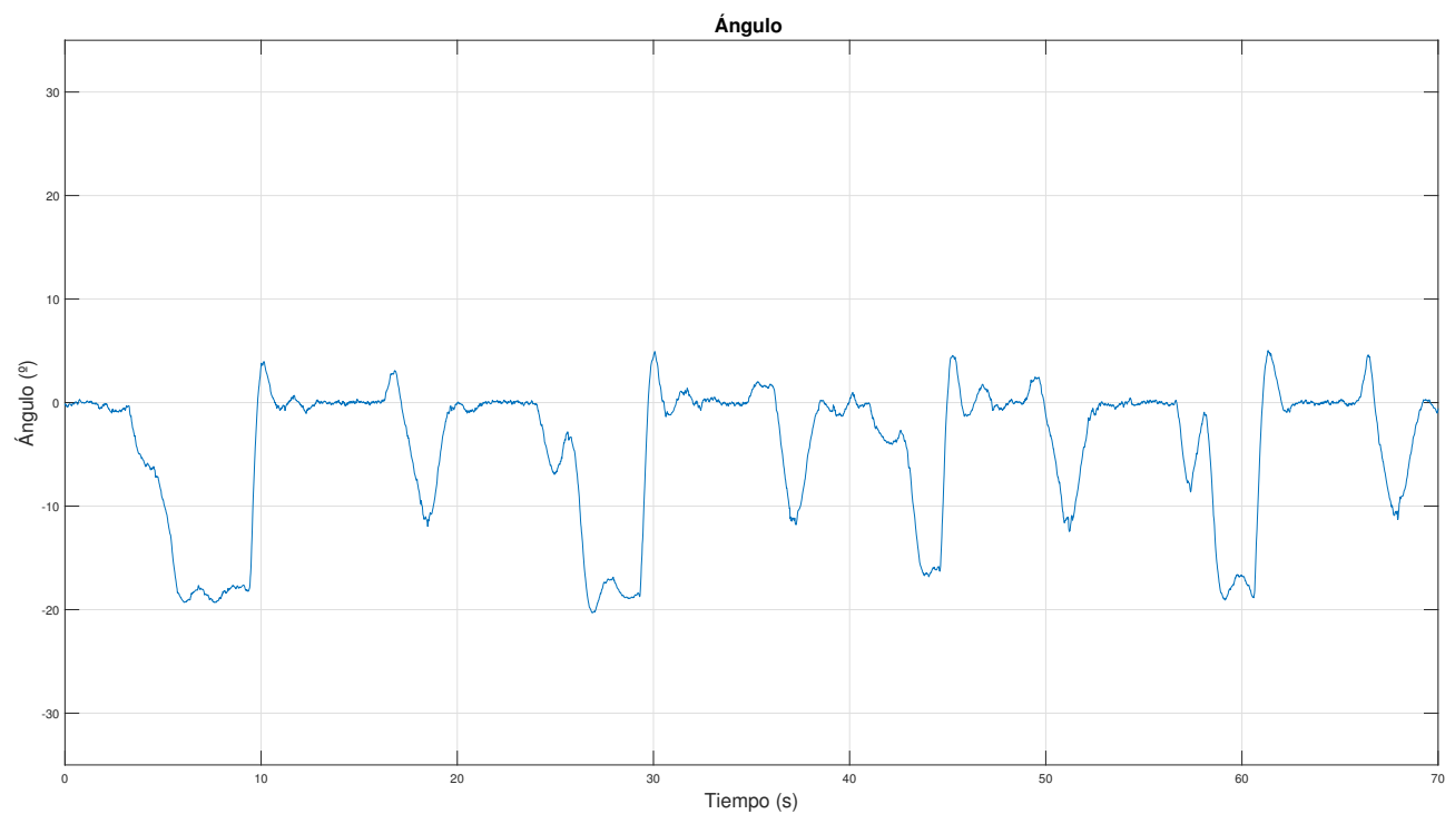
Figura 6.44 MPC: Ángulo ante ensayo en plano inclinado. Control remoto.
