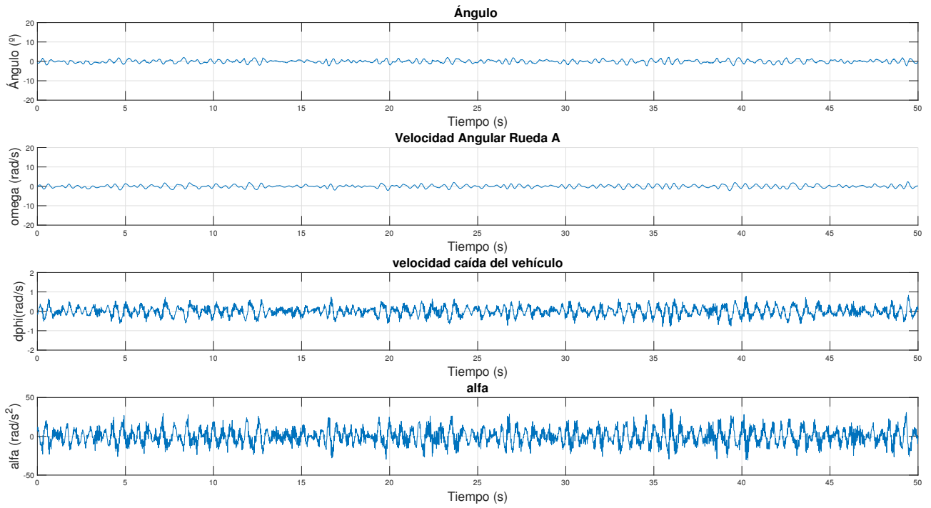
Figura 6.1 LQR: Variables ante ensayo de seguimiento de referencia nula en velocidad.
