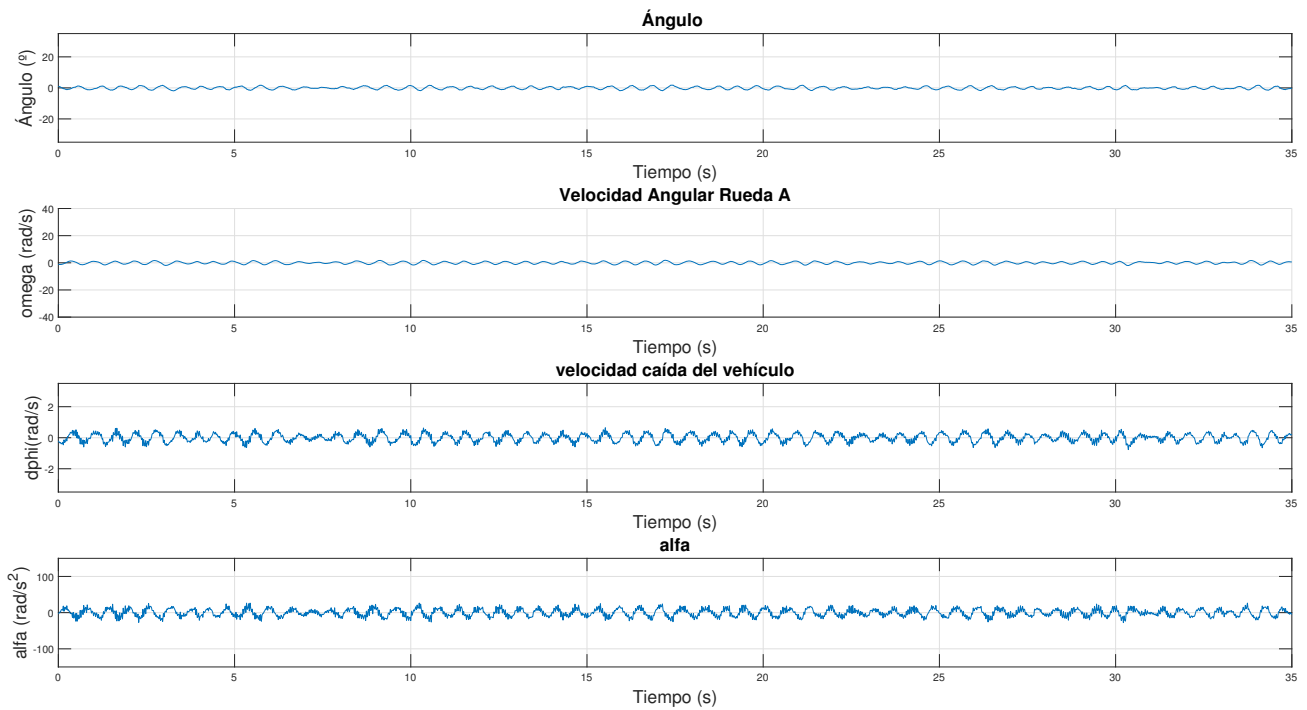
Figura 6.16 LQRI: Variables ante ensayo de seguimiento de referencia nula en velocidad.
