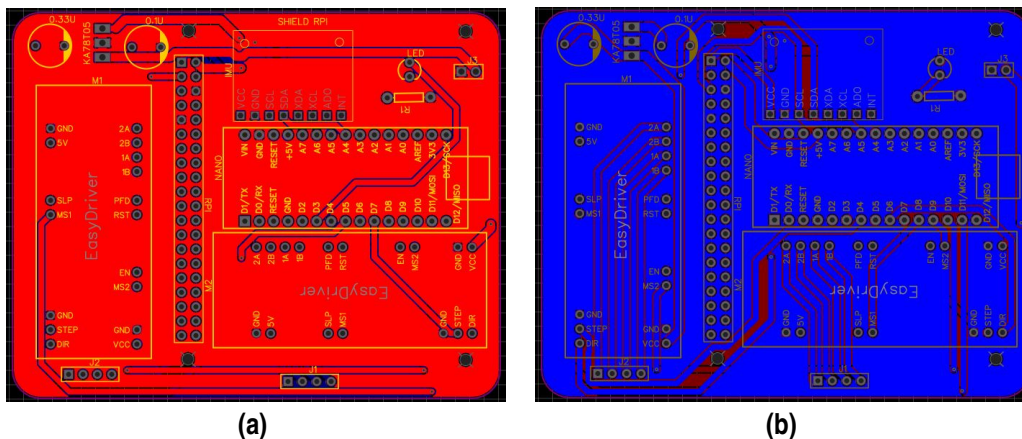
Figura 2.24 (a) Vista capa superior PCB. (b) Vista capa inferior PCB .
