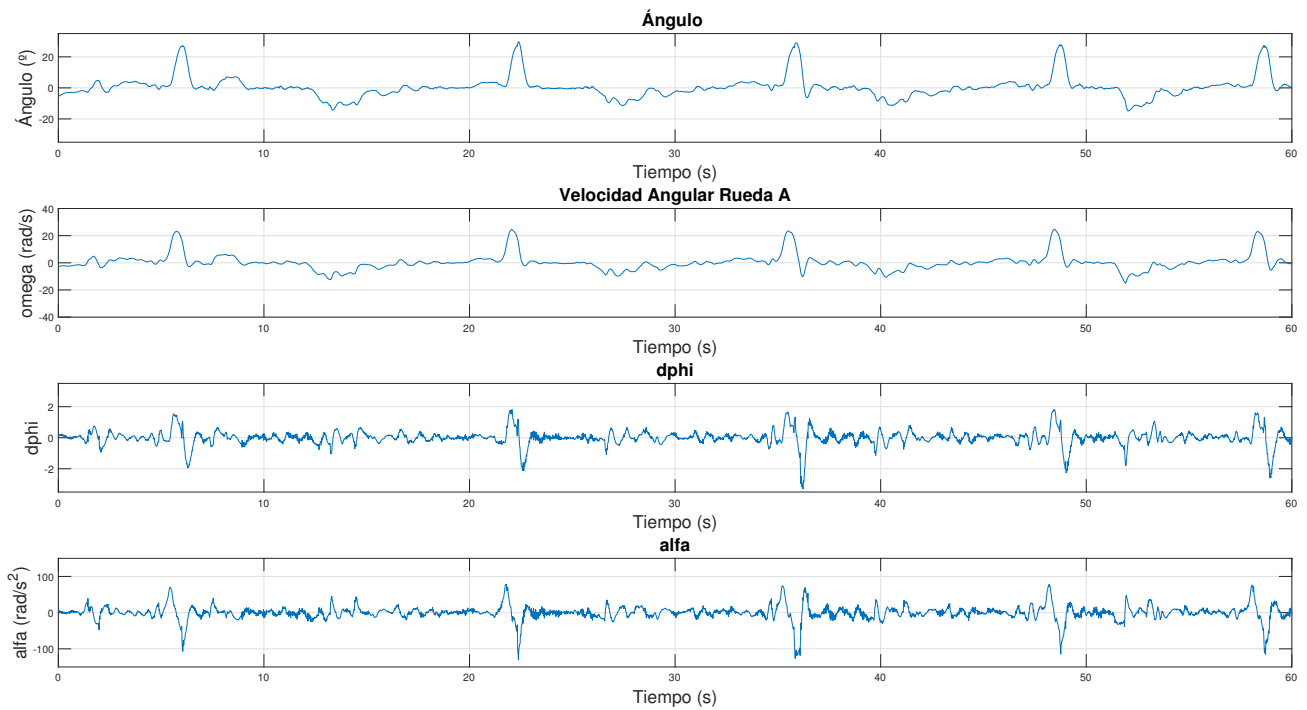
Figura 6.10 LQR: Variables ante ensayo en plano inclinado.
