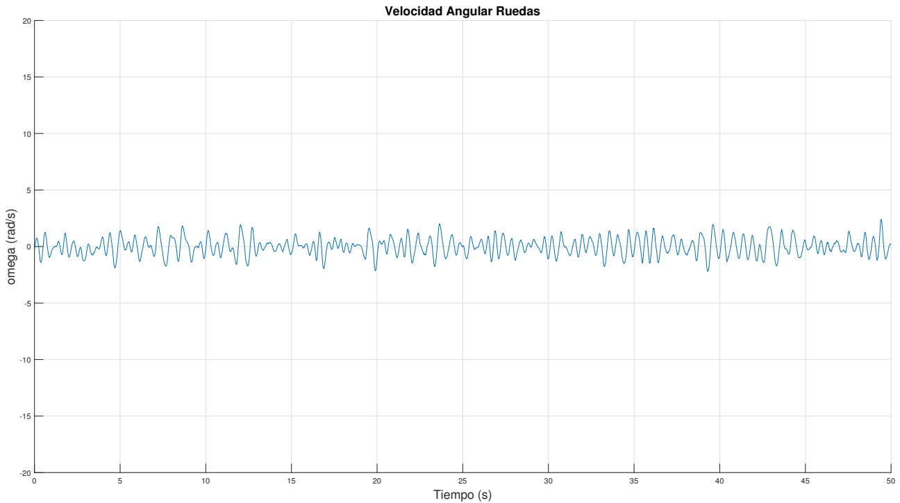
Figura 6.3 LQR: Velocidad angular de las ruedas ante ensayo de seguimiento de referencia nula en velocidad.
