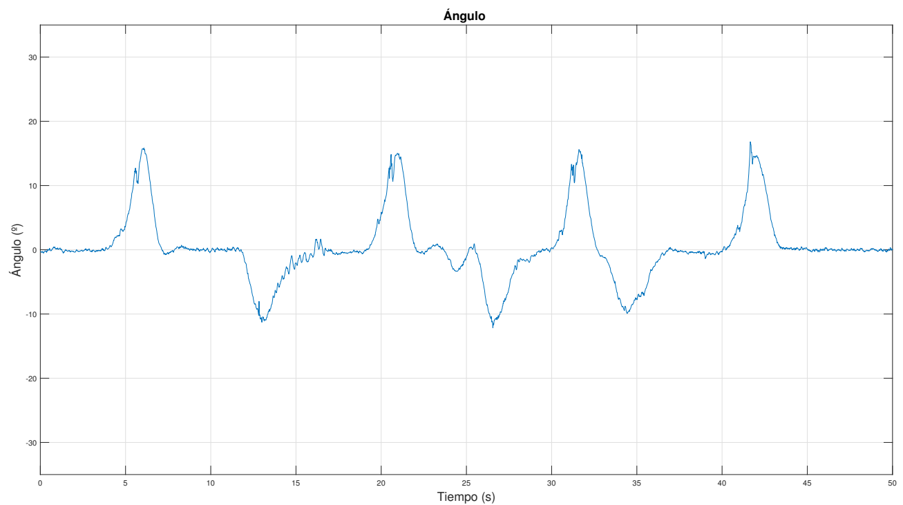
Figura 6.41 MPC: Ángulo ante ensayo en plano inclinado.
