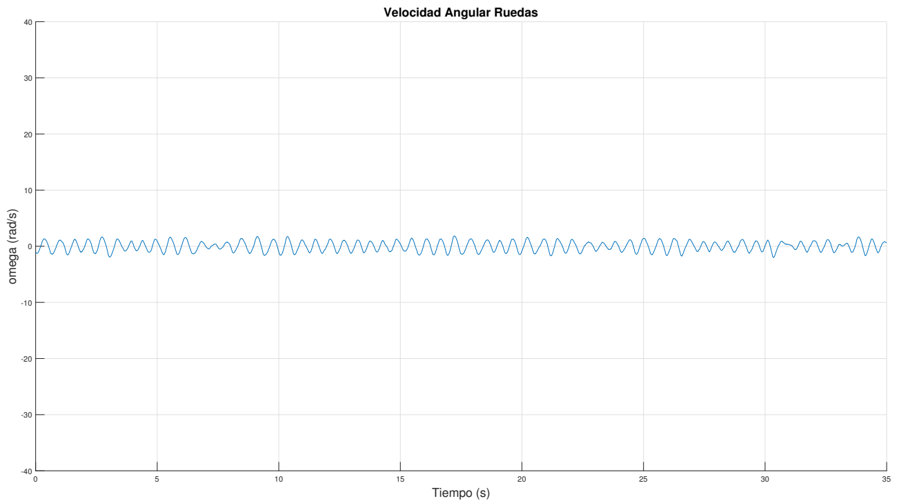
Figura 6.18 LQRI: Velocidad angular de las ruedas ante ensayo de seguimiento de referencia nula en velocidad.
