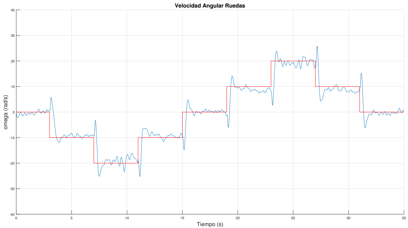
Figura 6.24 LQRI: Velocidad angular de las ruedas ante ensayo de seguimiento de referencia cambiante en velocidad.
