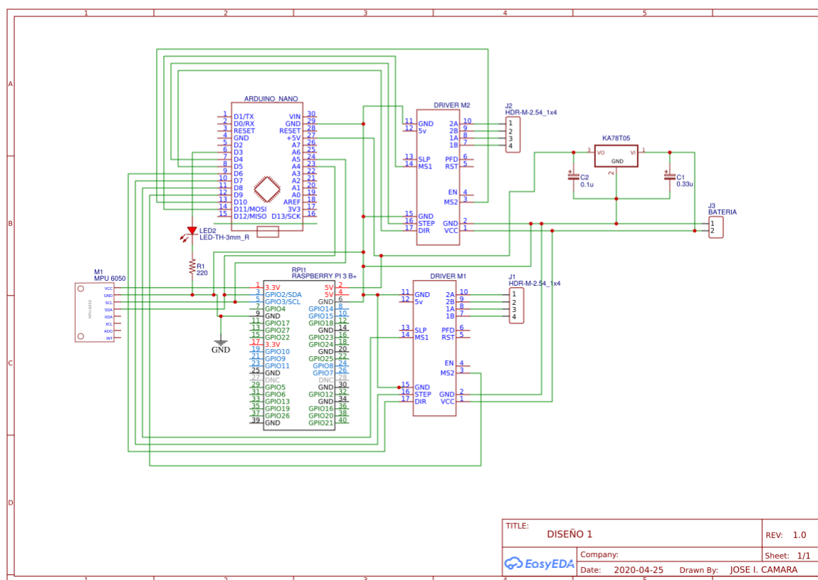
Figura 2.25 Esquema de conexiones.
