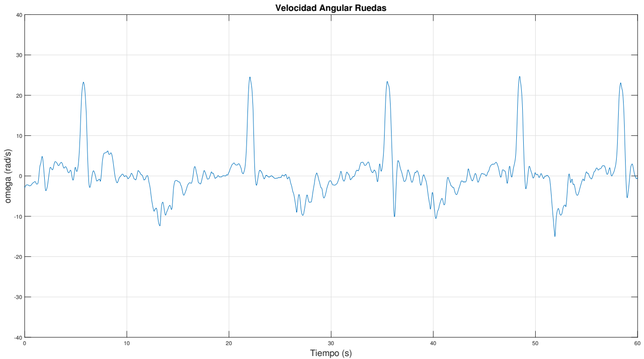
Figura 6.12 LQR: Velocidad angular de las ruedas ante ensayo en plano inclinado.
