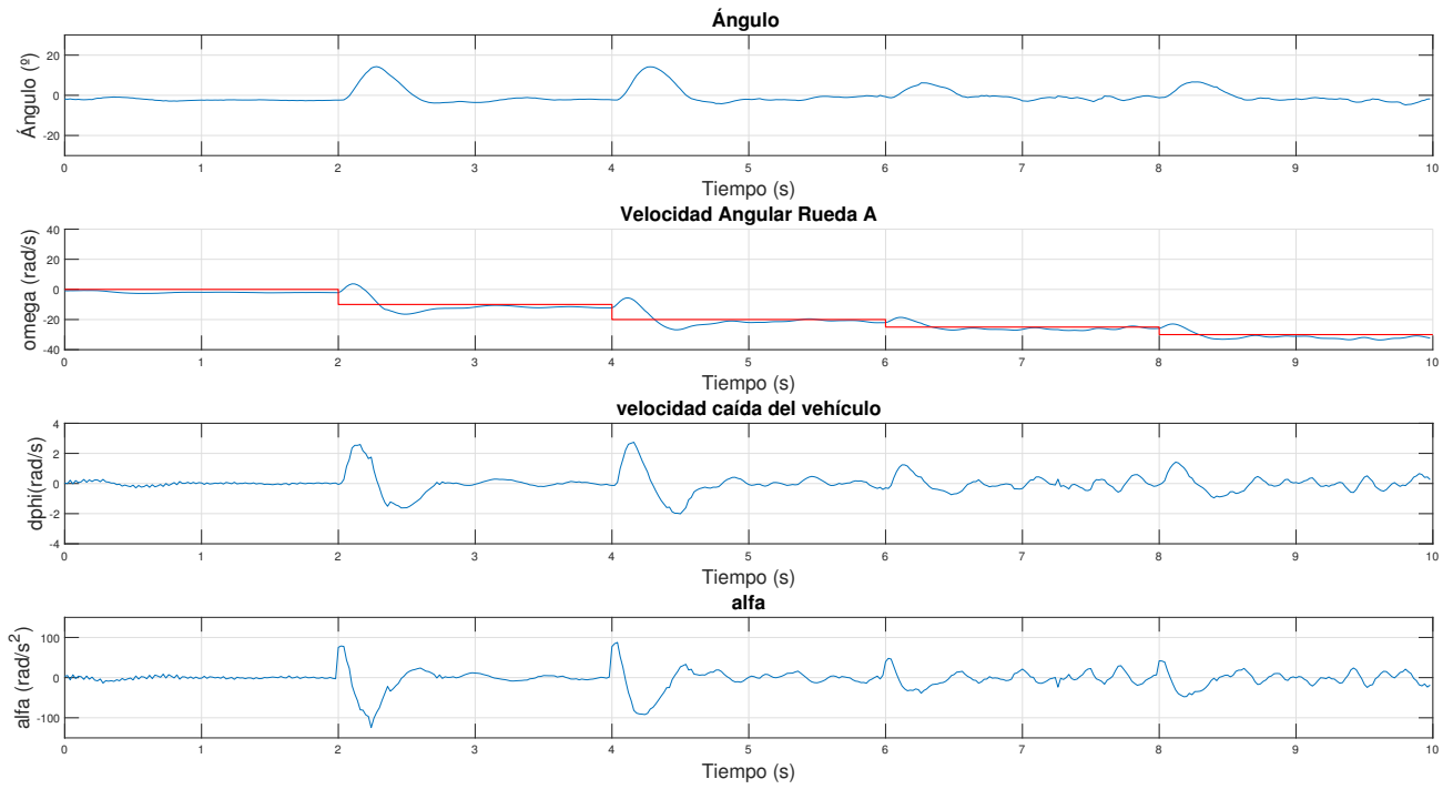
Figura 6.7 LQR: Variables ante ensayo de seguimiento de referencia cambiante en velocidad.
