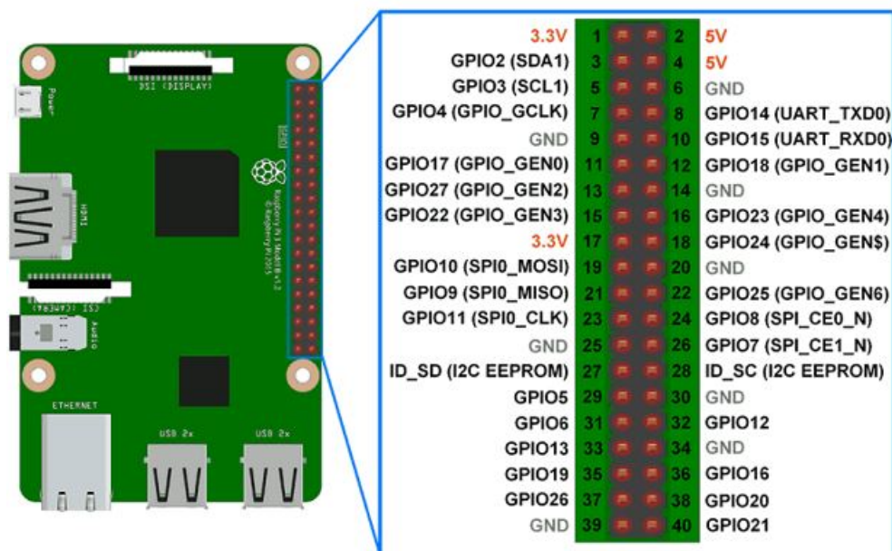
Figura 2.12 Distribución GPIO.
