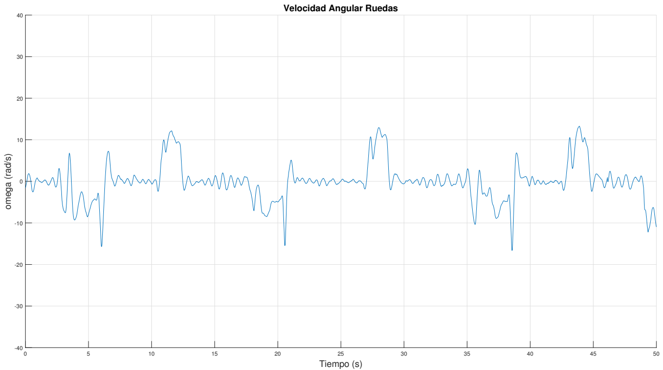
Figura 6.15 LQR: Velocidad angular de las ruedas ante ensayo en plano inclinado. Control remoto.
