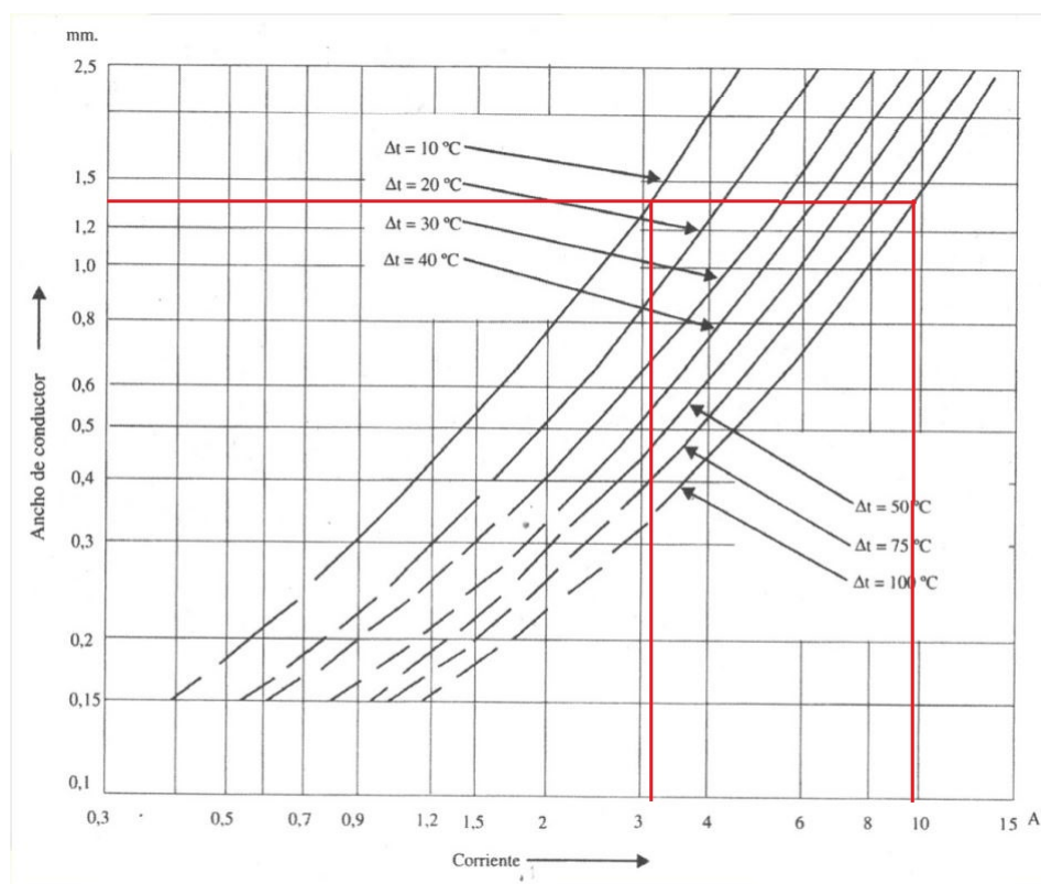
Figura 2.22 Elección del ancho de pista.
