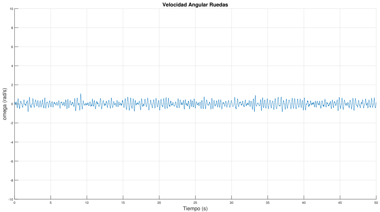
Figura 6.33 MPC: Velocidad angular de las ruedas ante ensayo de seguimiento de referencia nula en velocidad.
