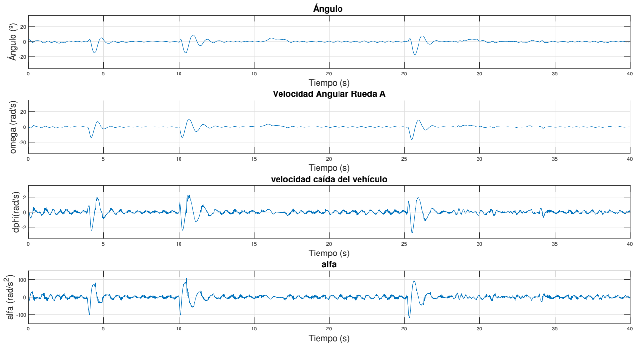
Figura 6.4 LQR: Variables ante ensayo de perturbaciones tipo pulso.
