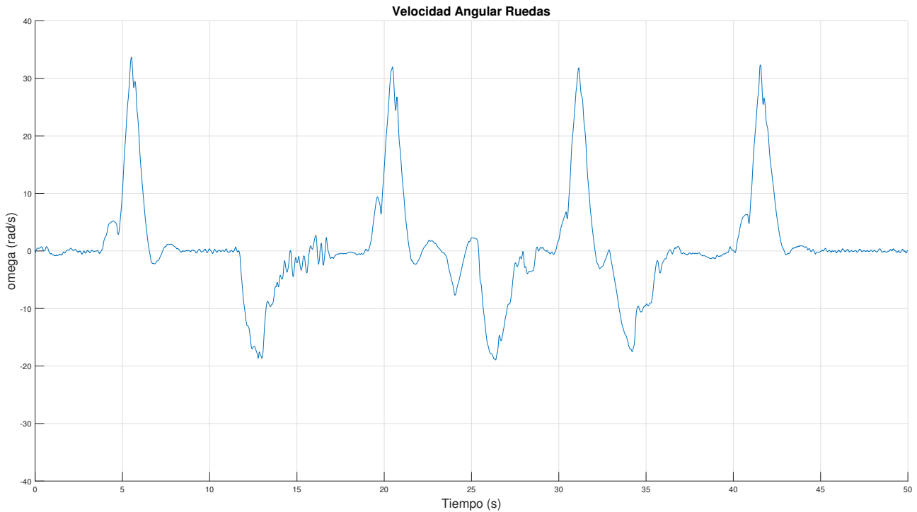
Figura 6.42 MPC: Velocidad angular de las ruedas ante ensayo en plano inclinado.
