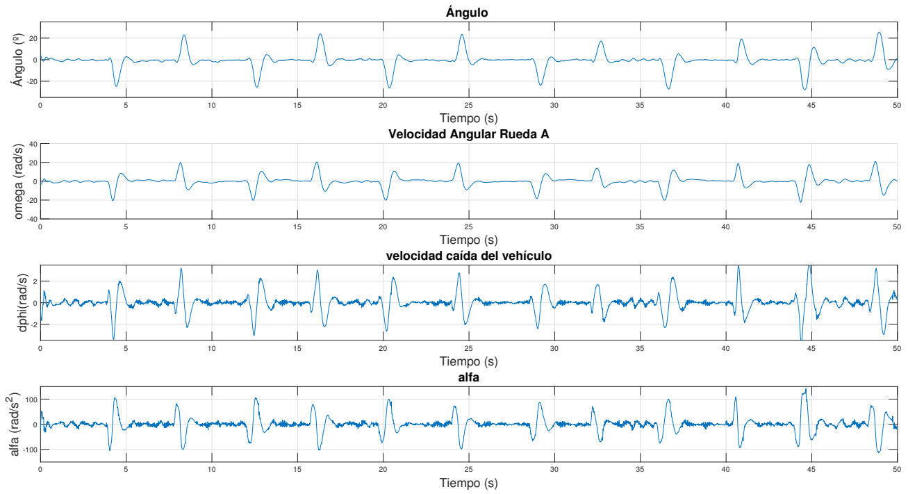
Figura 6.19 LQRI: Variables ante ensayo de perturbaciones tipo pulso.
