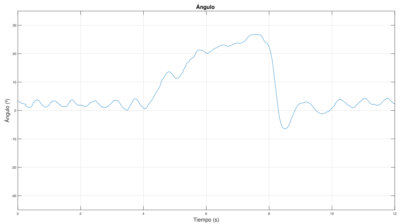
Figura 6.26 LQRI: Ángulo ante ensayo de fuerza creciente en parte superior del vehículo.
