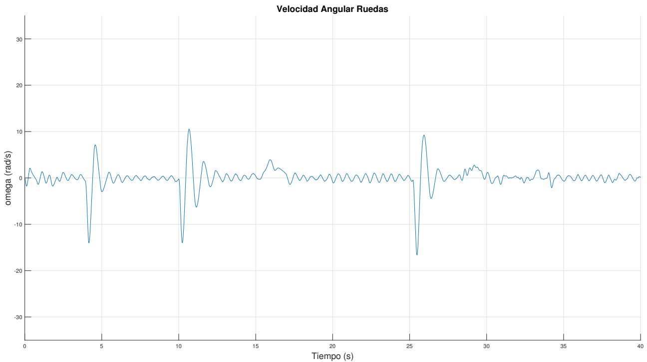
Figura 6.6 LQR: Velocidad angular de las ruedas ante ensayo de perturbaciones tipo pulso.
