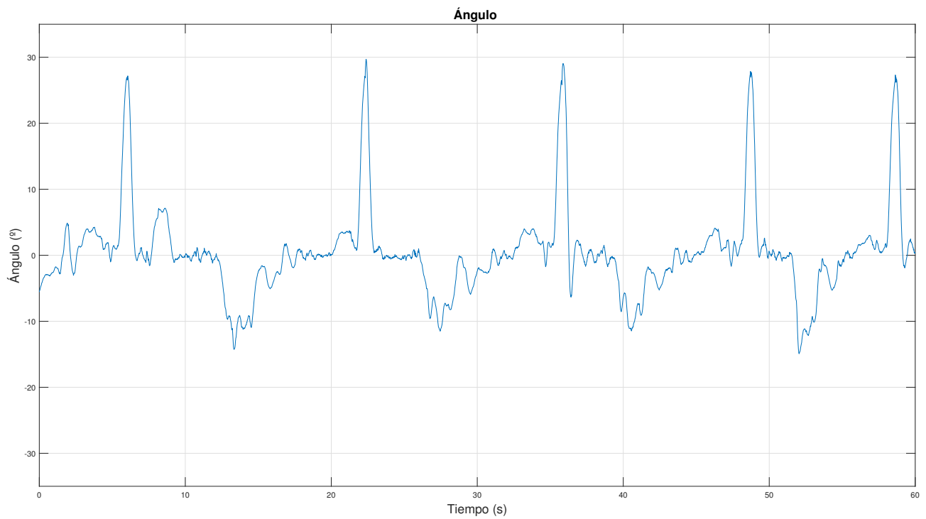
Figura 6.11 LQR: Ángulo ante ensayo en plano inclinado.
