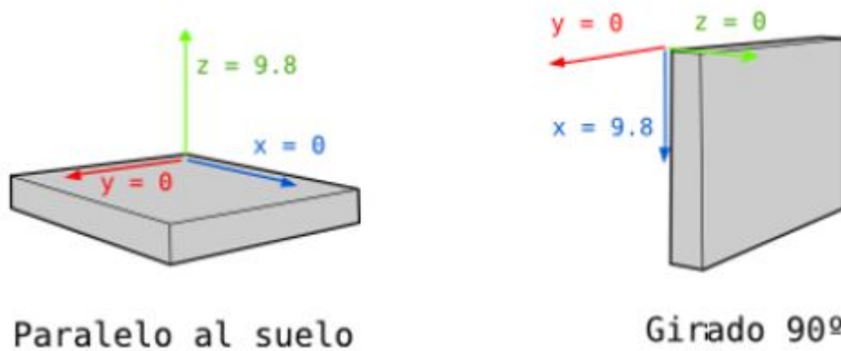
Figura 2.17 Disposición sensor MPU.
