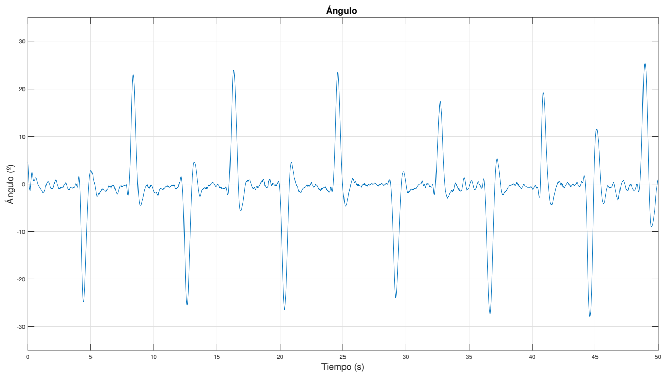
Figura 6.20 LQRI: Ángulo ante ensayo de perturbaciones tipo pulso.
