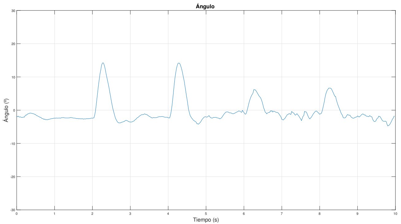
Figura 6.8 LQR: Ángulo ante ensayo de seguimiento de referencia cambiante en velocidad.
