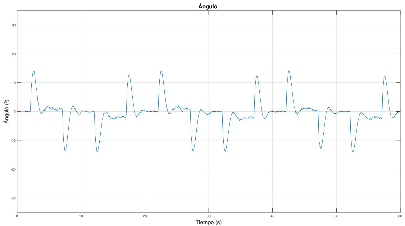
Figura 6.38 MPC: Ángulo ante ensayo de seguimiento de referencia cambiante en velocidad.
