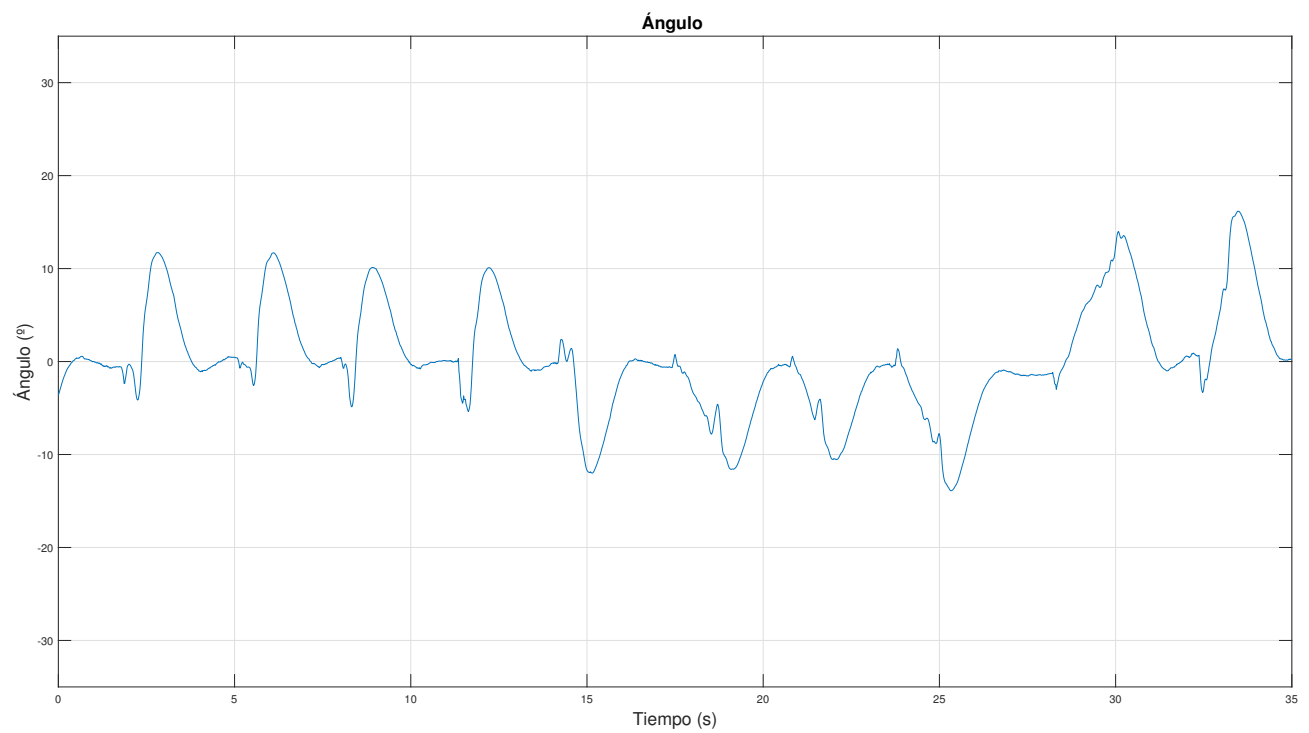
Figura 6.35 MPC: Ángulo ante ensayo de perturbaciones tipo pulso.
