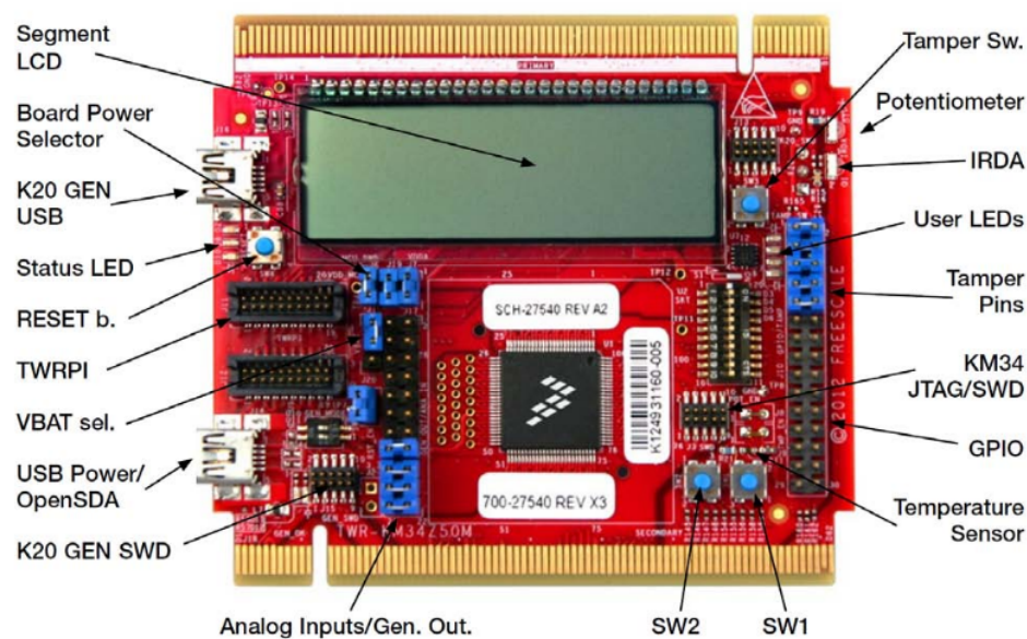
Figura 3.1 Frontal del módulo TWR-KM34Z50M (Dispositivos TWRPI no mostrados).
