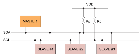
Figura 5.3 Estructura I2C.
