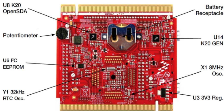
Figura 3.2 Trasera del módulo TWR-KM34Z50M.
