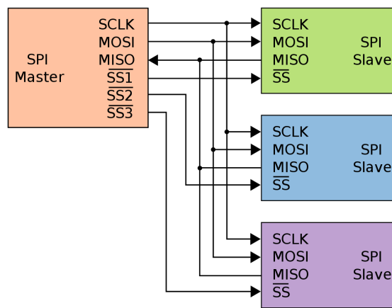
Figura 5.4 Estructura SPI.
