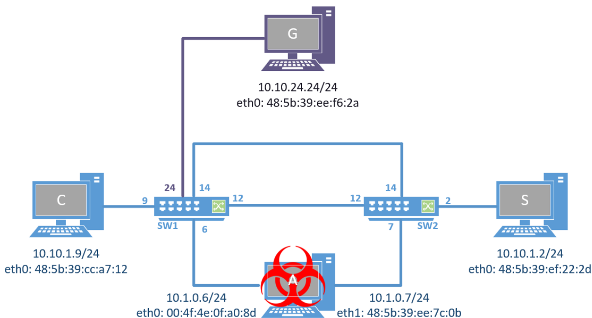
Figura 3-6. Escenario del ataque 7.2.2
