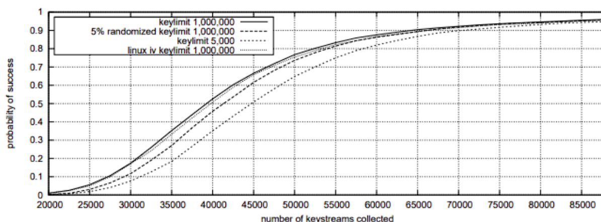
Figura 2-33. Relación entre IVs capturados y probabilidad de éxito del ataque PTW [72]
