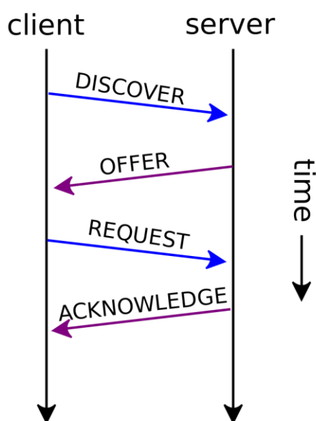
Figura 2-30. Proceso típico de asignación de direcciones con DHCP [56]
