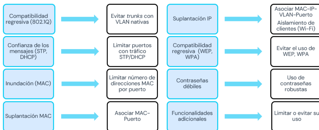
Figura 6-7. Metodologías de ataques y sus mecanismos de defensa L2
