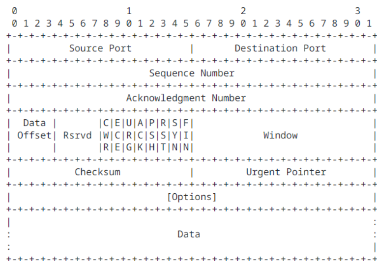
Figura 2-18. Formato de la cabecera TCP
