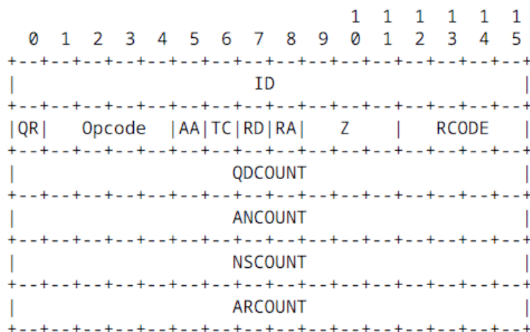
Figura 2-24. Formato del mensaje y de la cabecera DNS
