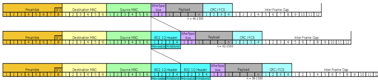
Figura 2-9. Comparativa entre tramas Ethernet sin etiqueta, con etiqueta y doble etiqueta [12]
