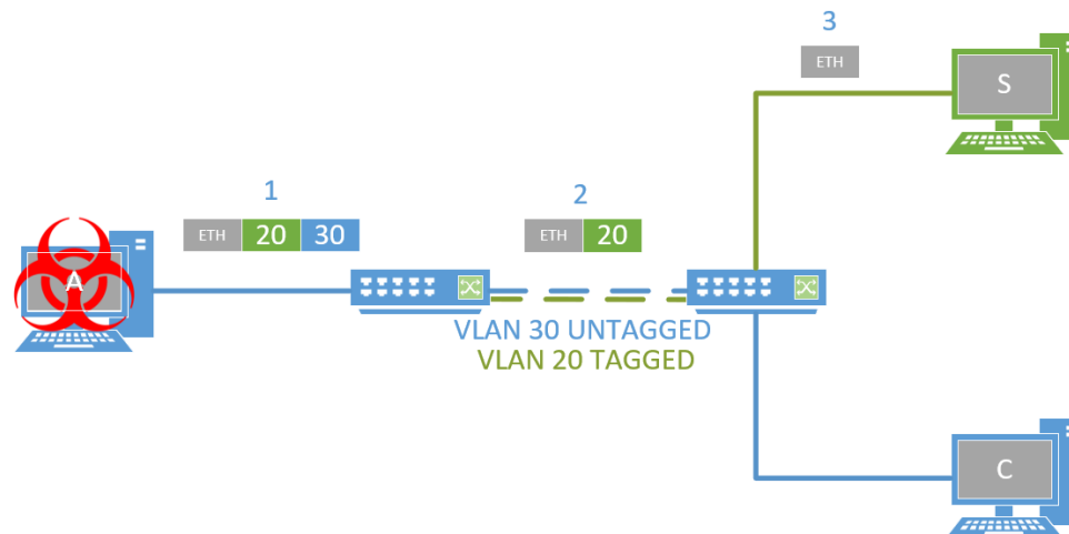
Figura 2-10. Ejemplo de envío de una trama Ethernet que realiza un salto de VLAN
