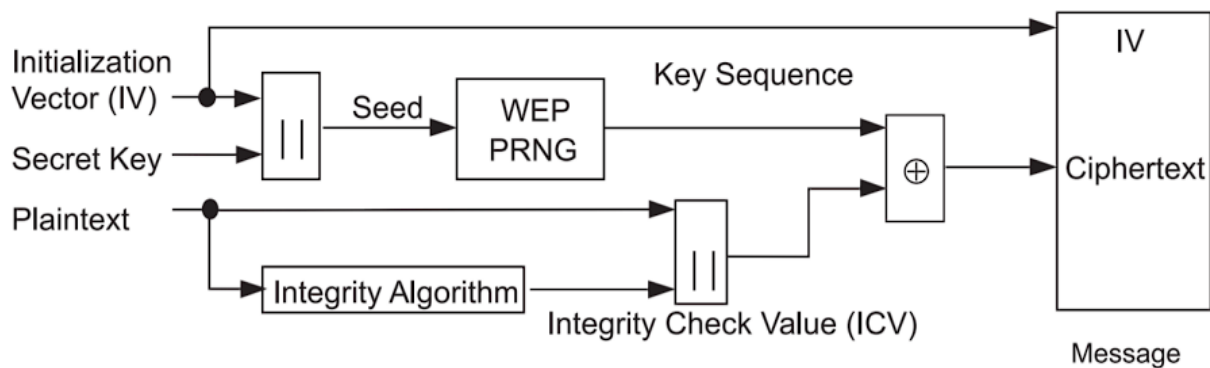
Figura 2-31. Proceso del cifrado WEP [71]
