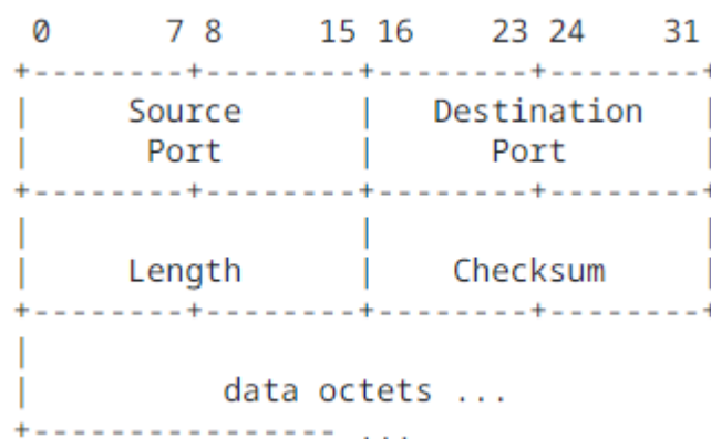
Figura 2-23. Formato de la cabecera UDP
