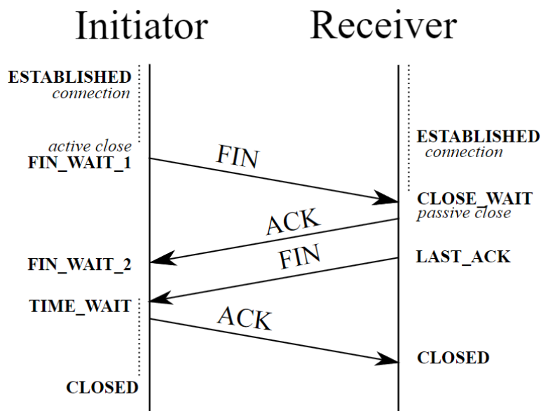
Figura 2-20. Diagrama de paso de mensajes y estados de los nodos al finalizar una conexión [31]
