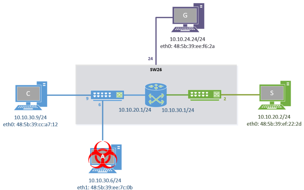
Figura 3-16. Escenario ataque redirección
