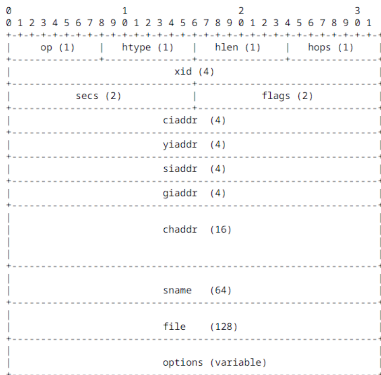
Figura 2-29. Formato de la cabecera DHCP
