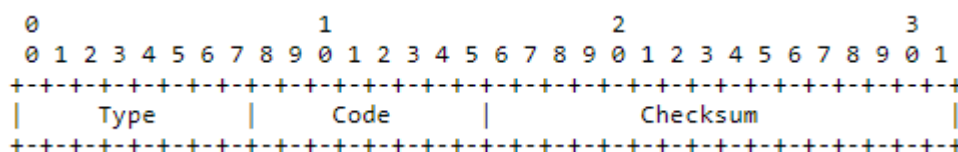
Figura 2-16. Fragmento común de la cabecera ICMPv4
