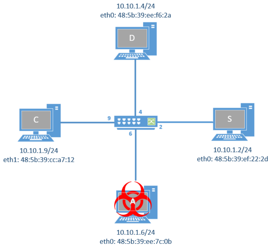
Figura 3-32. Escenario ataque secuestro/redireccionamiento DNS
