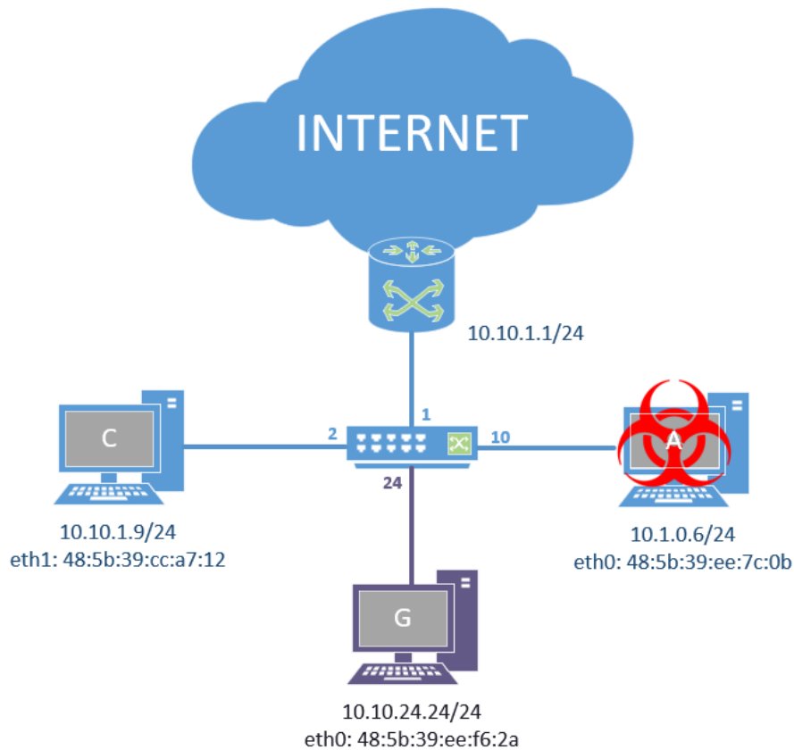
Figura 3-30. Escenario ataque amplificación/reflexión DNS
