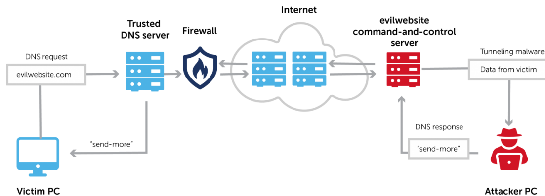
Figura 2-28. Ejemplo de tunelización DNS [53]
