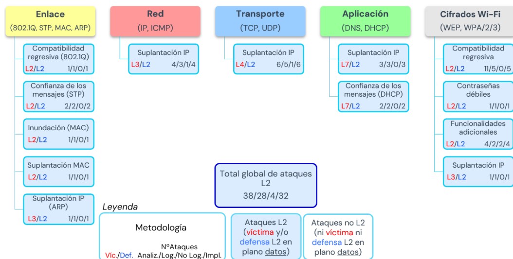
Figura 6-5. Esquema de las metodologías de los ataques L2 implementados en el proyecto
