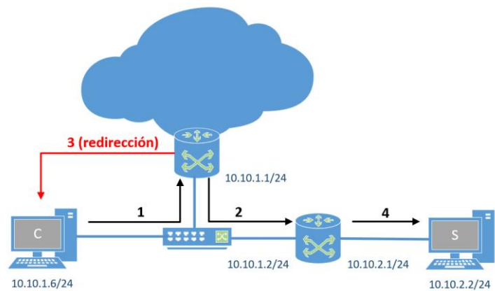
Figura 2-17. Envío de un mensaje ICMP de redirección
