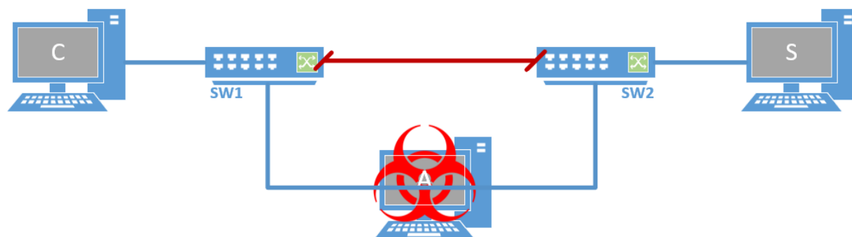
Figura 3-9. Esquema de la VLAN 1 tras el ataque 0
