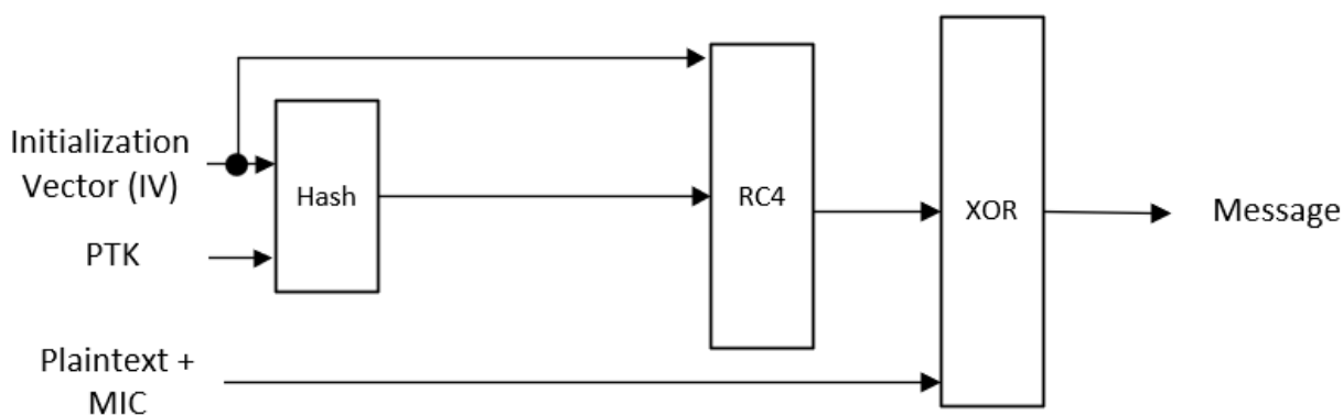
Figura 2-34. Proceso simplificado del cifrado WPA TKIP [73]
