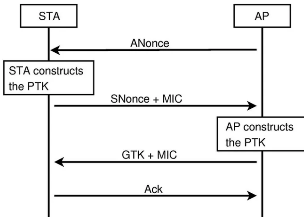
Figura 2-35. 4-way handshake entre cliente (STA) y punto de acceso [75]
