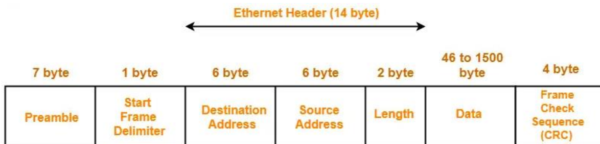
Figura 2-2. Ubicación de las direcciones MAC en una trama Ethernet
