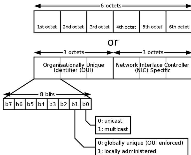
Figura 2-1. Formato de las direcciones EUI-48 [8]
