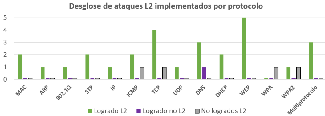
Figura 6-4. Ataques objetos de estudio logrados y no logrados por protocolo
