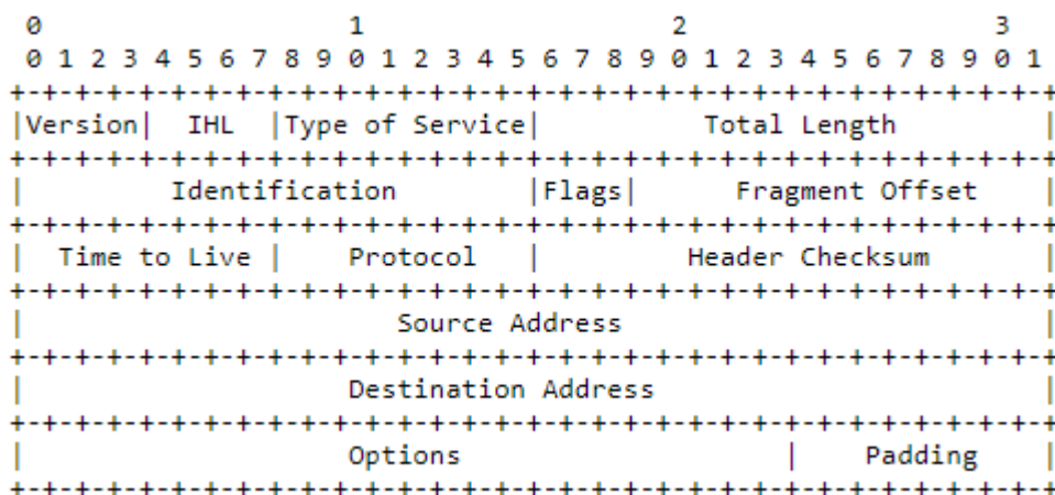
Figura 2-15. Esquema ASCII de la cabecera IPv4
