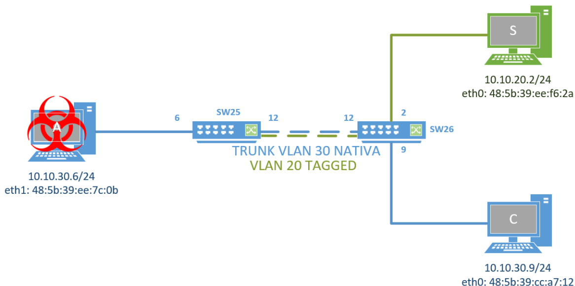
Figura 3-3. Escenario del ataque 7.2.1
