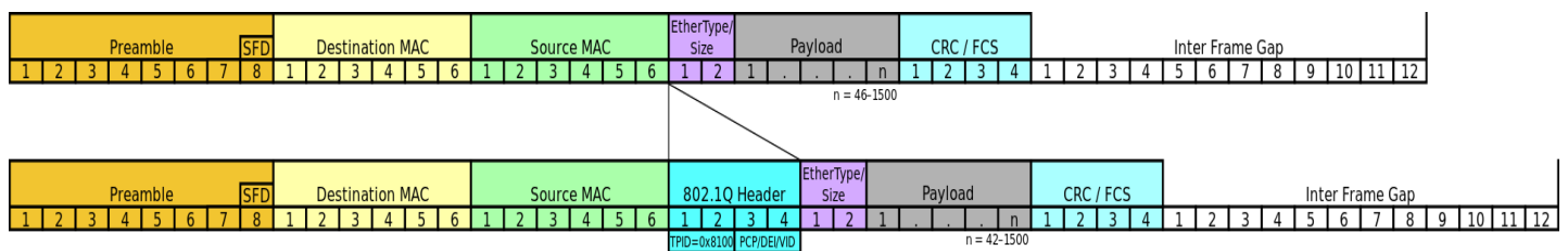
Figura 2-7. Inserción de la etiqueta VLAN en una trama Ethernet [11]
