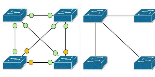
Figura 2-11. Red de puentes antes y después de ejecutar STP [13]
