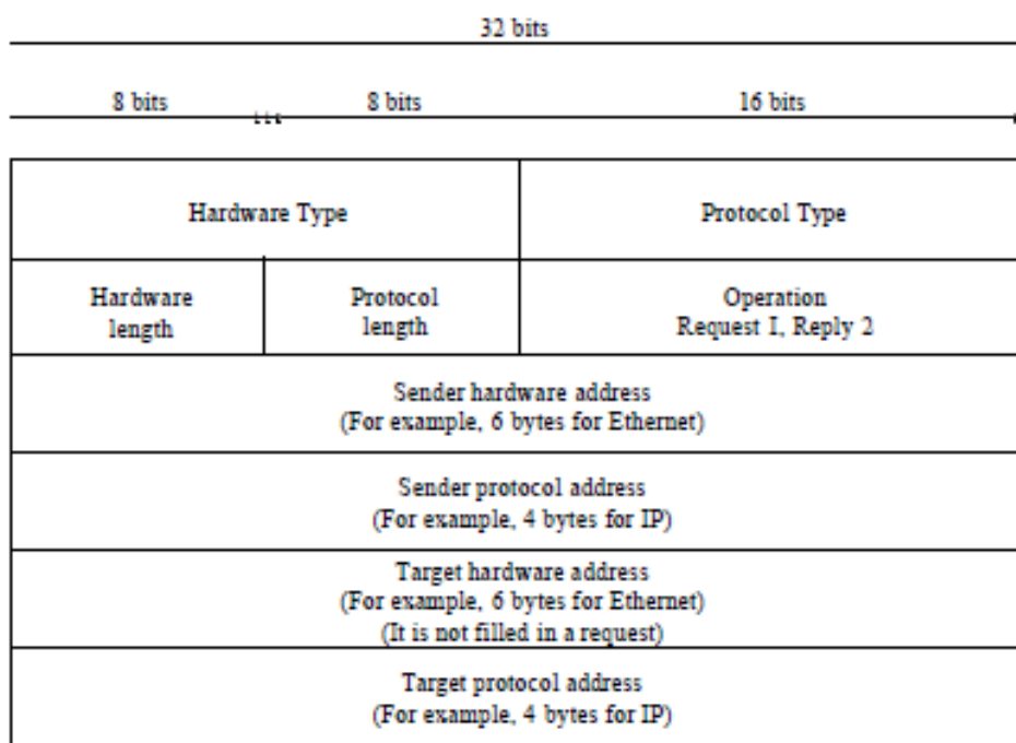
Figura 2-5. Formato de la cabecera del protocolo ARP [10]
