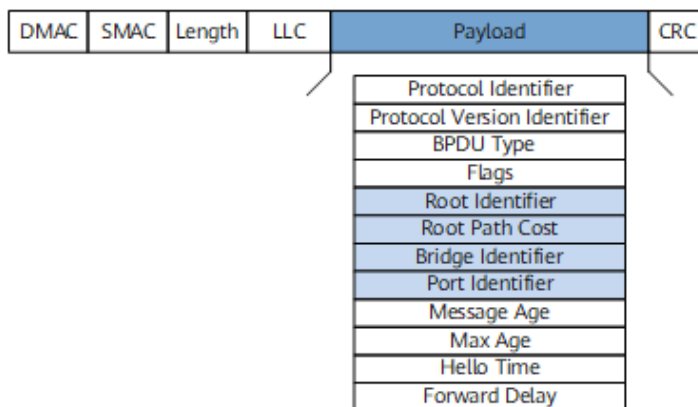
Figura 2-12. Estructura de una BPDU
