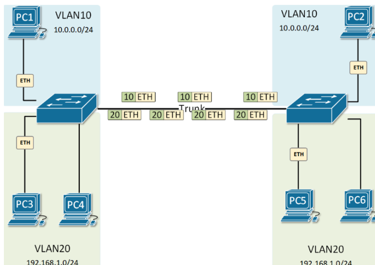
Figura 2-8. Escenario con dos VLANs y trunk entre conmutadores
