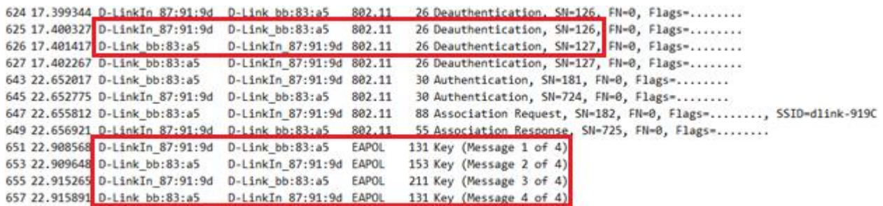
Figura E-36. Deautenticación del cliente y handshake capturado por parte del atacante
