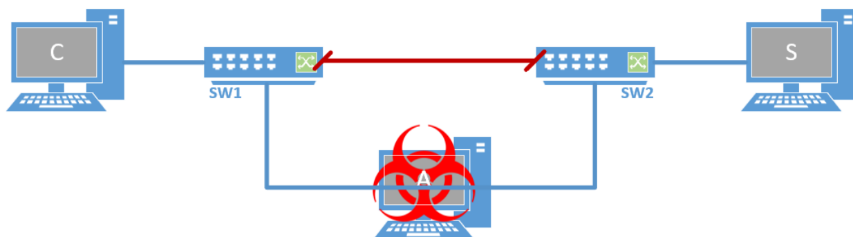
Figura 2-13. Atacante modificando la topología de la red tras suplantar el puente raíz
