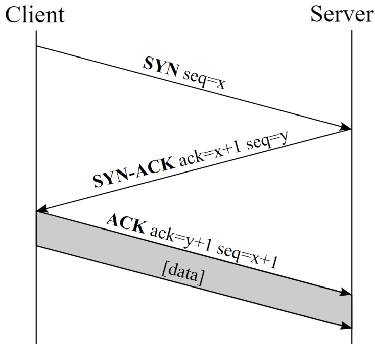
Figura 2-19. Diagrama de paso de mensajes del Triple-way handshake entre cliente y servidor [30]
