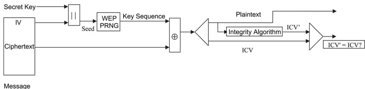
Figura 2-32. Proceso del descifrado WEP y verificación del mensaje
