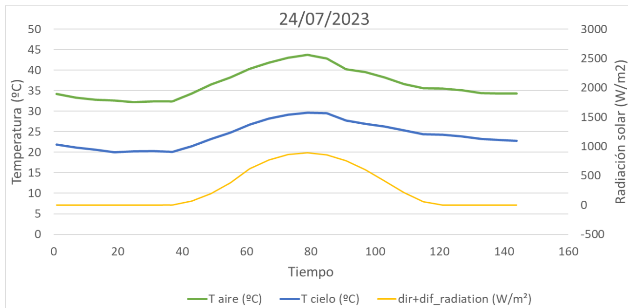
Figura 14: Radiación solar del 24/07/2023
