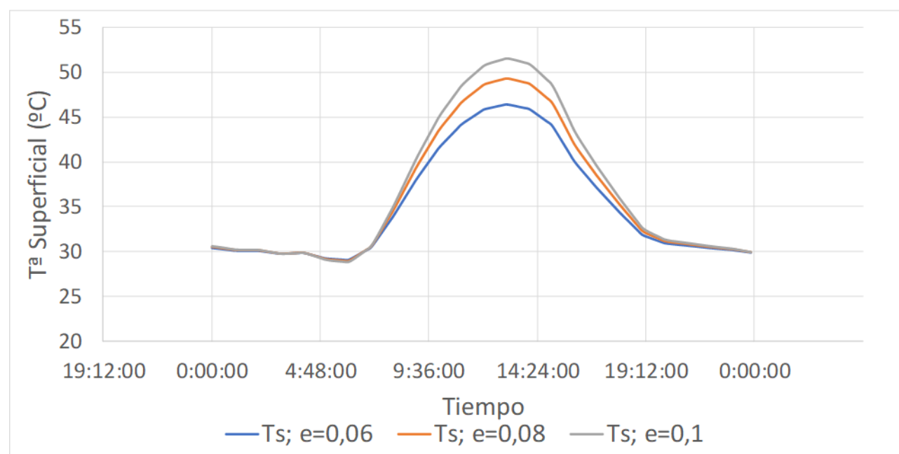
Figura 22: Influencia del espesor
