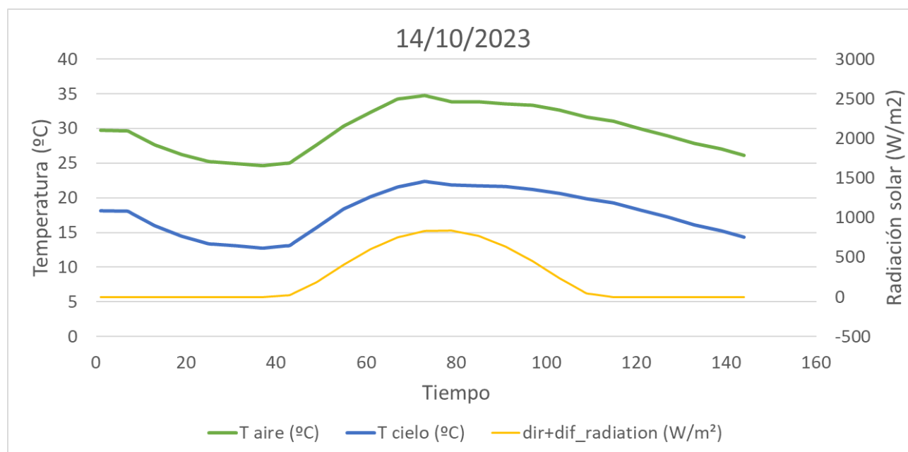
Figura 15: Radiación solar del 14/10/2023. Fuente: Elaboración propia
