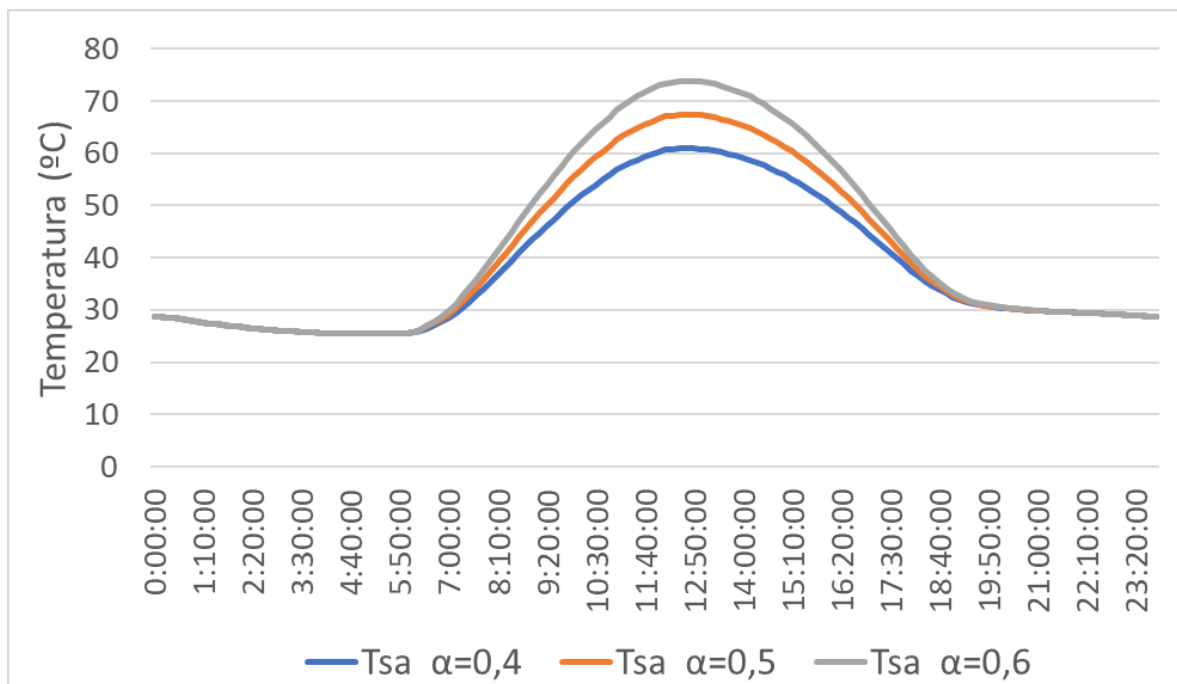
Figura 16: Influencia de la absortividad para un espesor dado. Fuente: Elaboración propia
