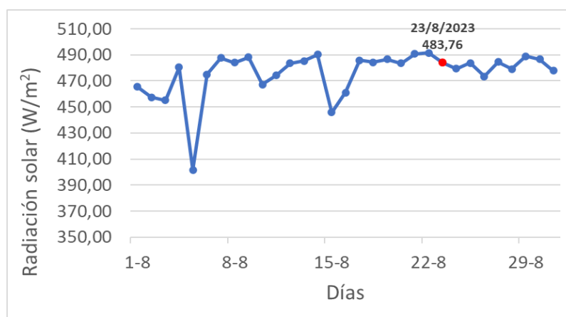
Figura 32: Día tipo de agosto. Fuente: Elaboración propia
