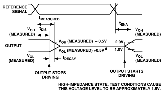
Figure 27. Output Enable/Disable
