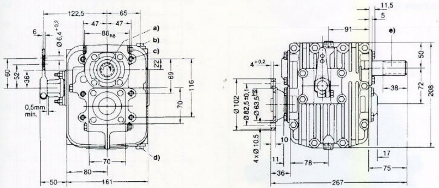
Fig. 6 HBW 125
