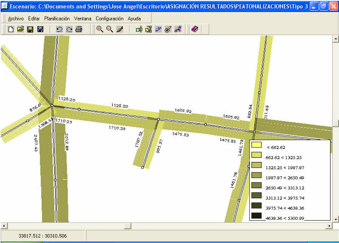
Fig.17.57.Av. Cruz del Campo. Peatonalización tipo 3
