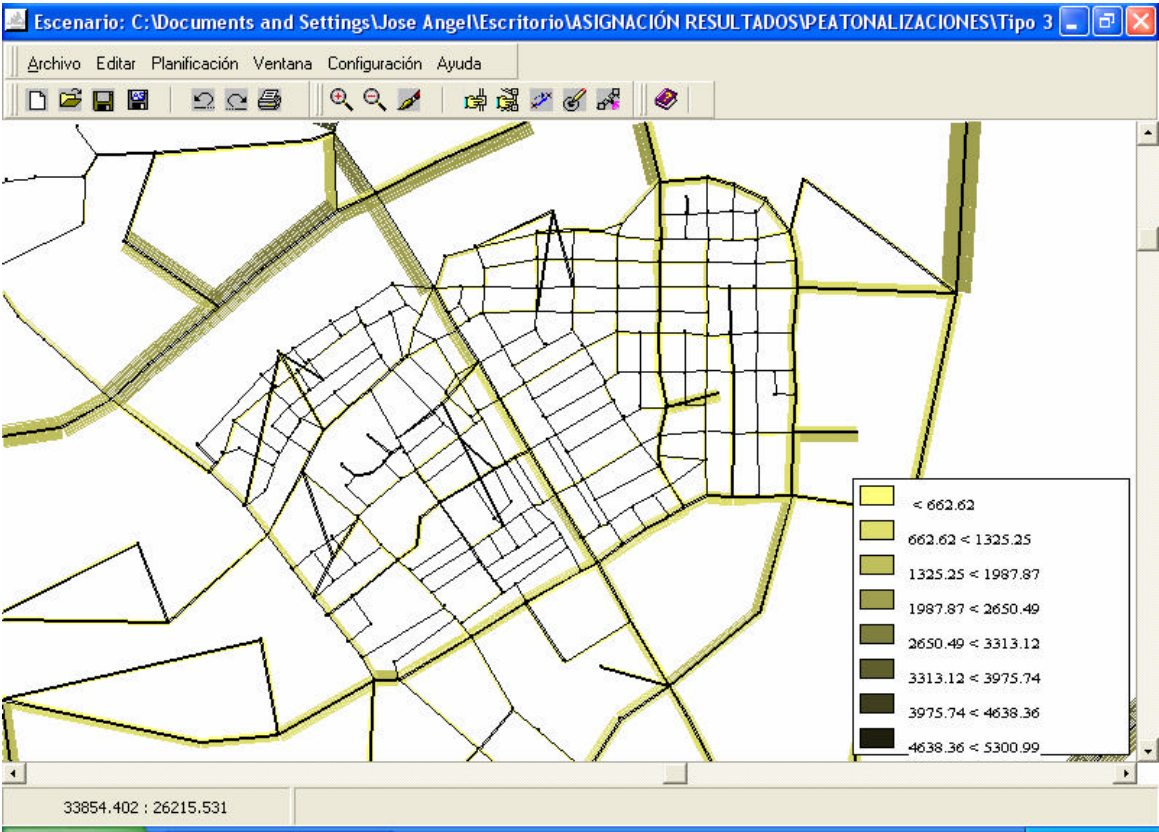
Fig.17.41. Los Remedios y Santa Cecilia. Plano General. Peatonalización tipo 3
