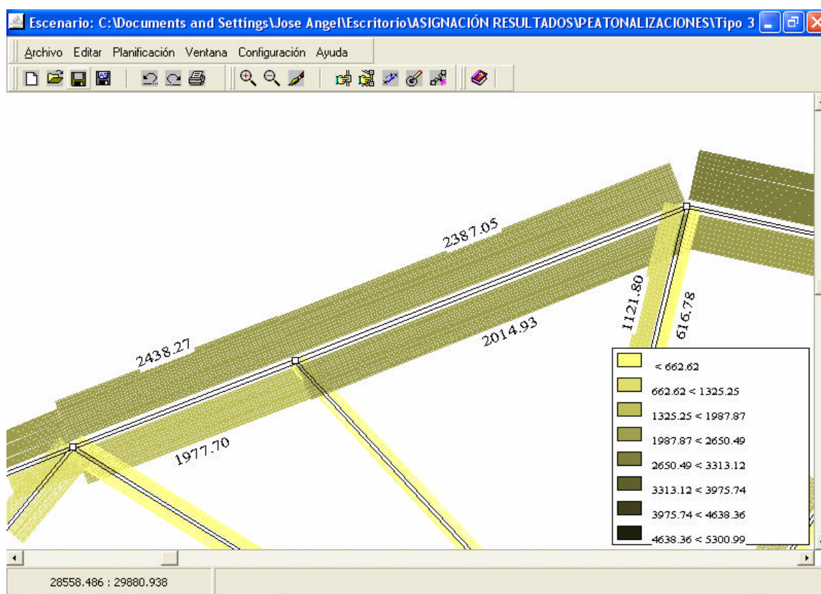
Fig.17.56.Alcalde Manuel del Valle. Peatonalización tipo 3
