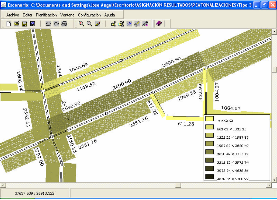
Fig.17.54.Av. La palmera. Peatonalizaci3n tipo 3
