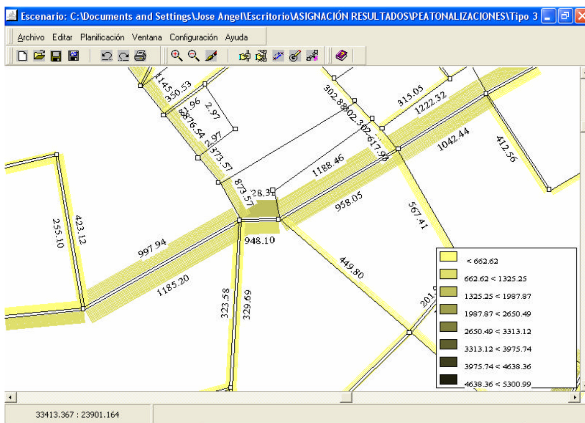
Fig.17.48. Los Remedios y Santa Cecilia. Zona 7 Peatonalización tipo 3.
