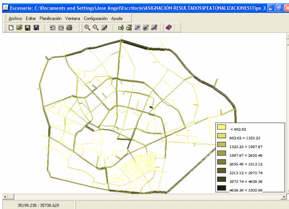
Fig.17.50.Plano general. Peatonalización tipo 3
