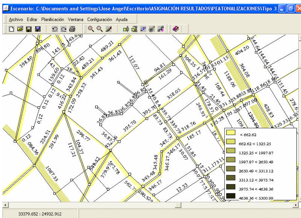
Fig.17.47. Los Remedios y Santa Cecilia. Zona 6 Peatonalización tipo 3.
