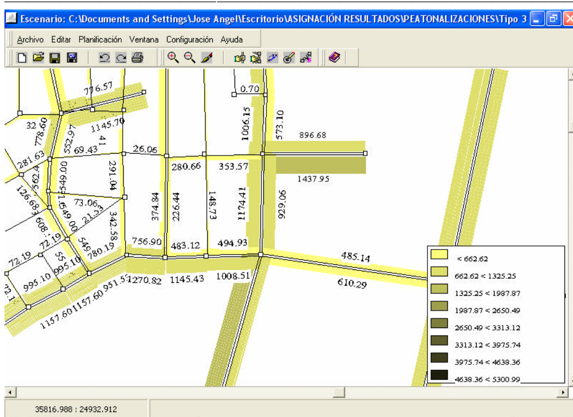
Fig.17.43. Los Remedios y Santa Cecilia. Zona 2. Peatonalización tipo 3.
