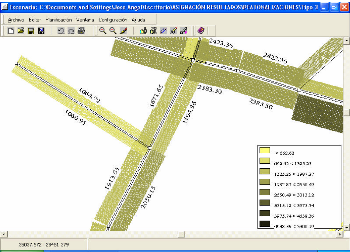
Fig.17.53.Ram3n y Cajal. Peatonalizaci3n tipo 3
