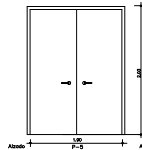
Puerta abatible dos hojas cristal
