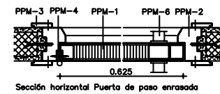
Sección horizontal Puerta de paso enrasada
