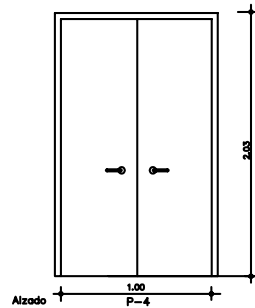
Puerta abatible dos hojas madera
