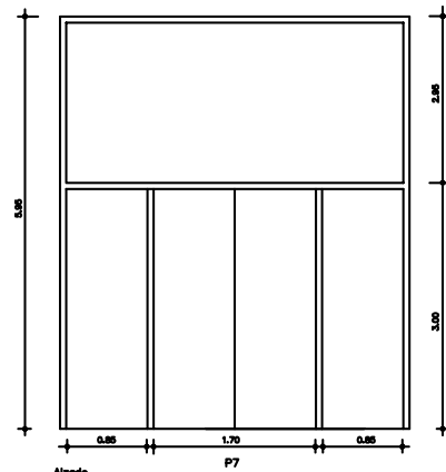
Puerta abatible cristal
