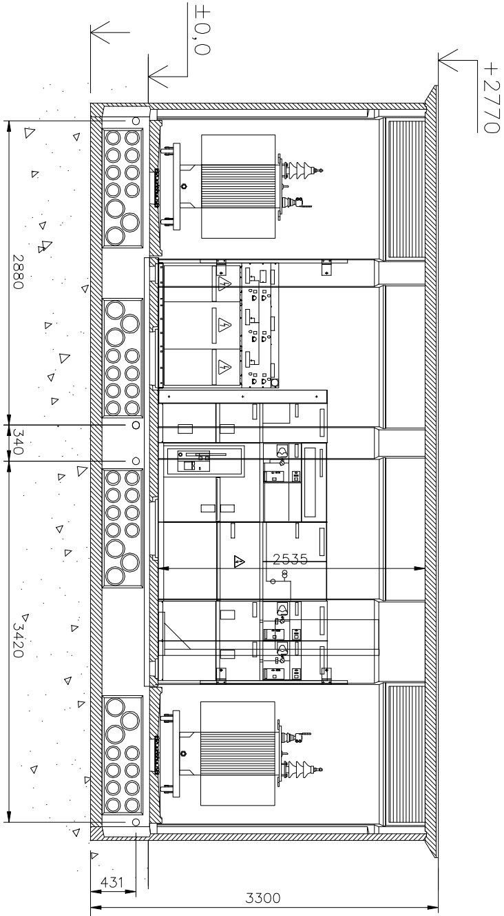
SECCIÓN
